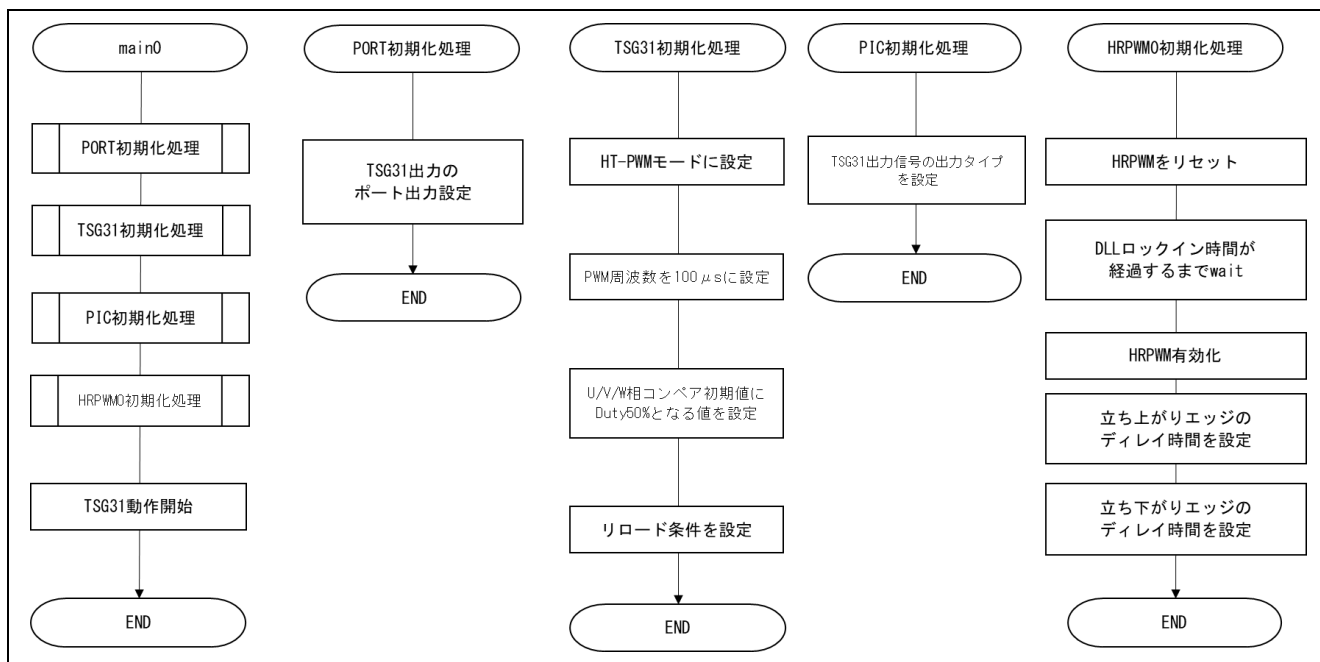
図 2-2 PWM 出力ディレイ動作フロー
