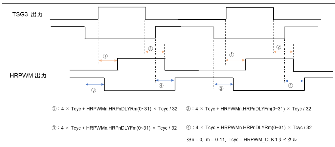
図 2-1 PWM 出力ディレイ動作概要
