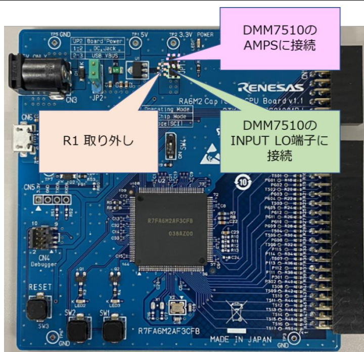
図 5-2 RA6M2 Cap Touch CPU ボード・前面
