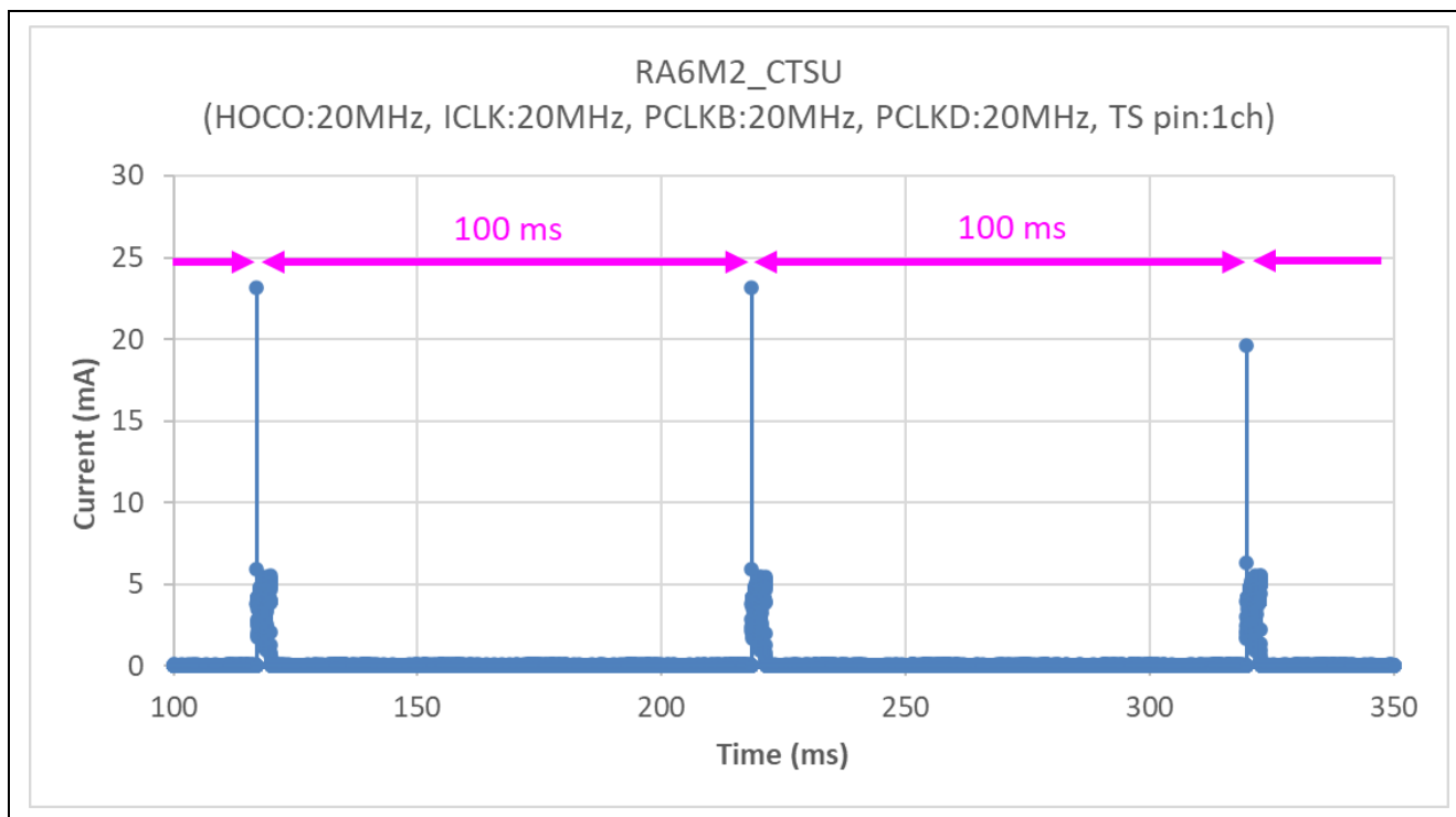
図 5-5 消費電流波形 TS 端子 1ch 計測 (1/2)
