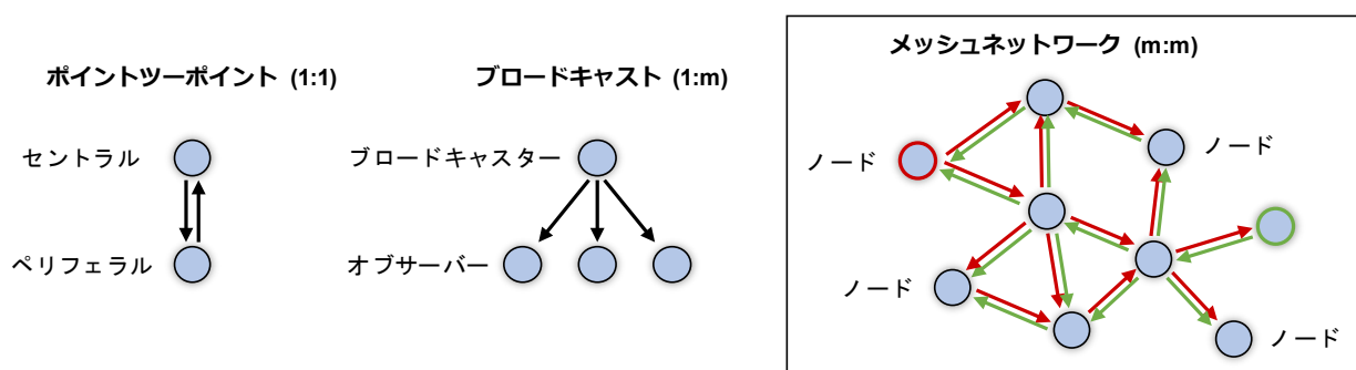
図 1-1 通信トポロジー
