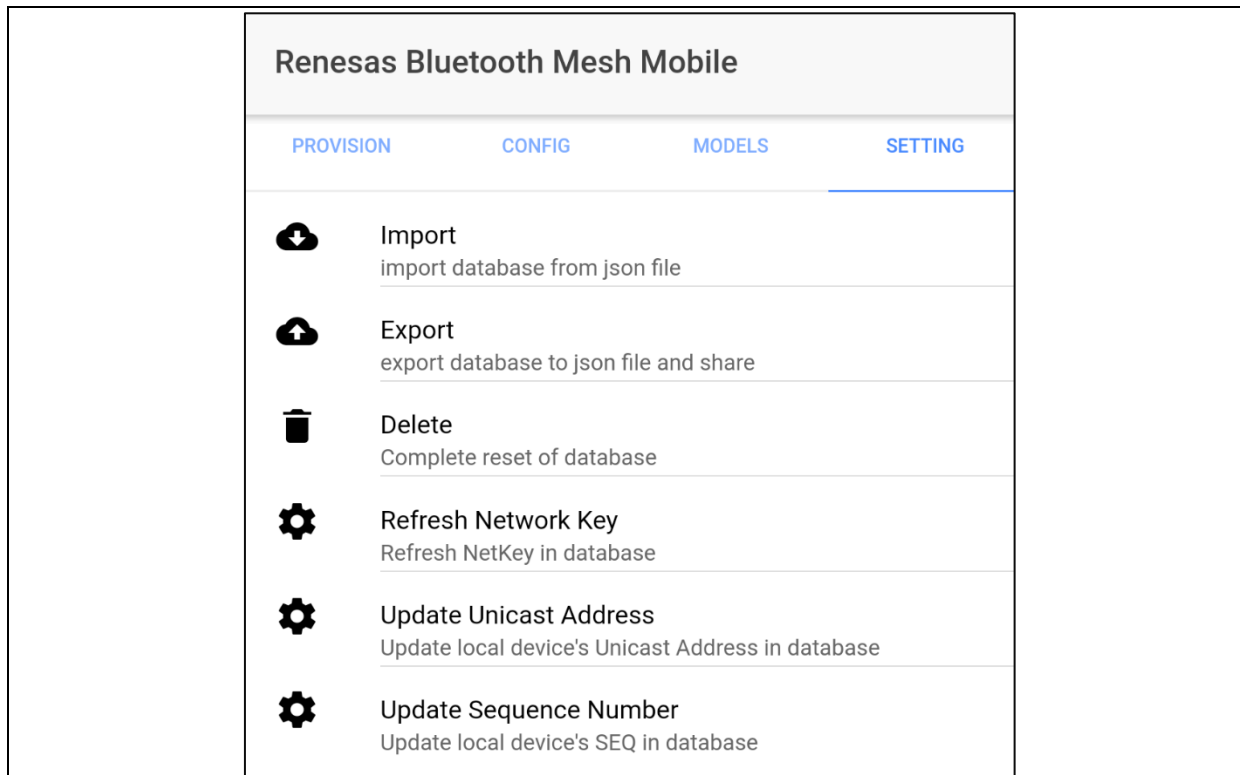
図 6-2 SETTING タブ
