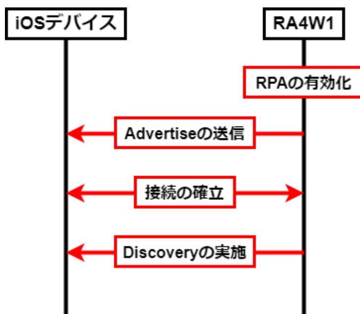
図 1.2 接続時の動作フロー
