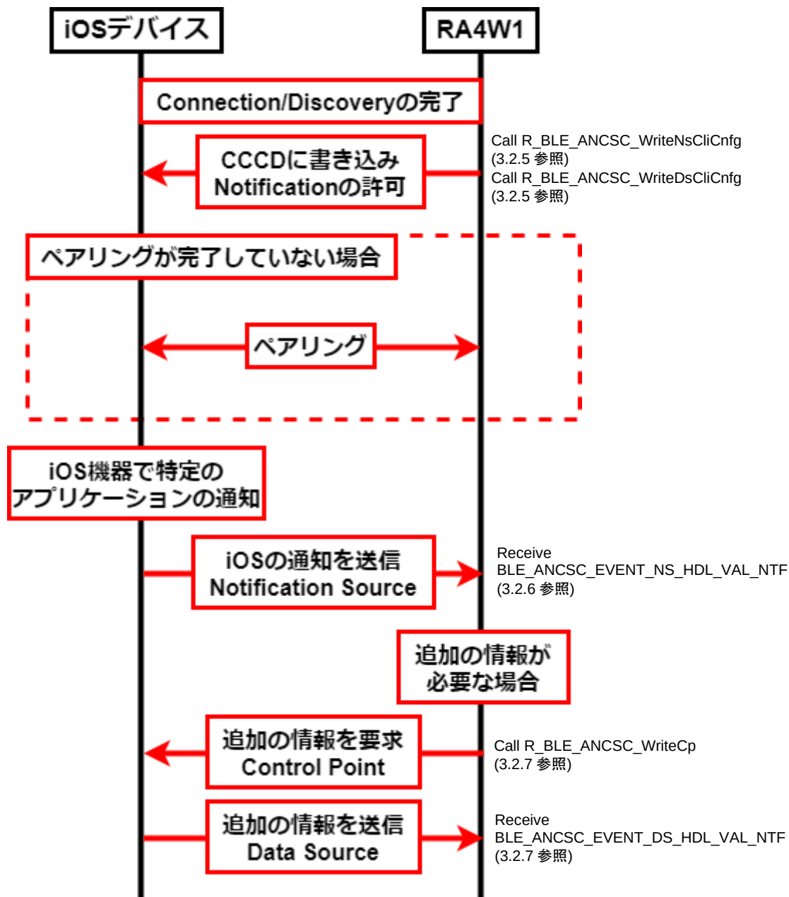
図 1.3 ANCS の動作フロー
