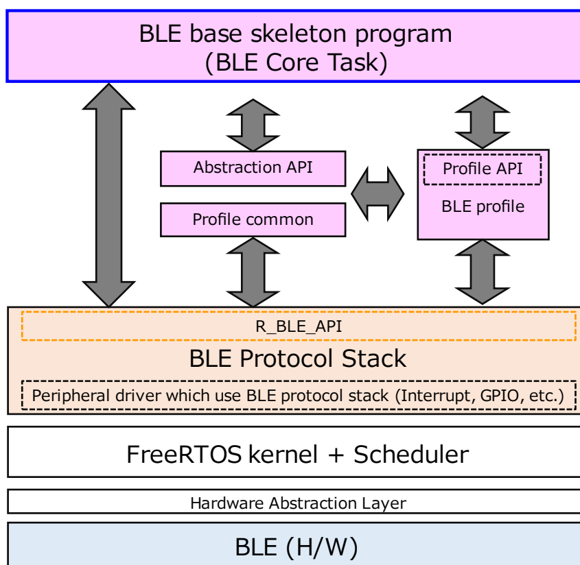
図 3.1 FreeRTOS 版プロジェクトの構成
