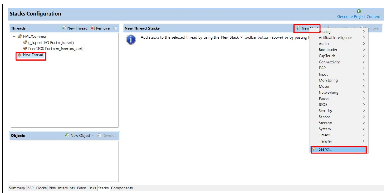
図 25 AWS Core MQTT モジュールの選択
