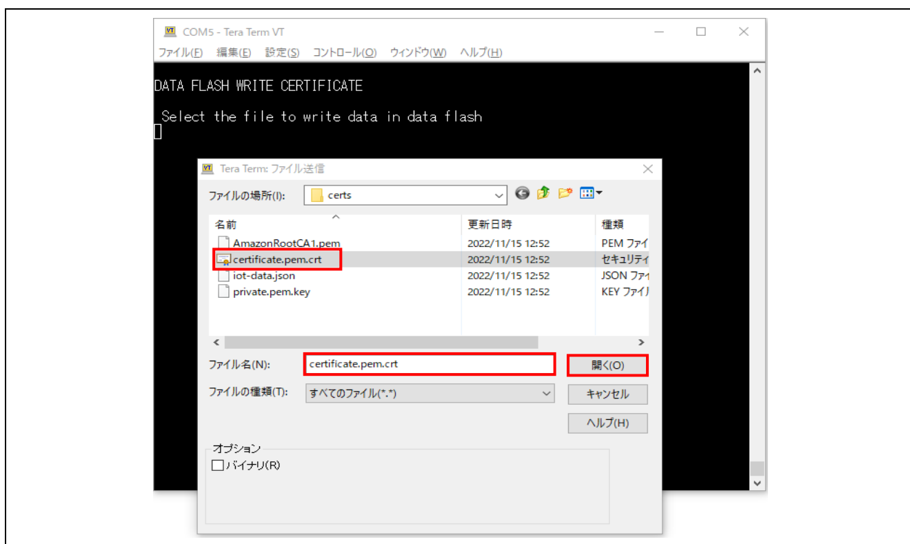
図 14 データフラッシュへのデバイス証明書のダウンロード
