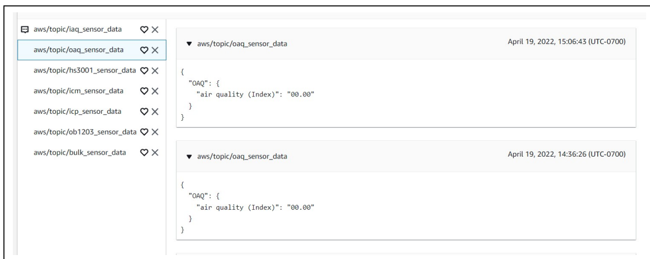
図 21 AWS IoT 画面でのサブスクライブされたメッセージ
