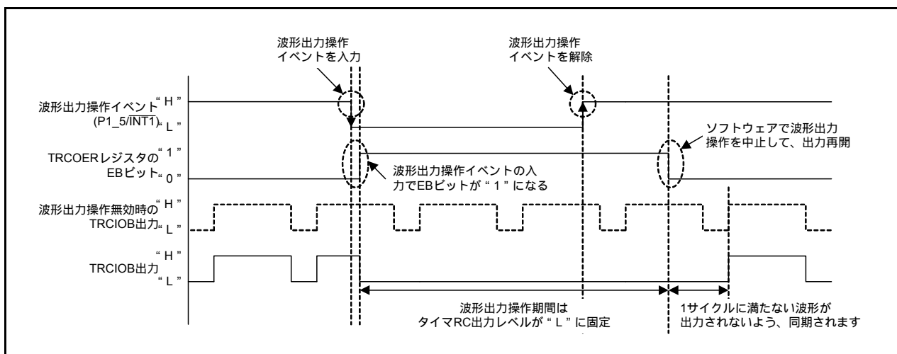
図 1.2 リスタート方式がソフトウェアで出力再開の場合の動作例
