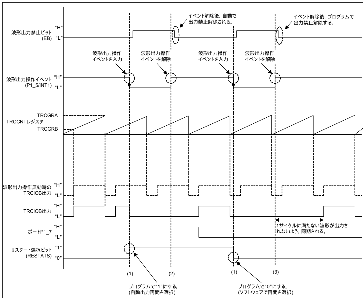
図 4.1 タイミング図
