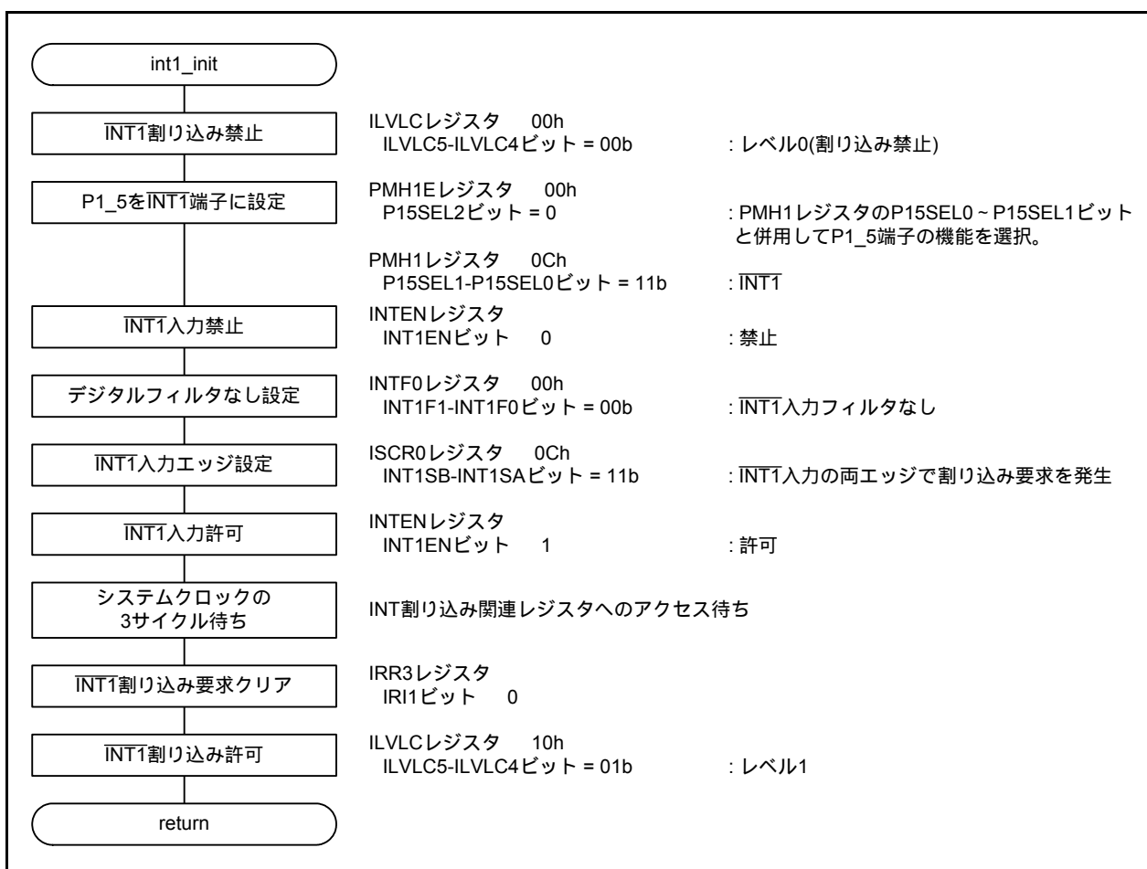
図 4.4 INT1 割り込み設定処理
