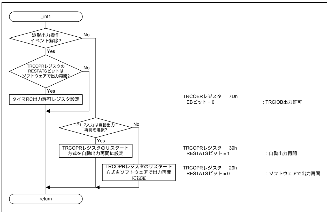
図 4.6 INT1 割り込み処理
