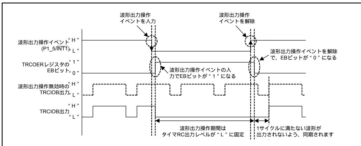
図 1.1 リスタート方式が自動出力再開の場合の動作例
