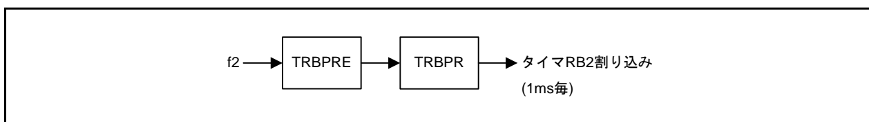
図 3.1 ブロック図
