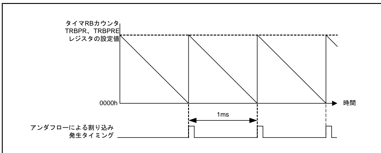
図 3.2 タイミング図
