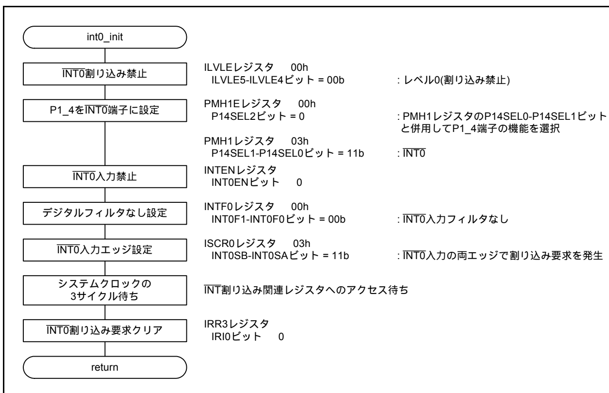
図 4.4 INT0 割り込み設定処理
