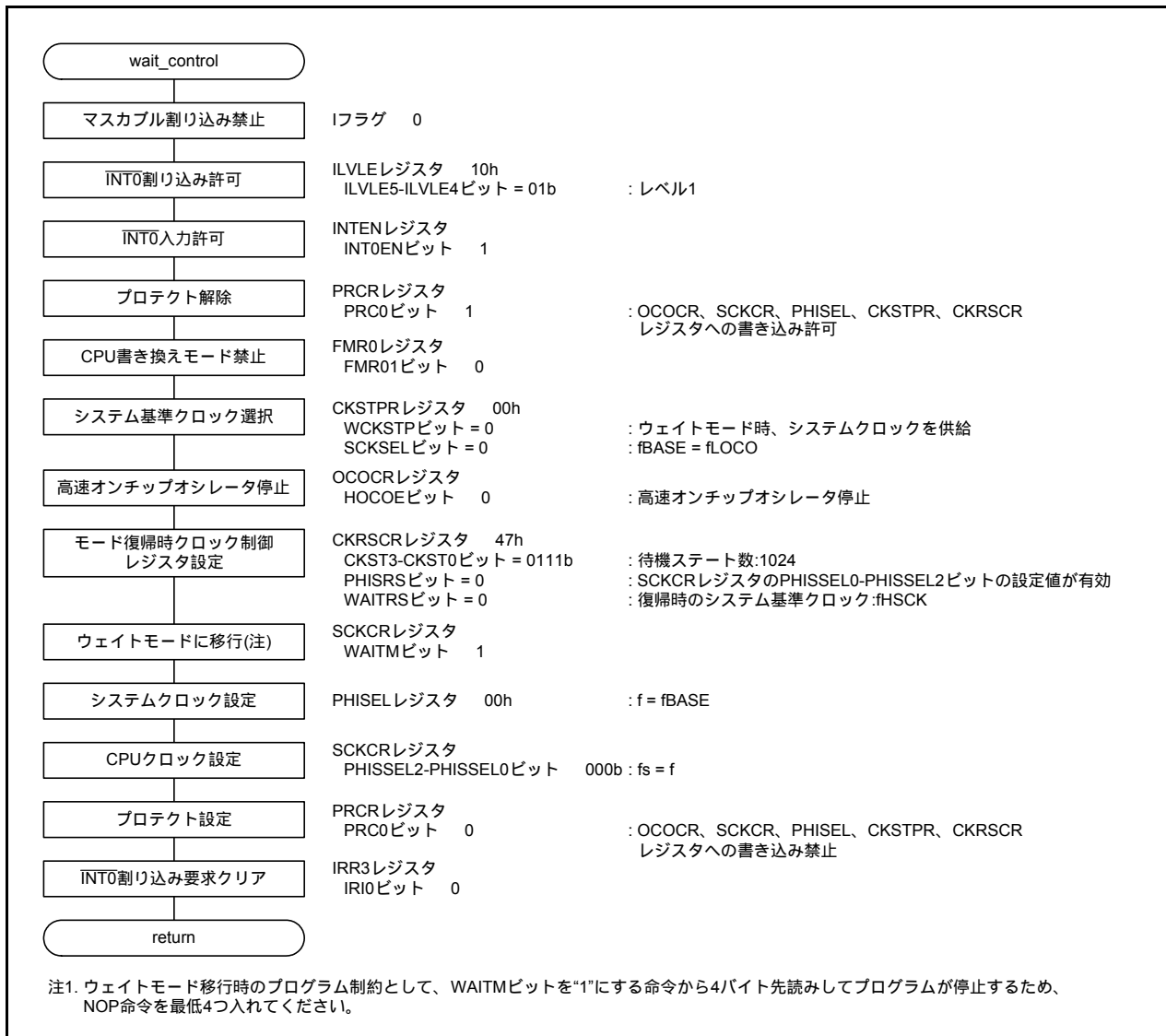
図 4.5 ウェイトモード処理
