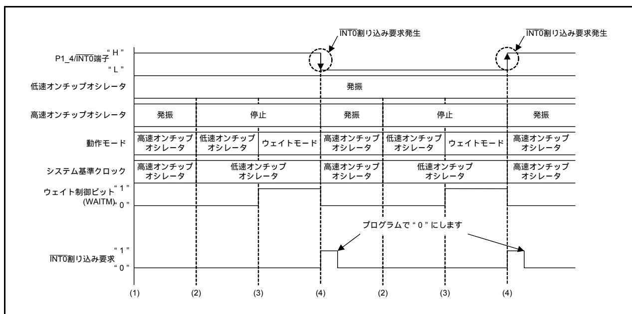
図 4.1 タイミング図
