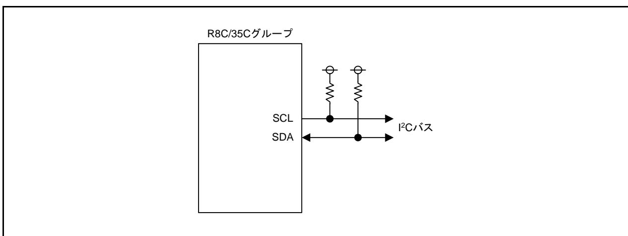
図 3.2 ブロック図
