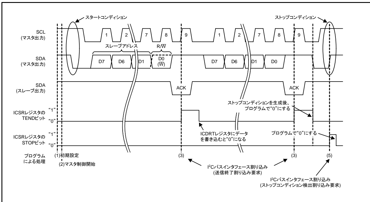
図 3.4 マスタ送信のタイミング図
