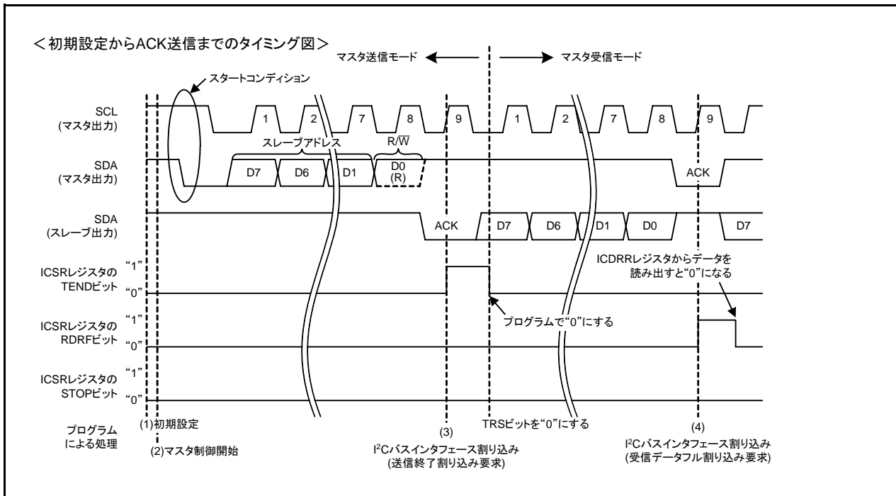
図 3.5 マスタ受信のタイミング図(1)
