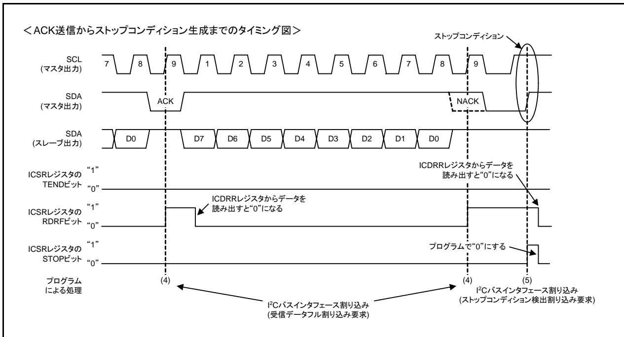
図 3.6 マスタ受信のタイミング図(2)
