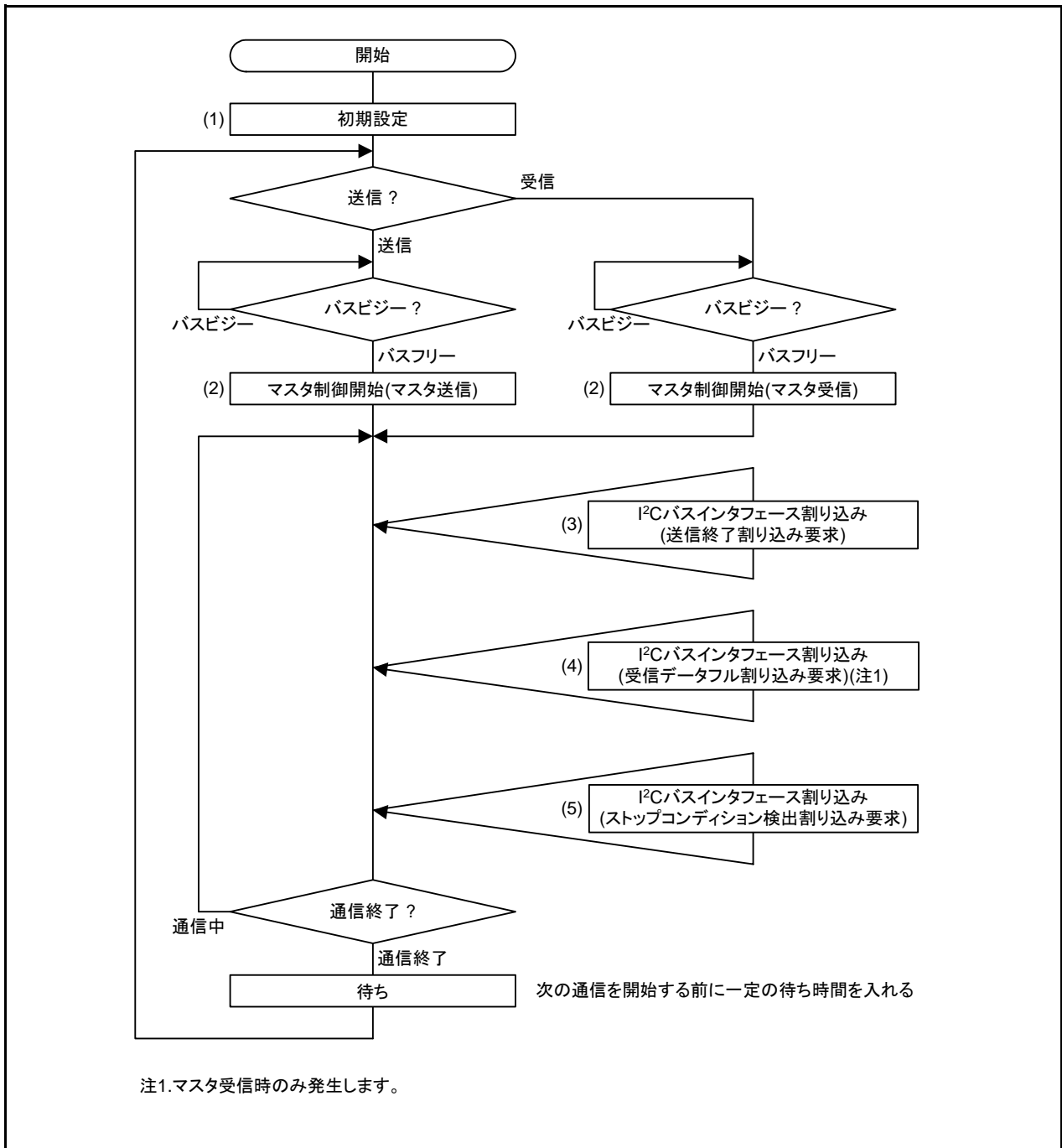
図 3.3 概略フローチャート
