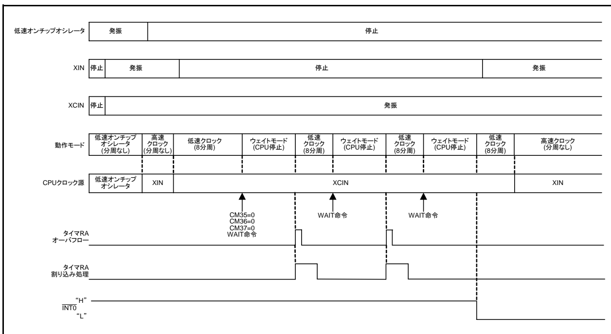
図 3.1 ウェイトモード動作例
