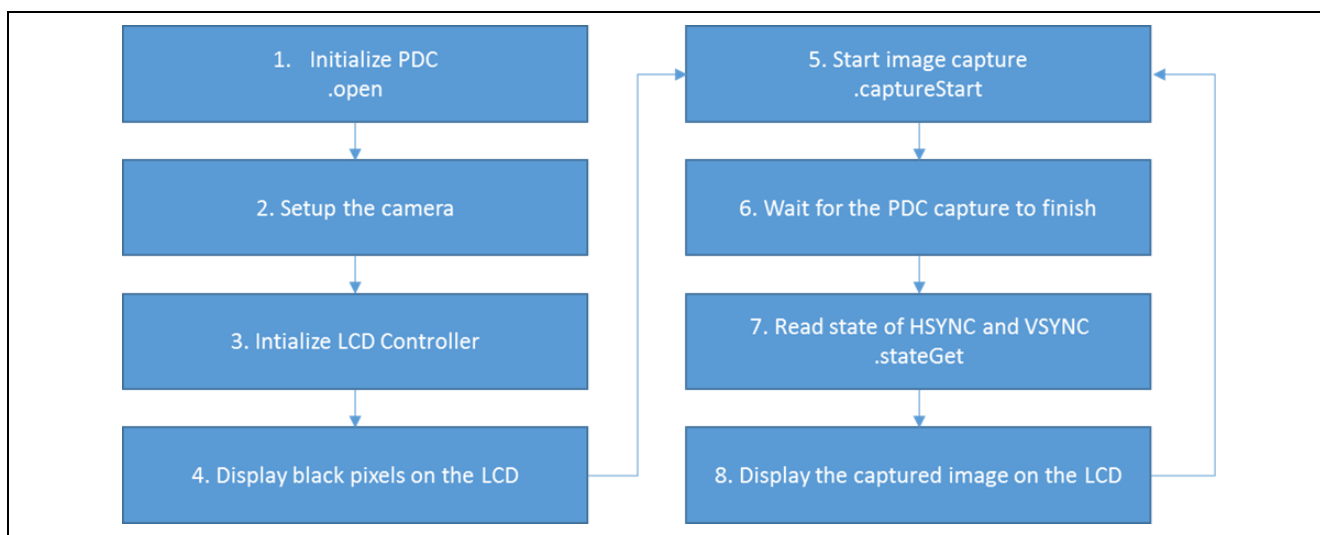
図 1 PDC HAL モジュールのアプリケーションプロジェクトのフロー
