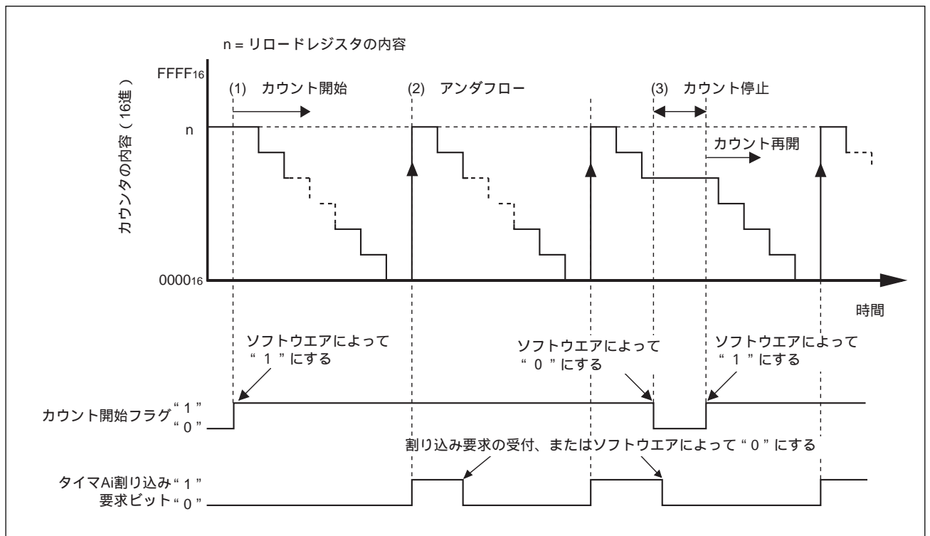
図1 タイマモード動作タイミング
