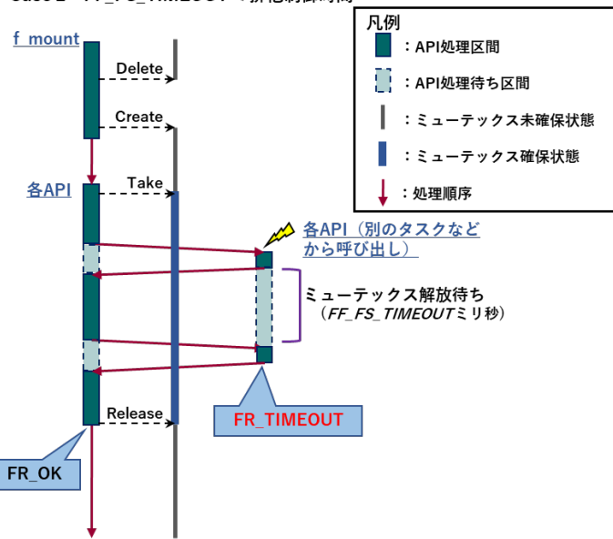
図 1.2 ボリュームに対する排他制御
