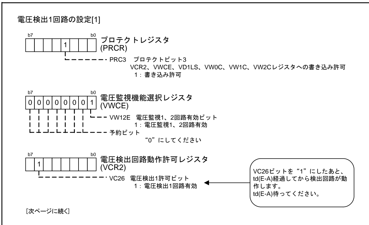
図 5.3 電圧監視1回路に関するレジスタ設定(1/2)
