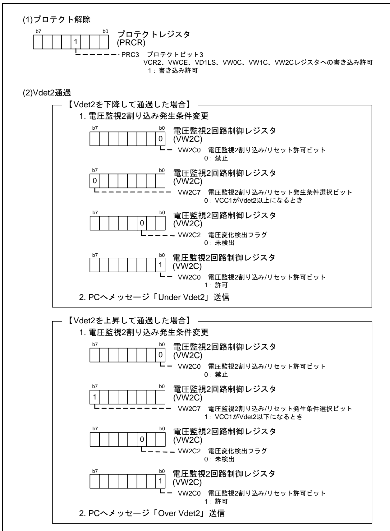
図 5.6 割り込み処理とレジスタ設定 (1/2)
