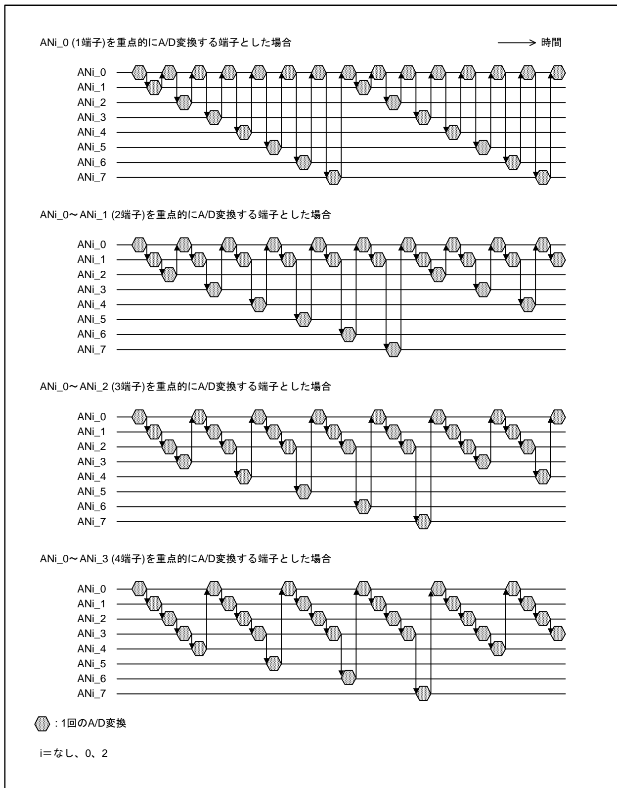
図 3.1 繰り返し掃引モード1でA/D変換する端子の遷移図
