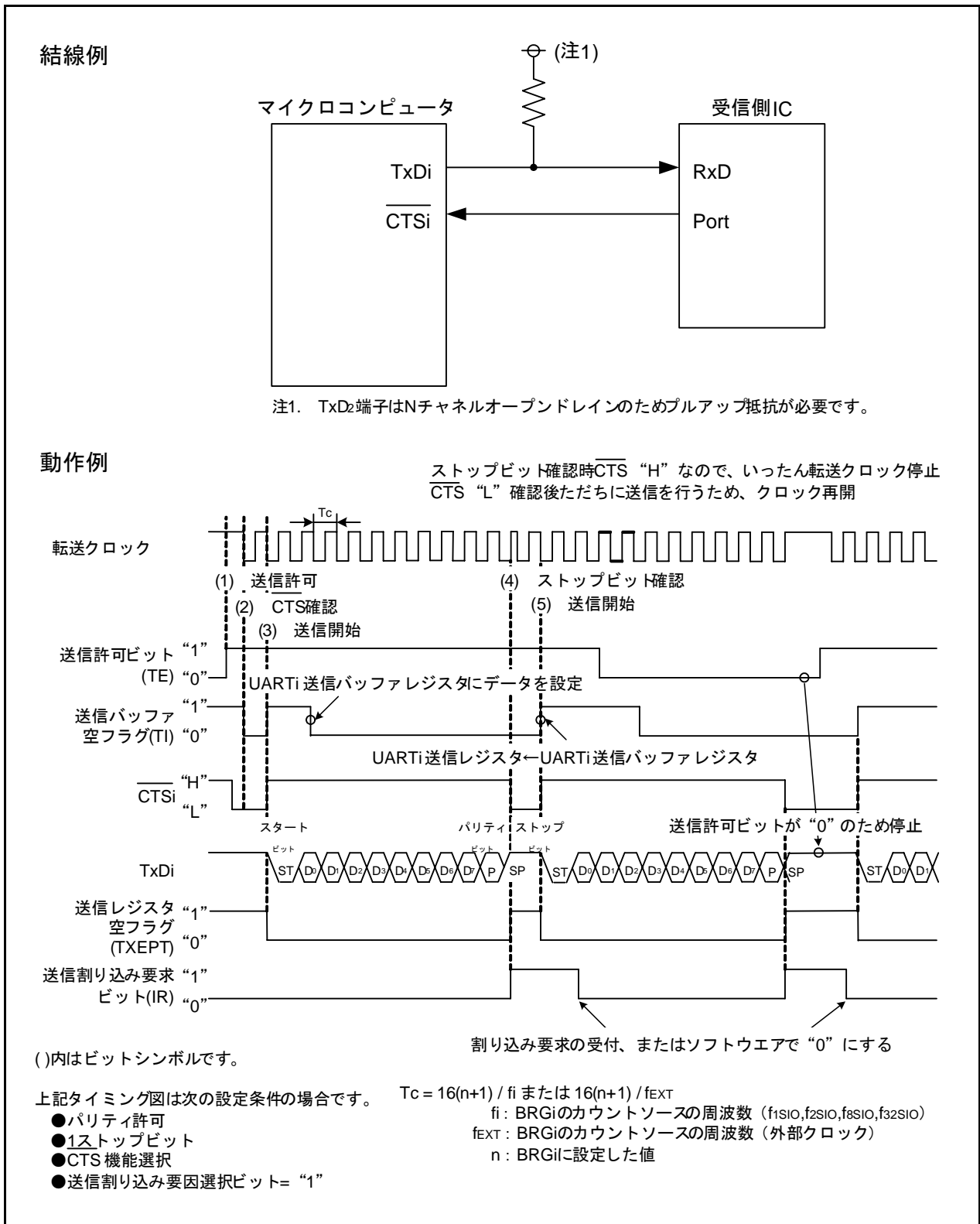
図 4.1 クロック非同期形シリアルI/Oモードの送信動作タイミング
