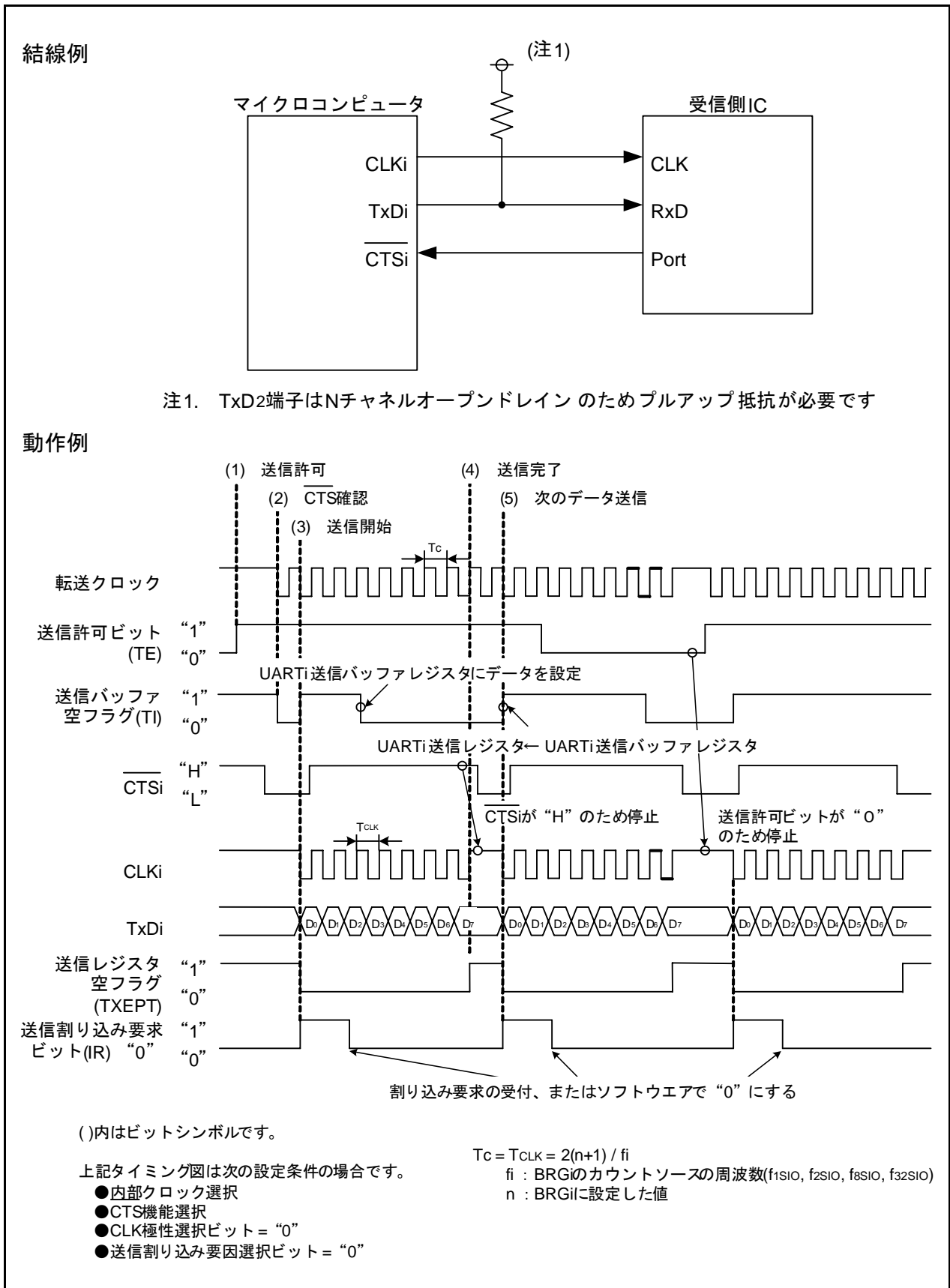
図 4.1 クロック同期形シリアルI/Oモードの送信動作タイミング
