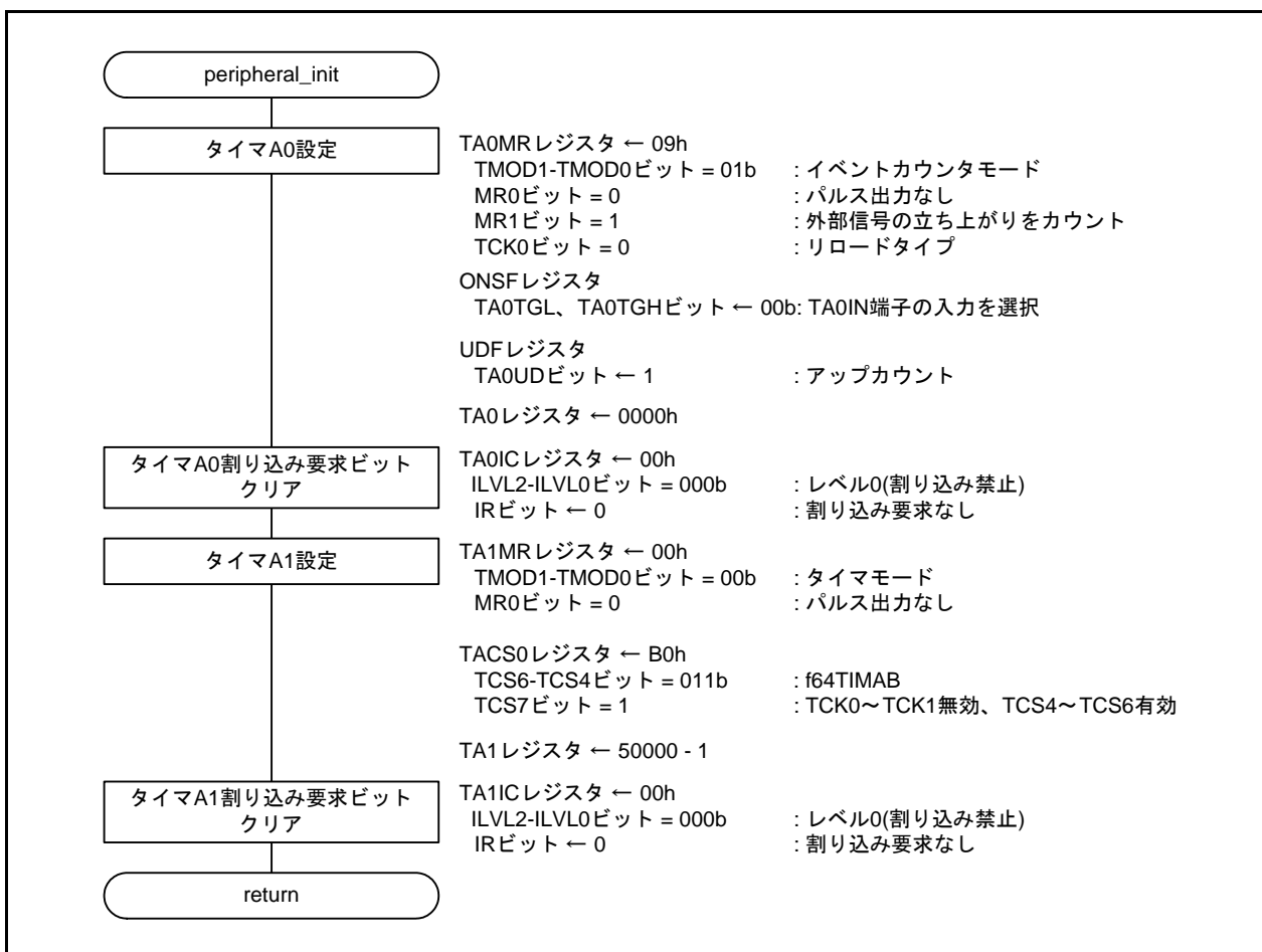
図 4.3 周辺機能初期設定処理
