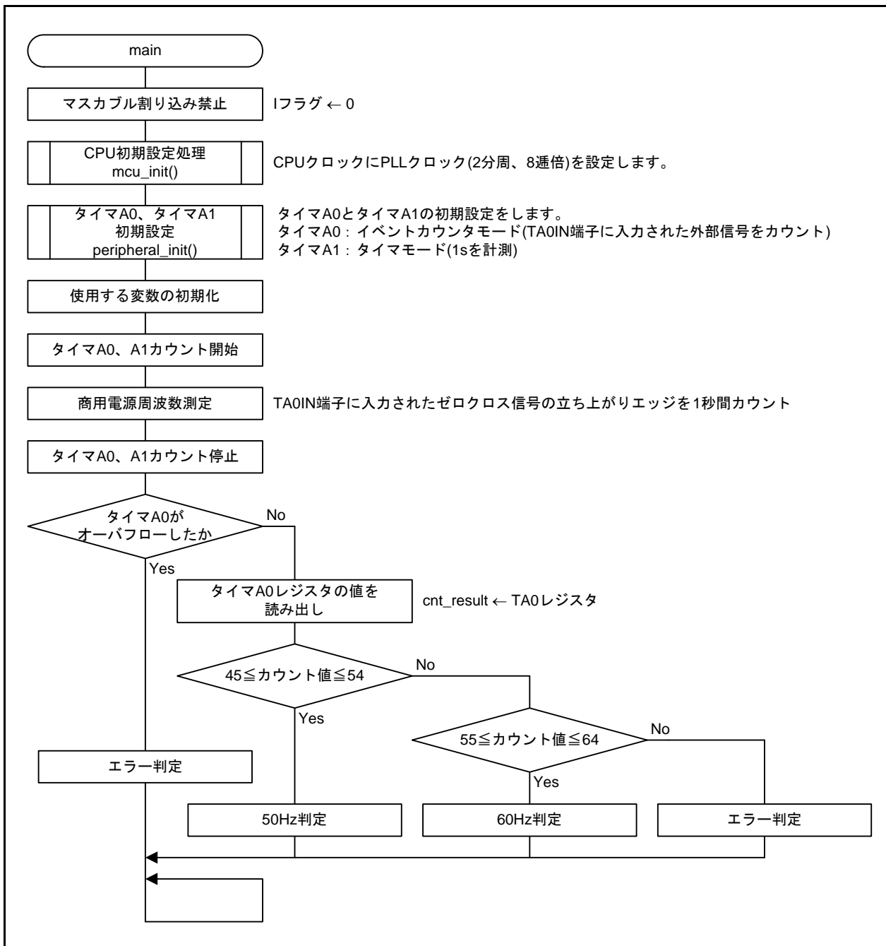
図 4.2 メイン処理
