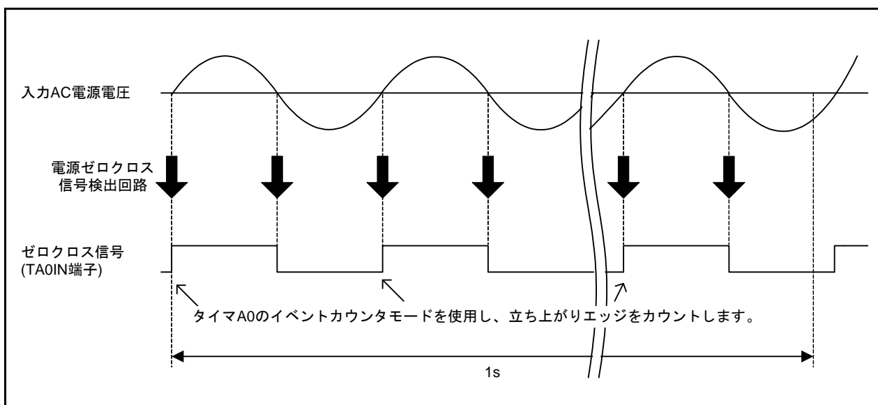
図 1.2 AC電源電圧ゼロクロス信号の検出
