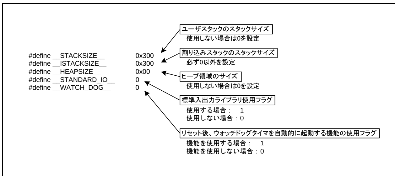
図 4.2 cstartdef.h
