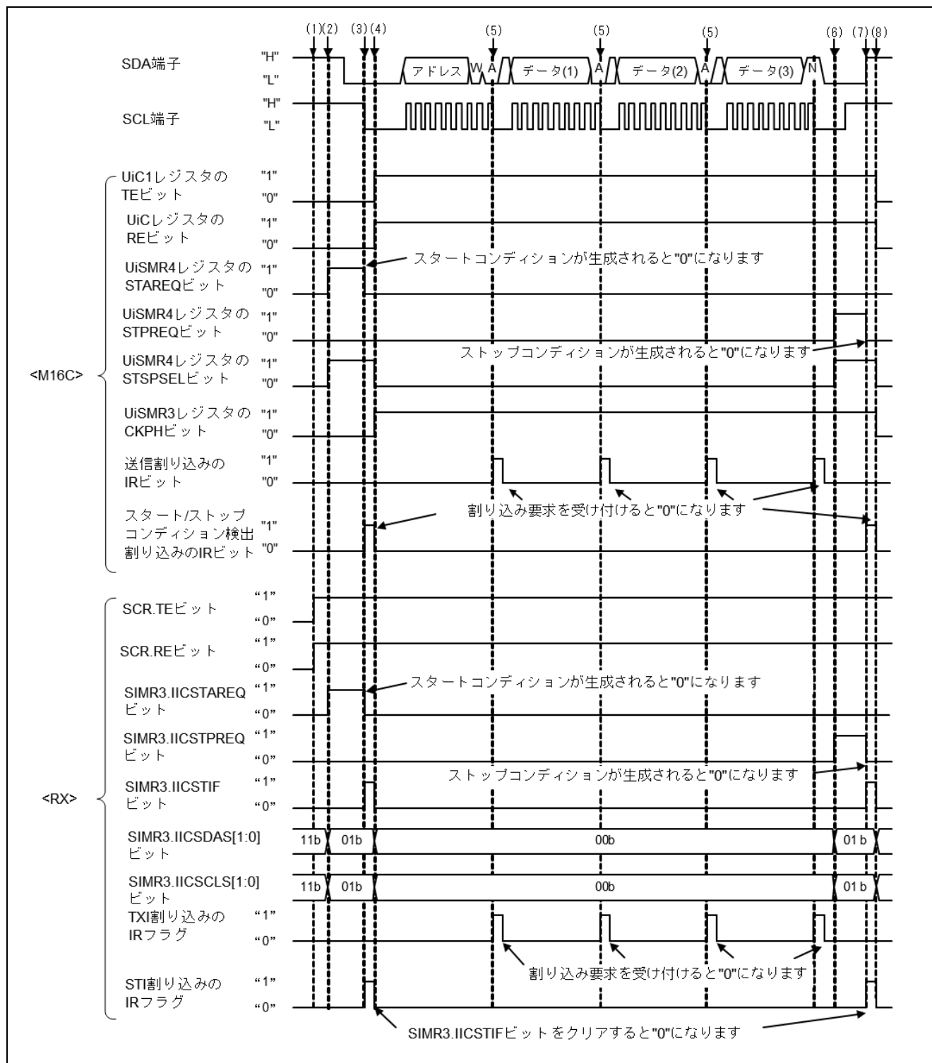
図 3.1 RX と M16C のマスタ送信タイミング相違点(3 バイトずつ送信する場合)
