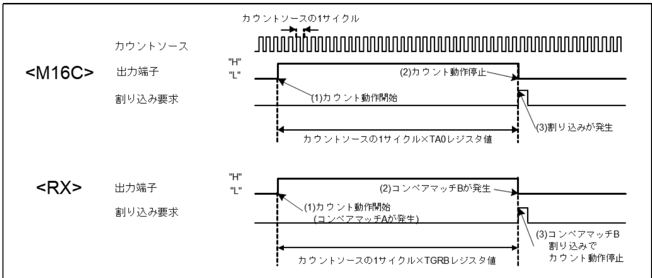
図 1.2 ワンショットパルス出力例
