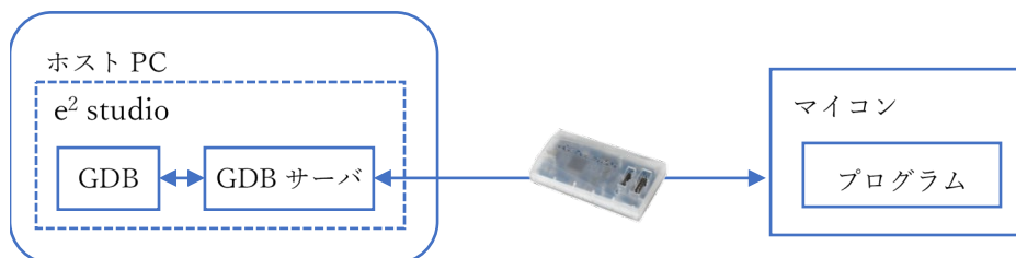
図1 e 2 studio で GDB と GDB サーバを使用した接続の例
