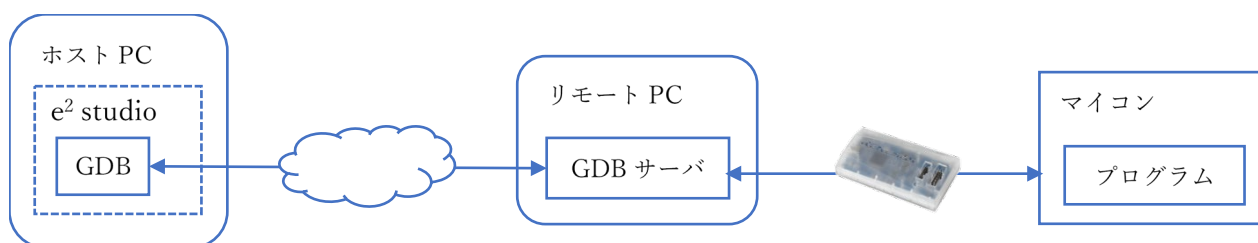
図2 e 2 studio からリモート PC 上の GDB サーバに接続する例
