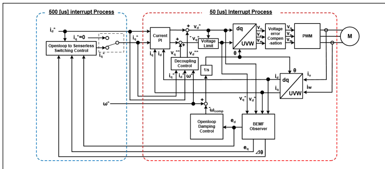
図 3-8 センサレスベクトル制御概略ブロック図(オープンループ制御時)
