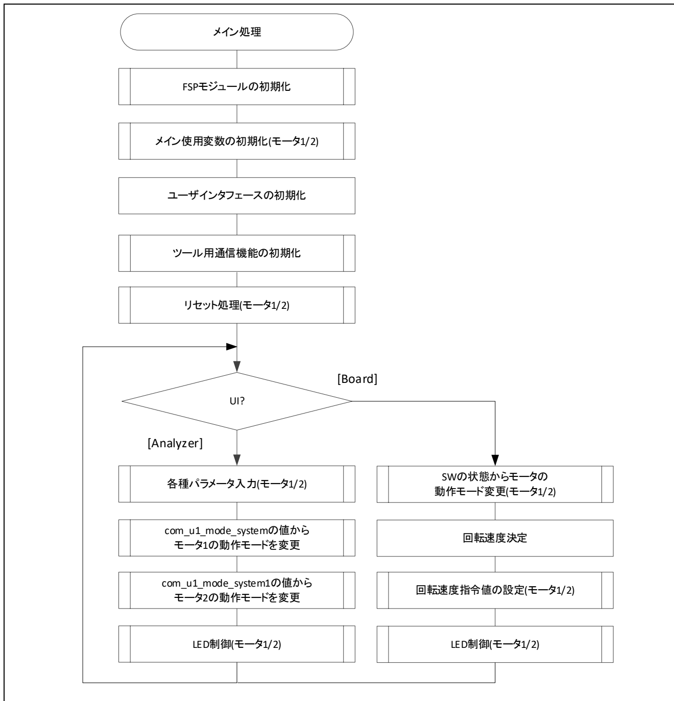
図 3-15 メイン処理フローチャート
