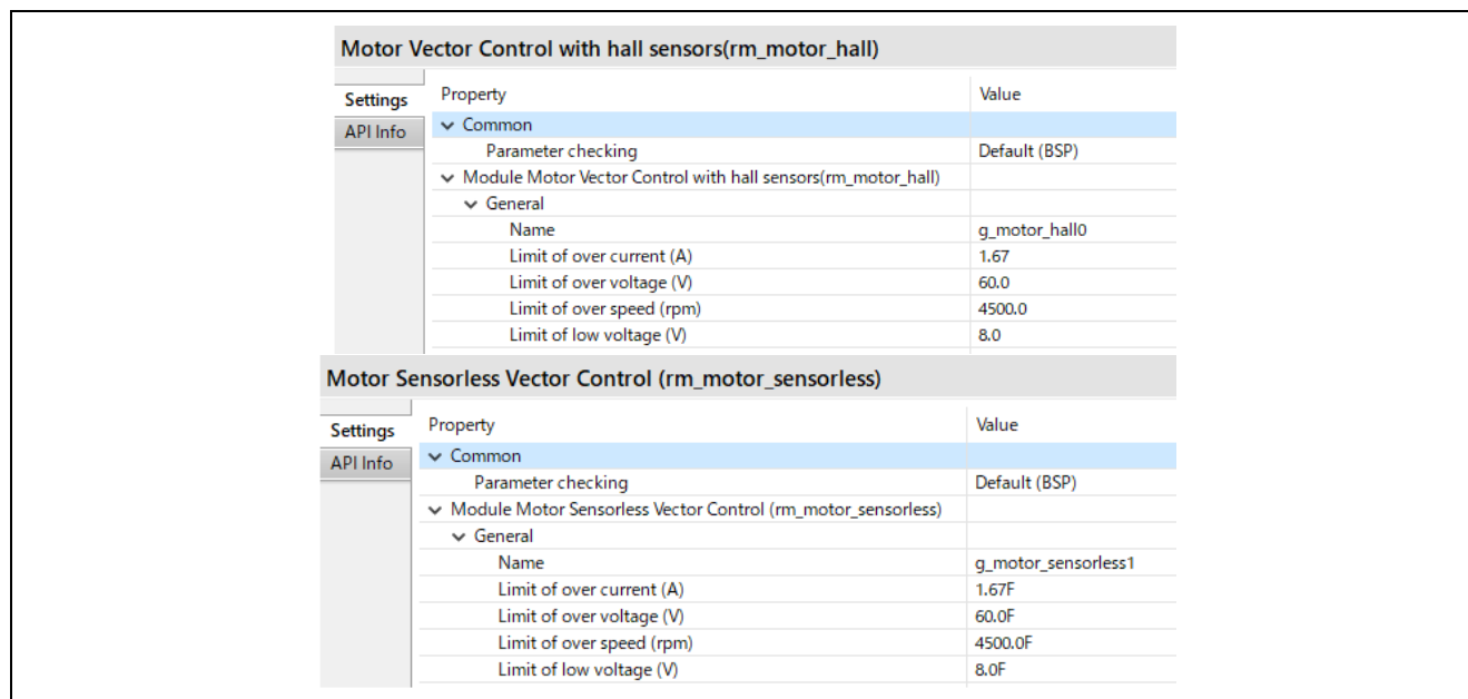
図 3-10 ホールセンサ/センサレスベクトル制御の FSP コンフィグレーション
