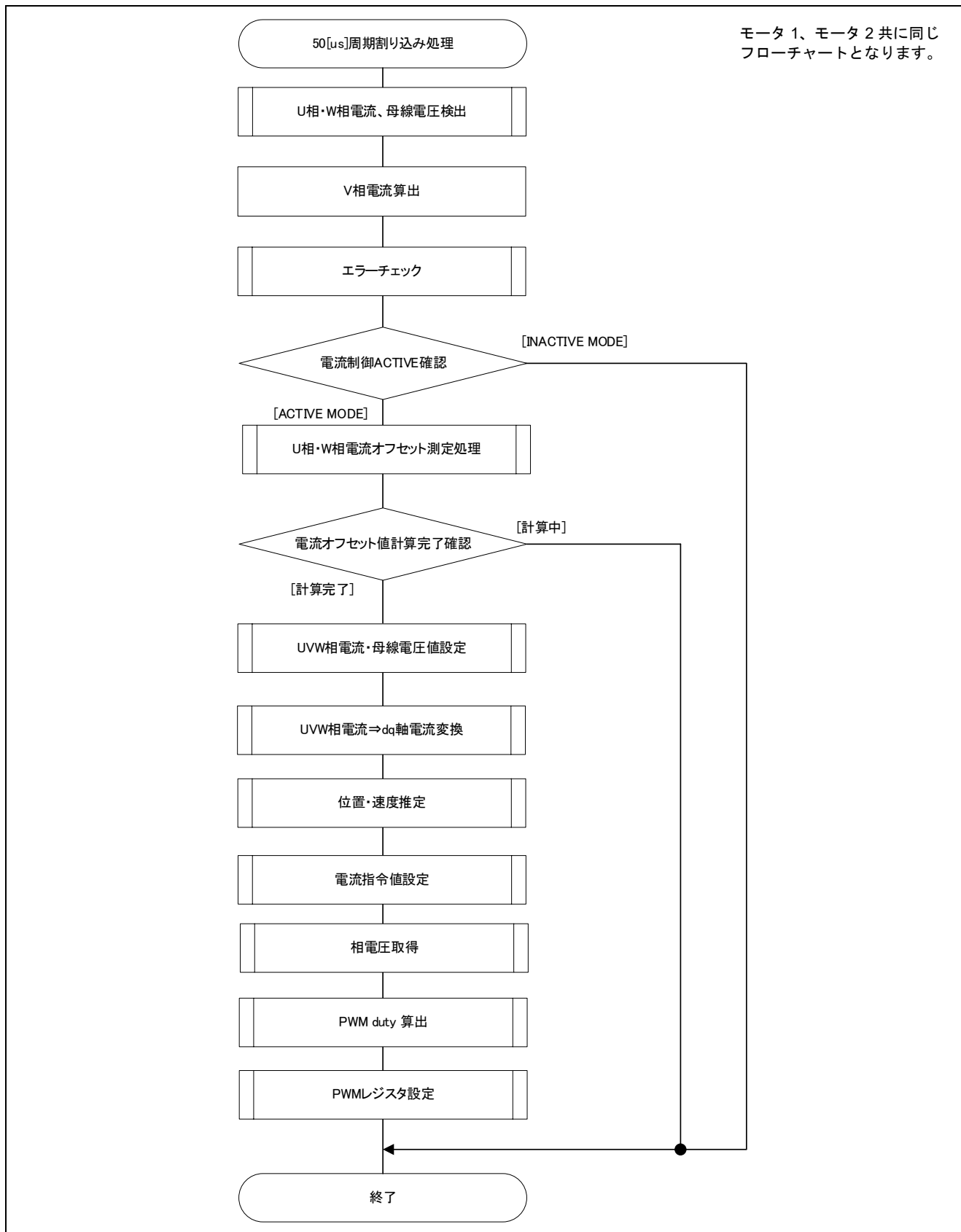
図 3-16 50[us]周期割り込み処理フローチャート
