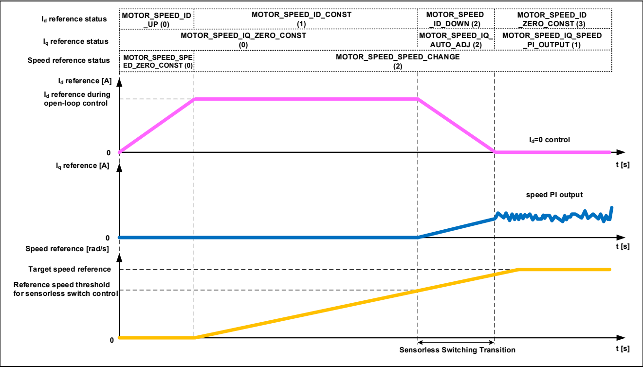
図 3-5 センサレスベクトル制御ソフトウェアの始動制御内容
