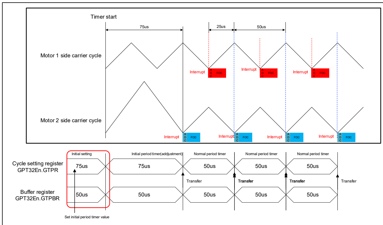
図 3-6 キャリア出力調整
