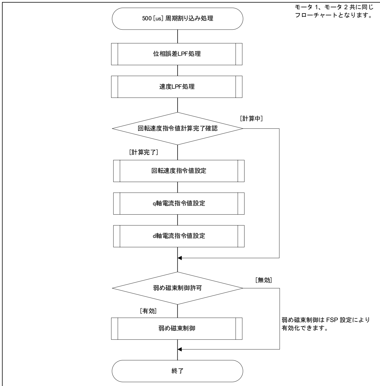
図 3-17 500 [us]周期割り込み処理フローチャート
