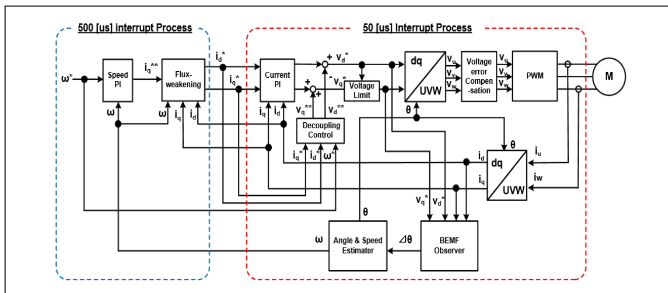
図 3-9 センサレスベクトル制御概略ブロック図(センサレス制御時)
