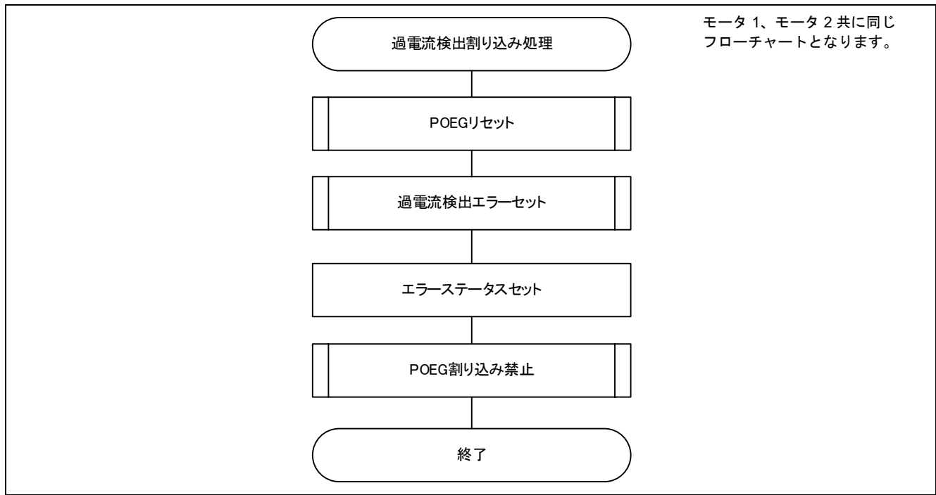
図 3-18 過電流検出割り込み処理フローチャート
