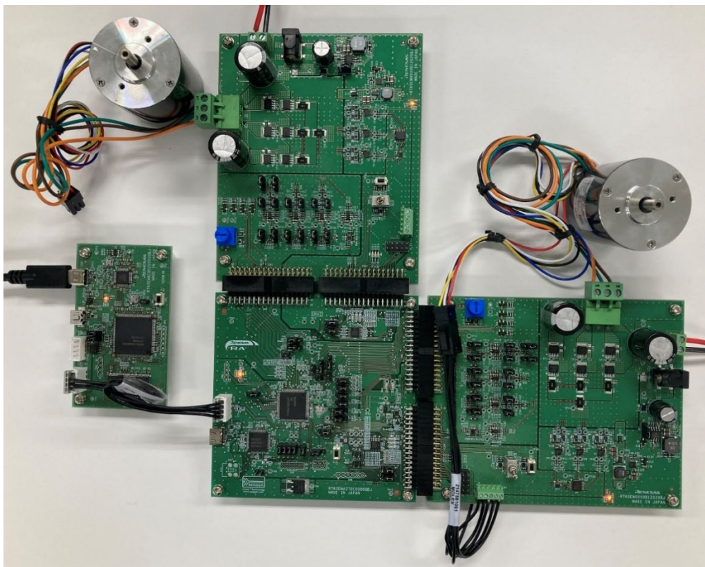
図 2-4 CPU ボードとインバータボードの接続
