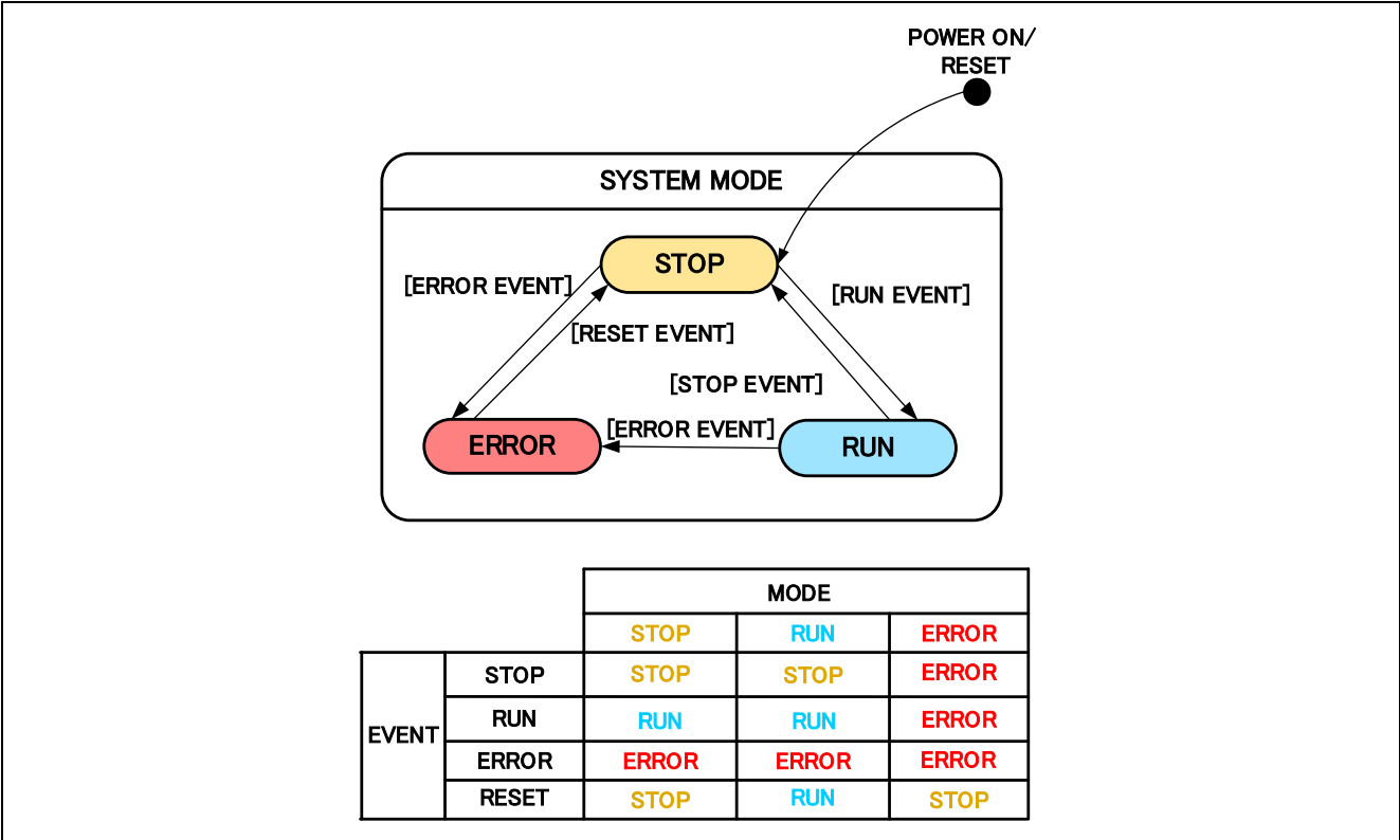
図 3-3 ホールセンサ/センサレスベクトル制御ソフトウェアの状態遷移図
