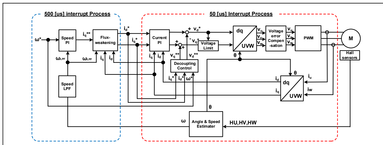
図 3-7 ホールセンサベクトル制御概略ブロック図
