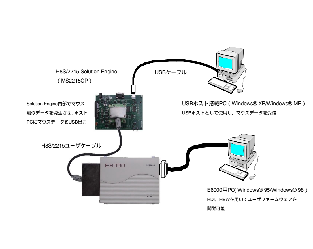
図 3.1 デバイスの接続形態
