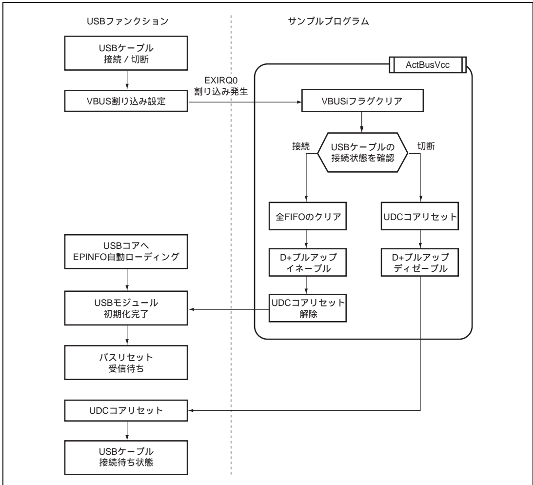
図 5.5 ケーブル接続時割り込み
