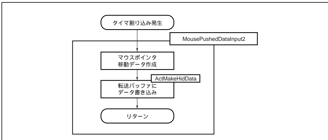
図 5.16 HID データ生成
