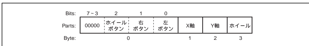
図 2.4 レポートプロトコルフォーマット
