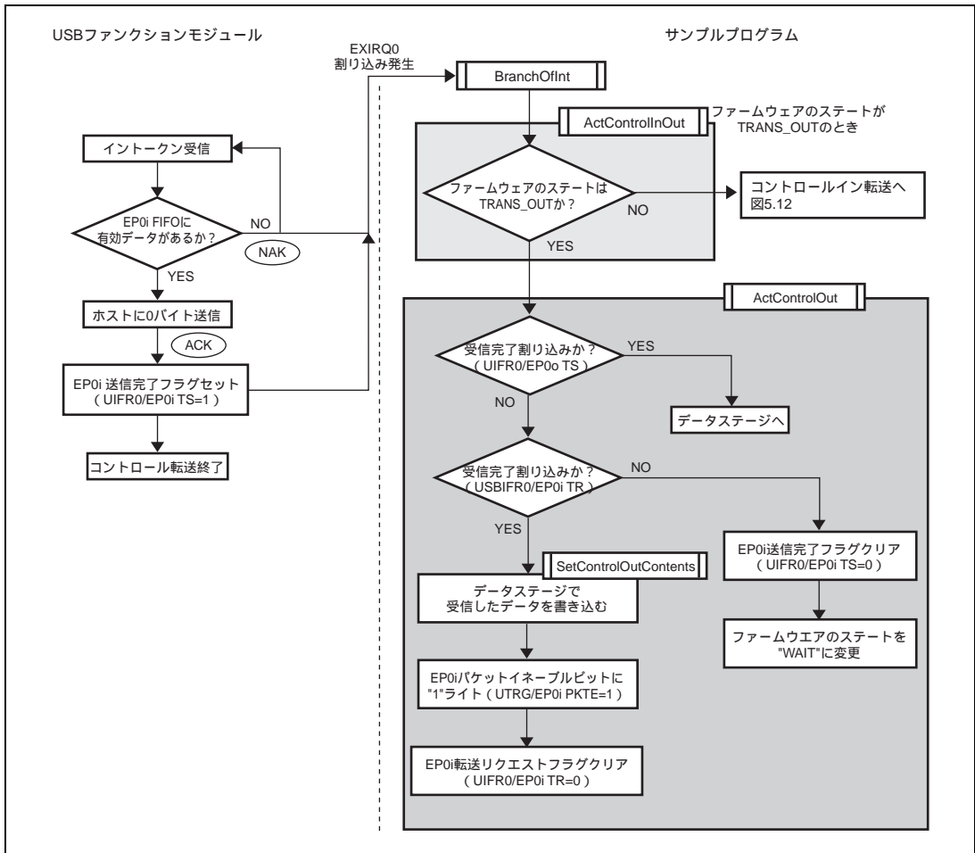
図 5.13 ステータスステージ (コントロールアウト転送)
