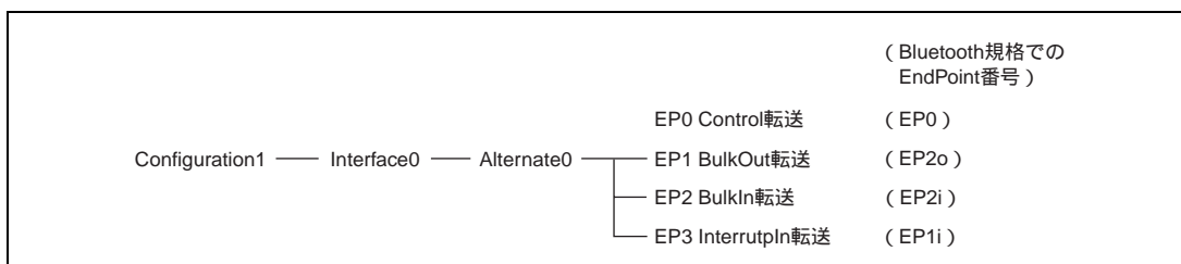
図 5.4 サンプルプログラムの EndPoint 構成
