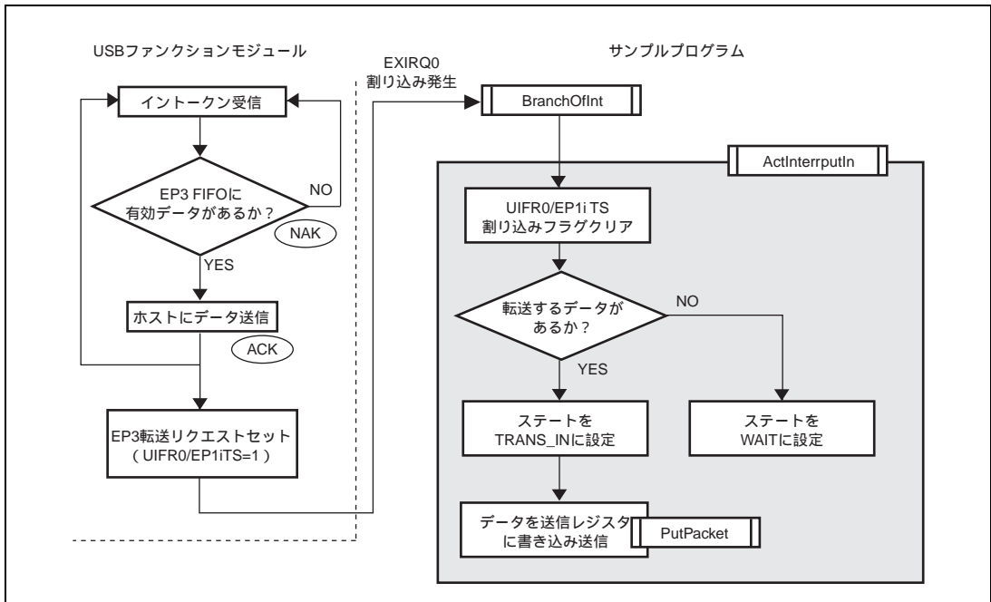
図 5.15 インタラプトイン転送
