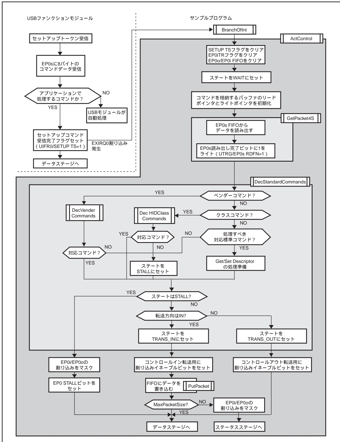
図 5.9 セットアップステージ
