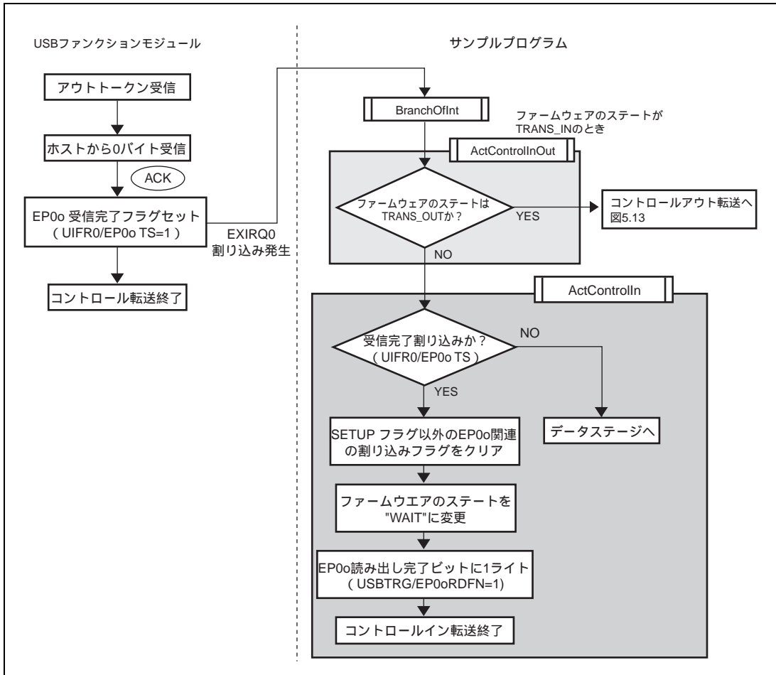
図 5.12 ステータスステージ (コントロールイン転送)
