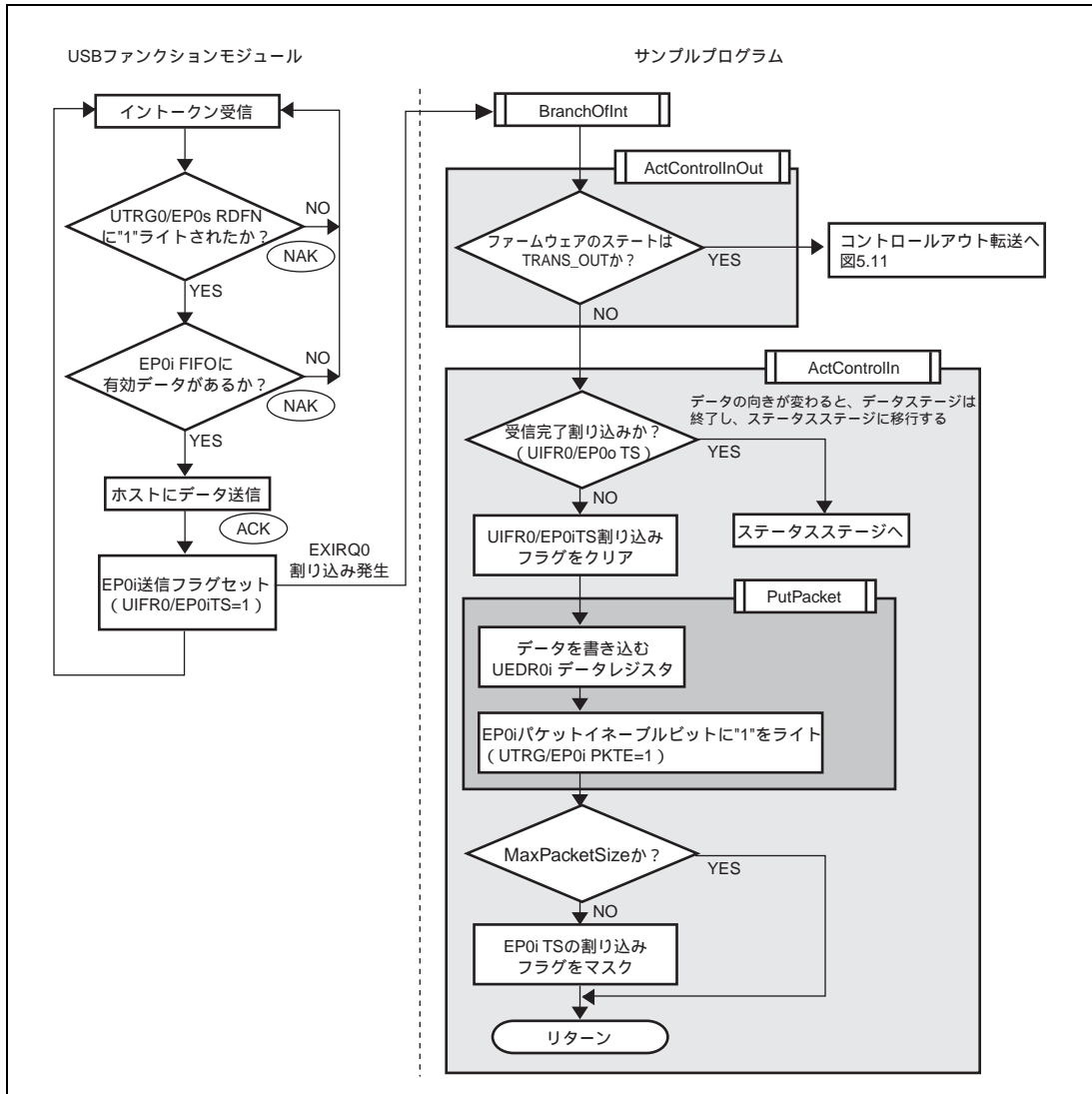
図 5.10 データステージ (コントロールイン転送)
