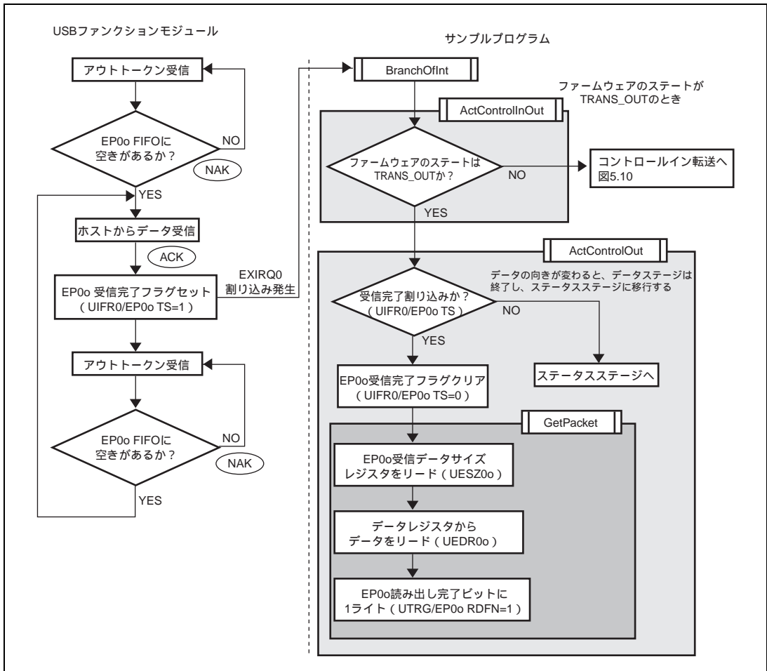
図 5.11 データステージ (コントロールアウト転送)
