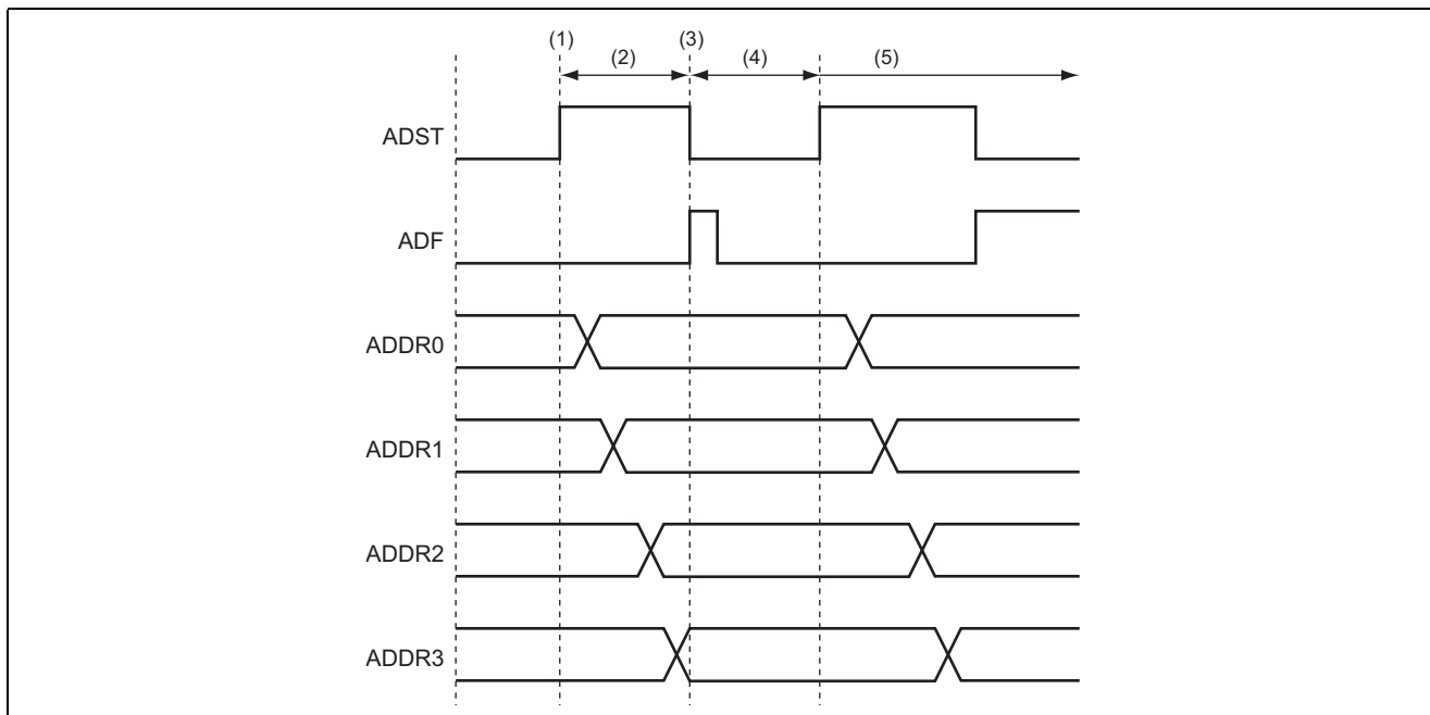
図3 A/D 変換タイミング
