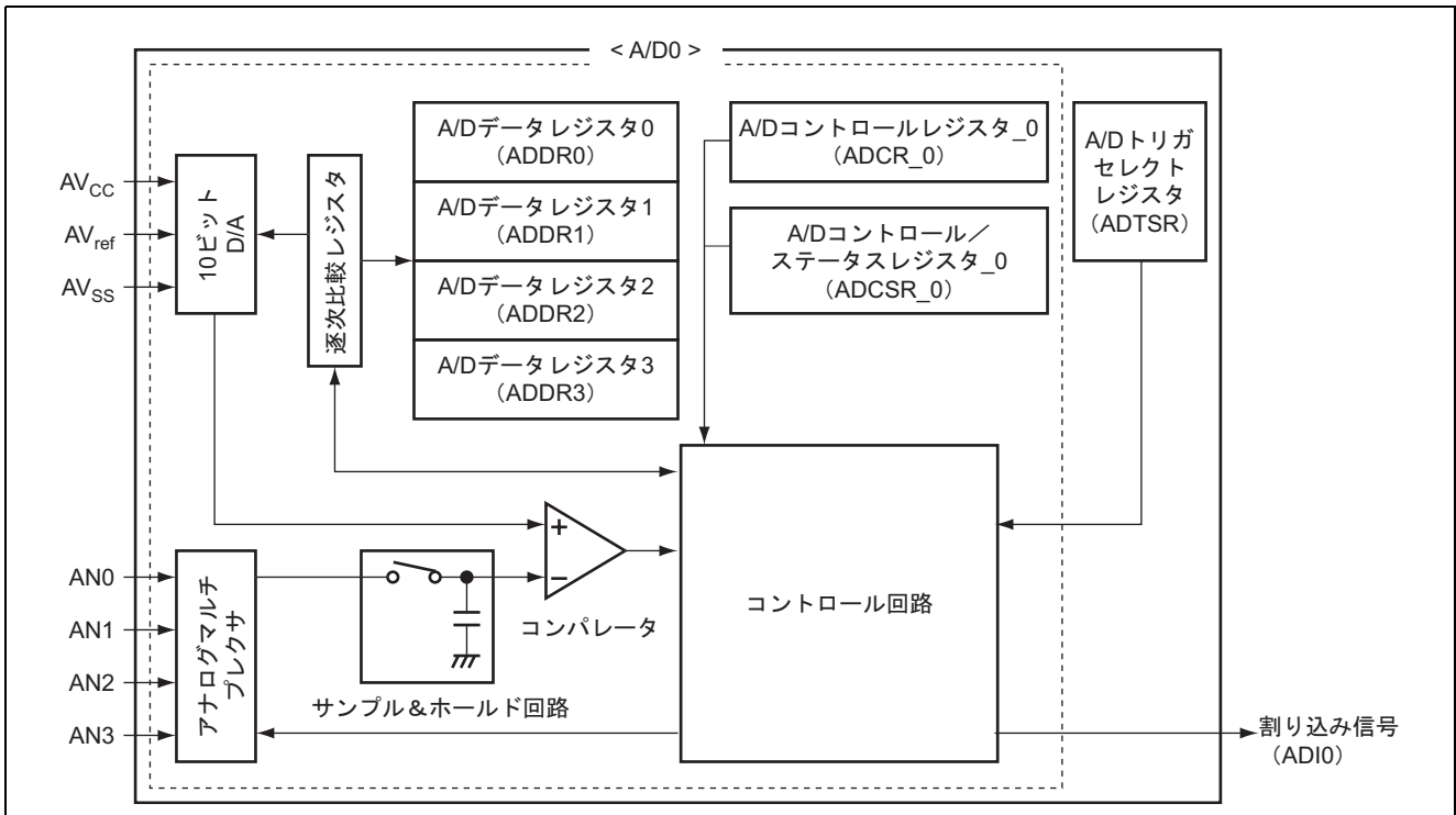
図 2 A/D 変換器(ch0~3)のブロック図
