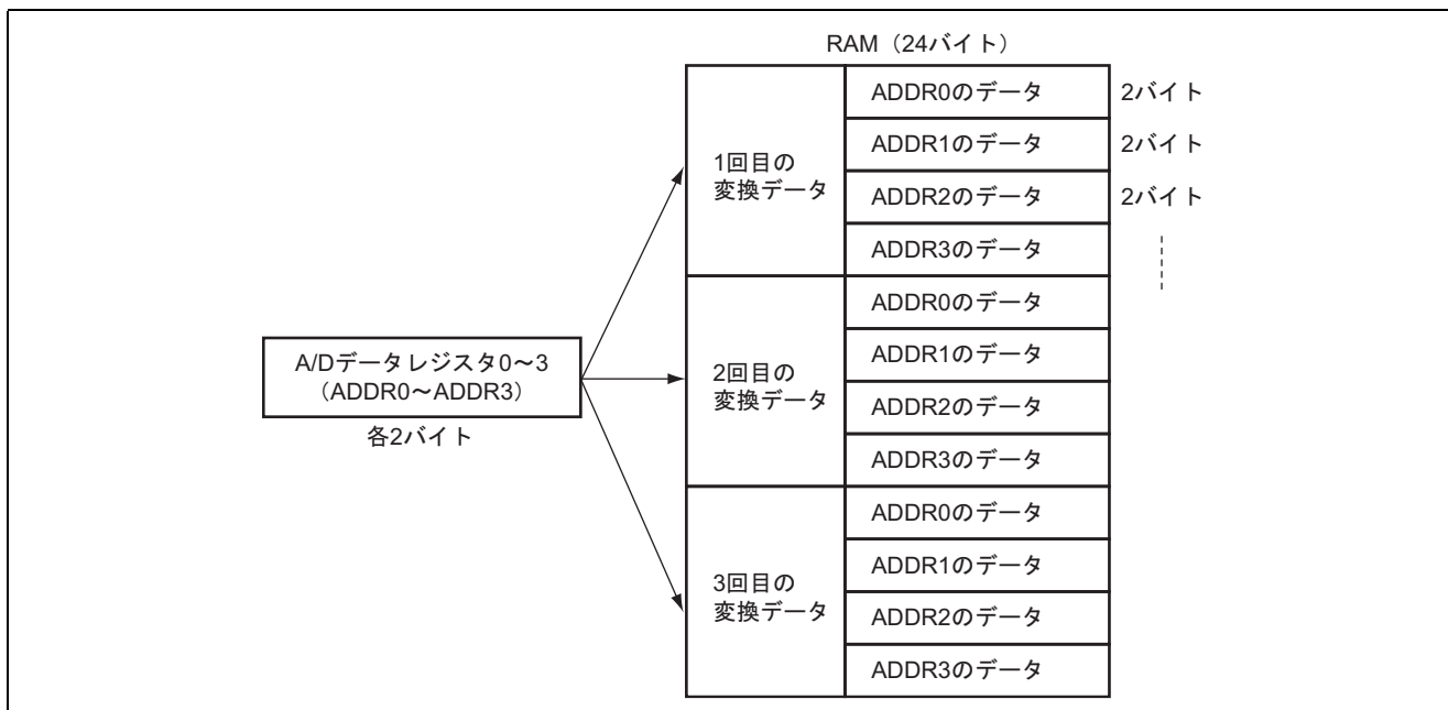
図 1 A/D 変換データの格納
