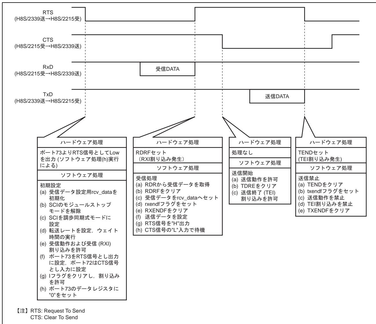
図4 調歩同期式 SCI 動作原理
