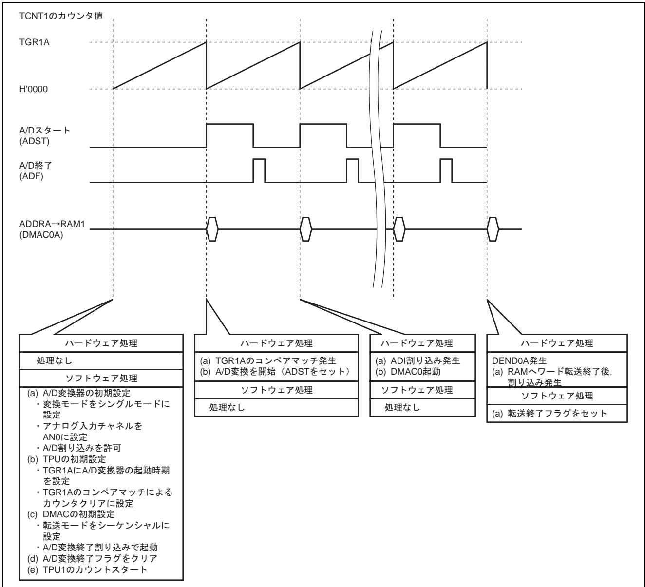
図3 タイマトリガによる A/D 変換動作原理
