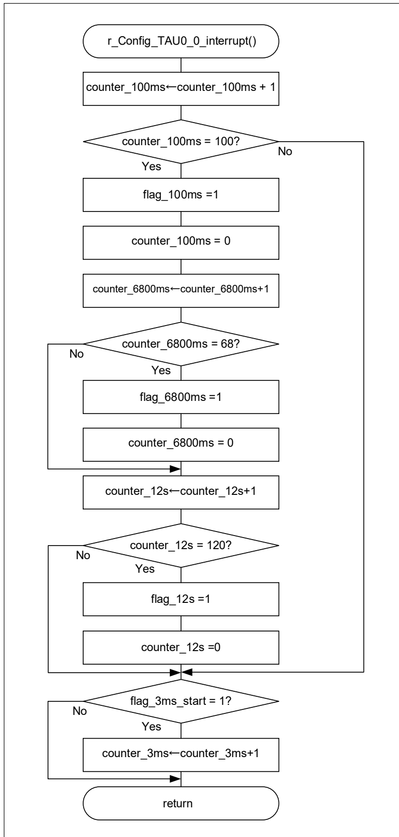
図 4-19 1ms インターバル・タイマ割り込み処理関数
