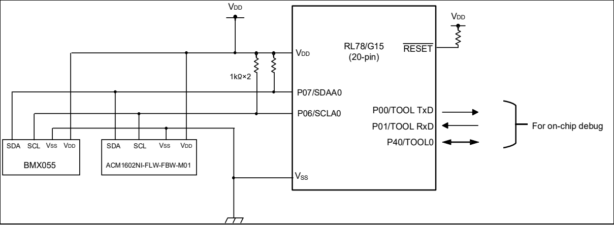
図 3-1 ハードウェア構成
