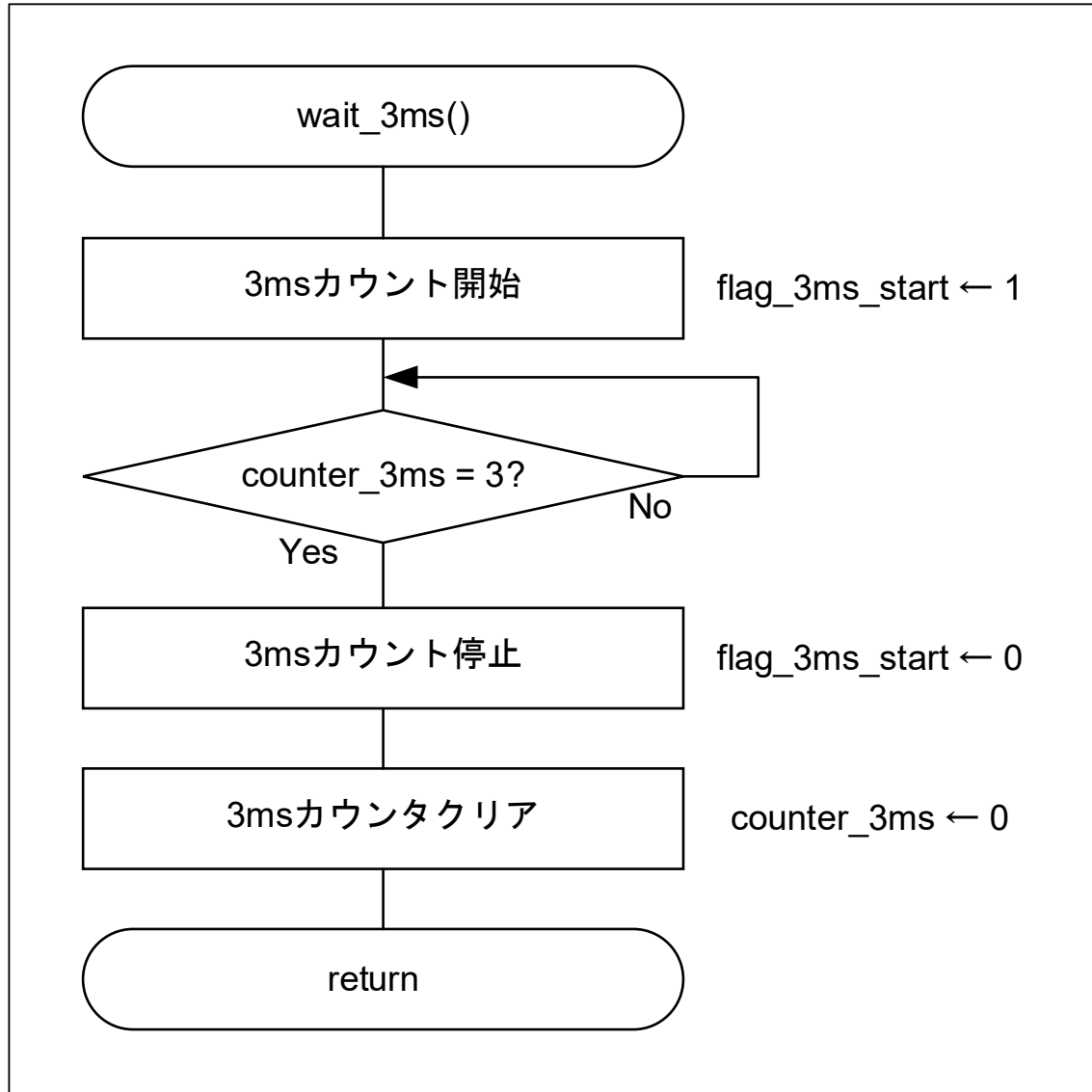
図 4-17 3ms ウェイト関数
