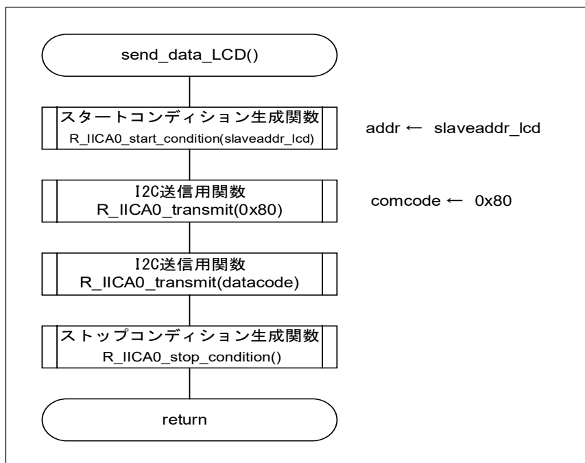
図 4-10 データ送信用 (LCD) 関数
