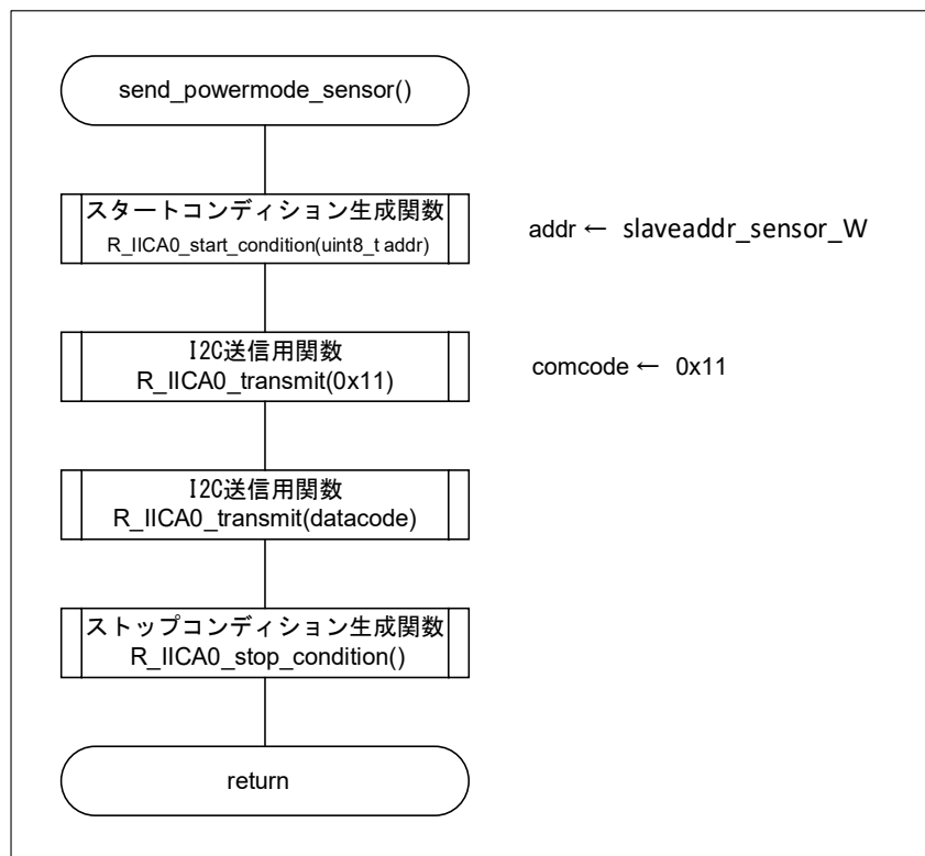
図 4-13 ジャイロセンサへのパワーモード設定用関数
