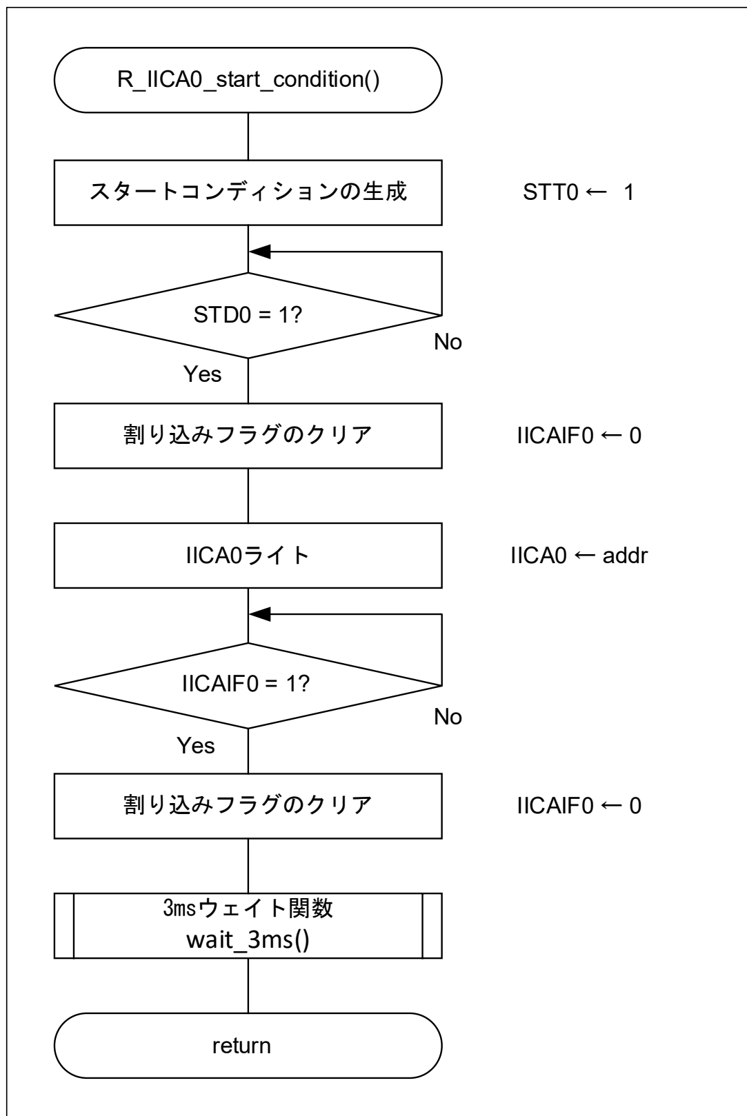
図 4-6 スタートコンディションの生成関数
