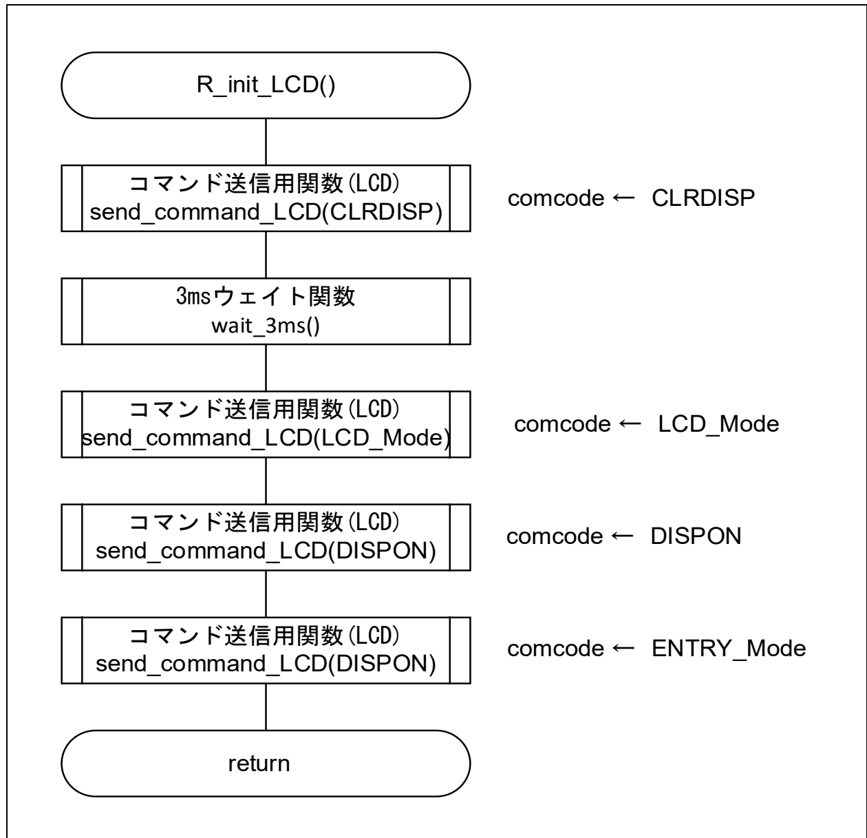
図 4-4 LCD 初期設定関数
