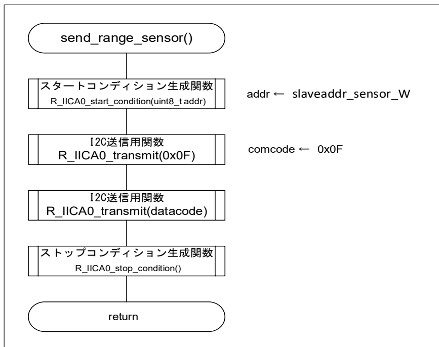
図 4-11 ジャイロセンサへの測定レンジ設定用関数
