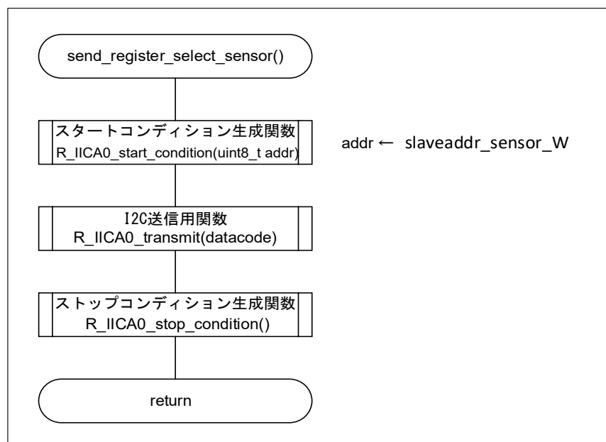
図 4-14 ジャイロセンサへのレジスタ設定用関数
