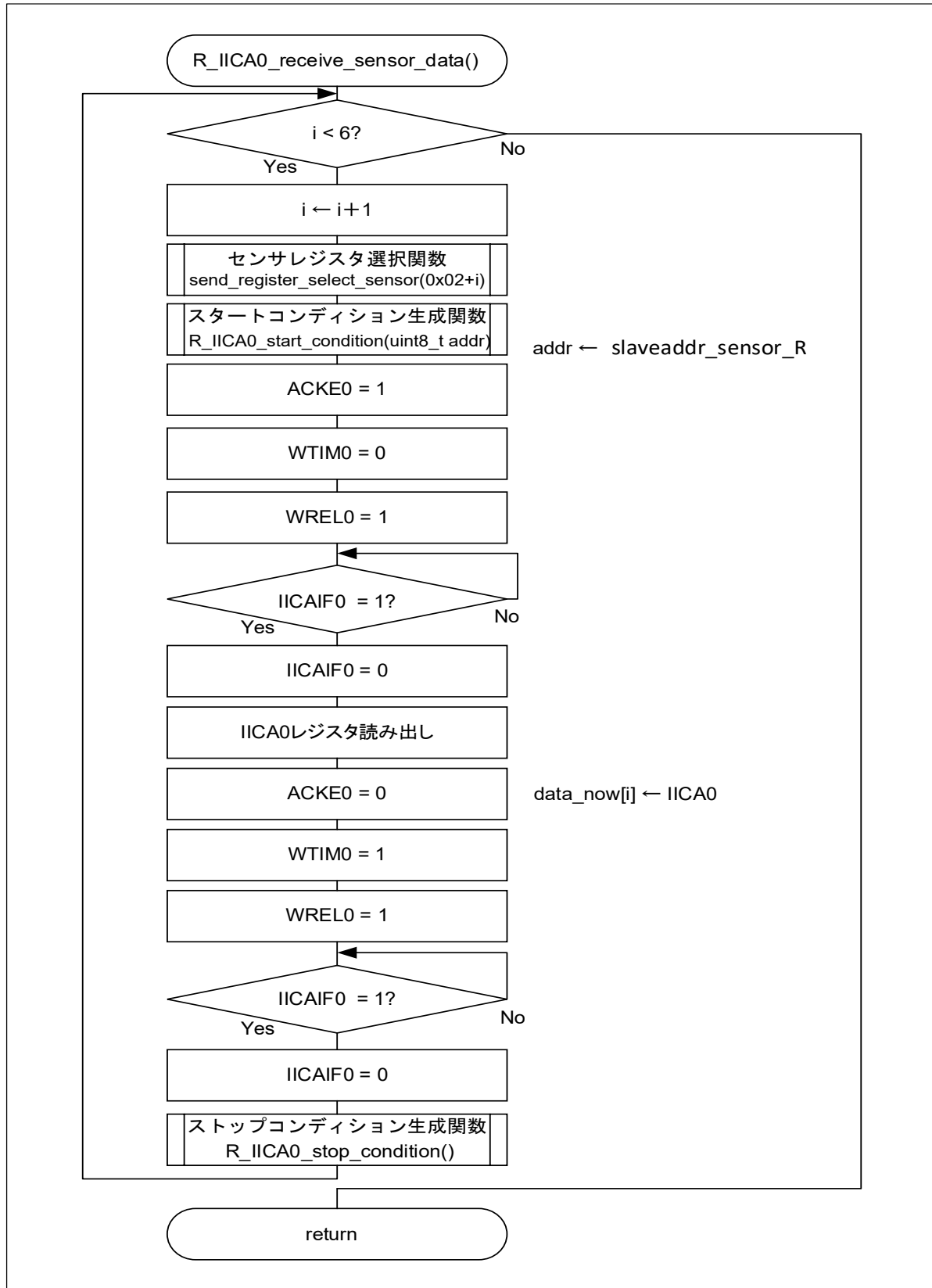
図 4-15 I2C 受信用関数
