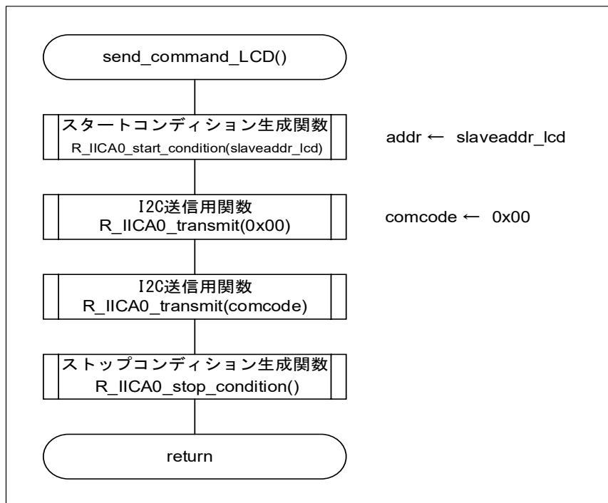
図 4-9 コマンド送信用 (LCD) 関数
