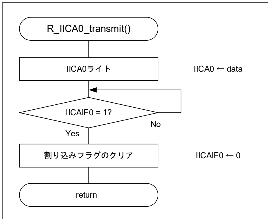
図 4-8 I2C 送信用関数
