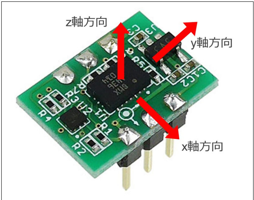
図 1-1 ジャイロセンサ (BMX055) 軸方向
