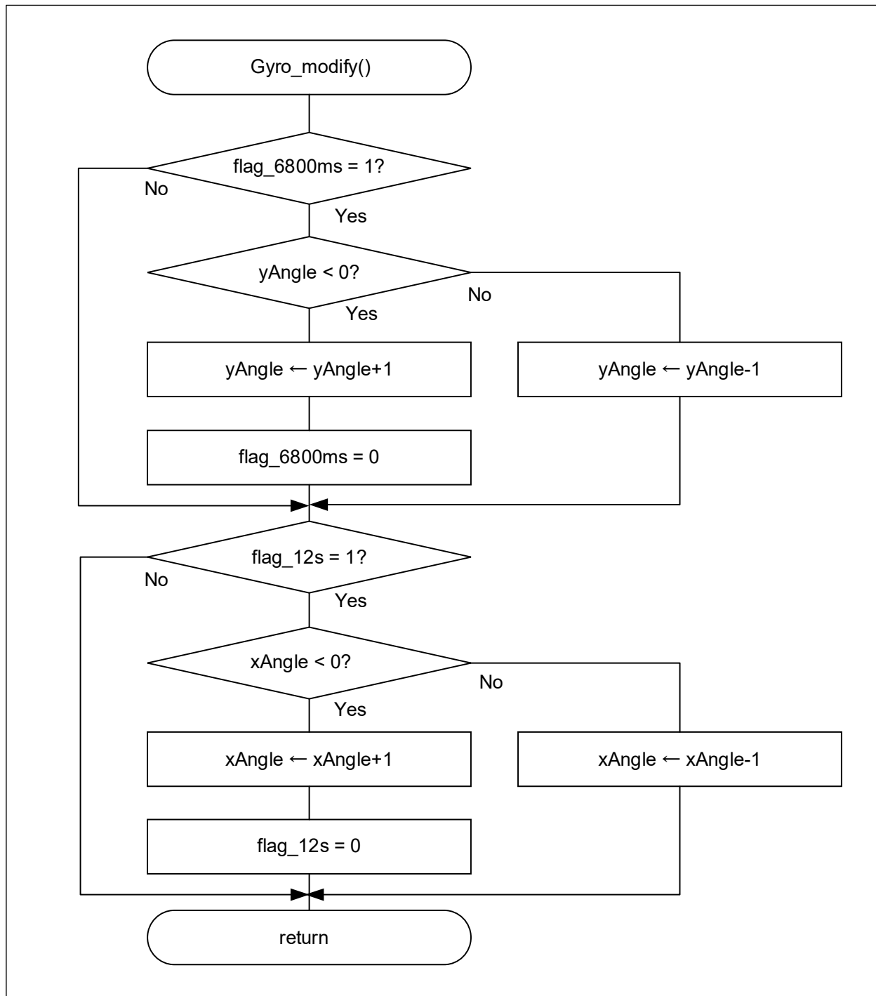
図 4-18 ジャイロドリフト補正関数
