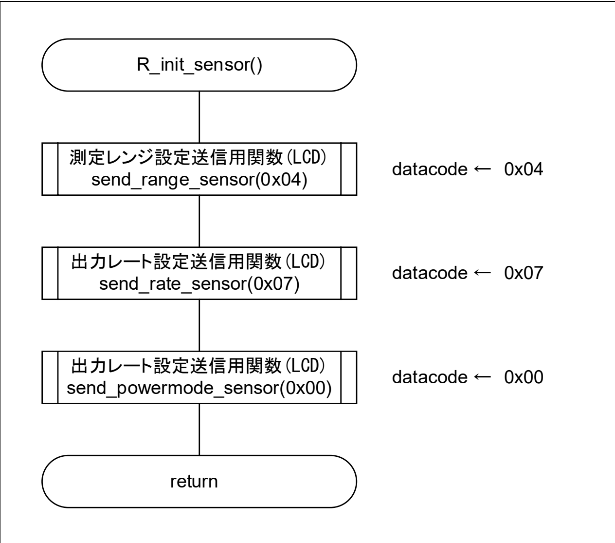
図 4-5 ジャイロセンサ初期設定関数
