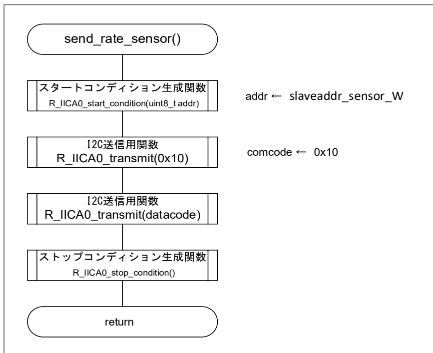
図 4-12 ジャイロセンサへの出力レート設定用関数
