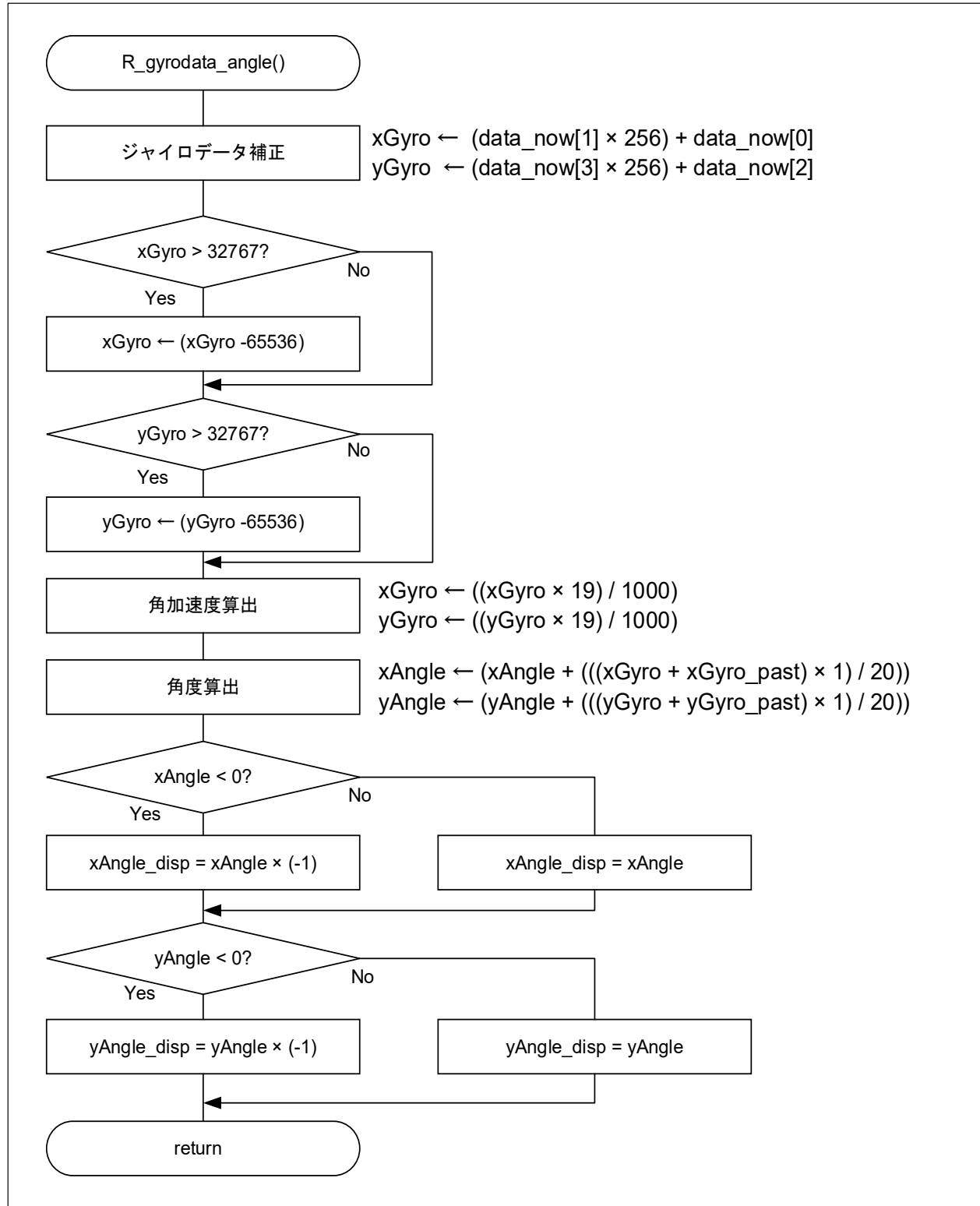
図 4-16 角度算出用関数
