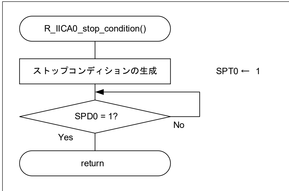
図 4-7 ストップコンディションの生成関数
