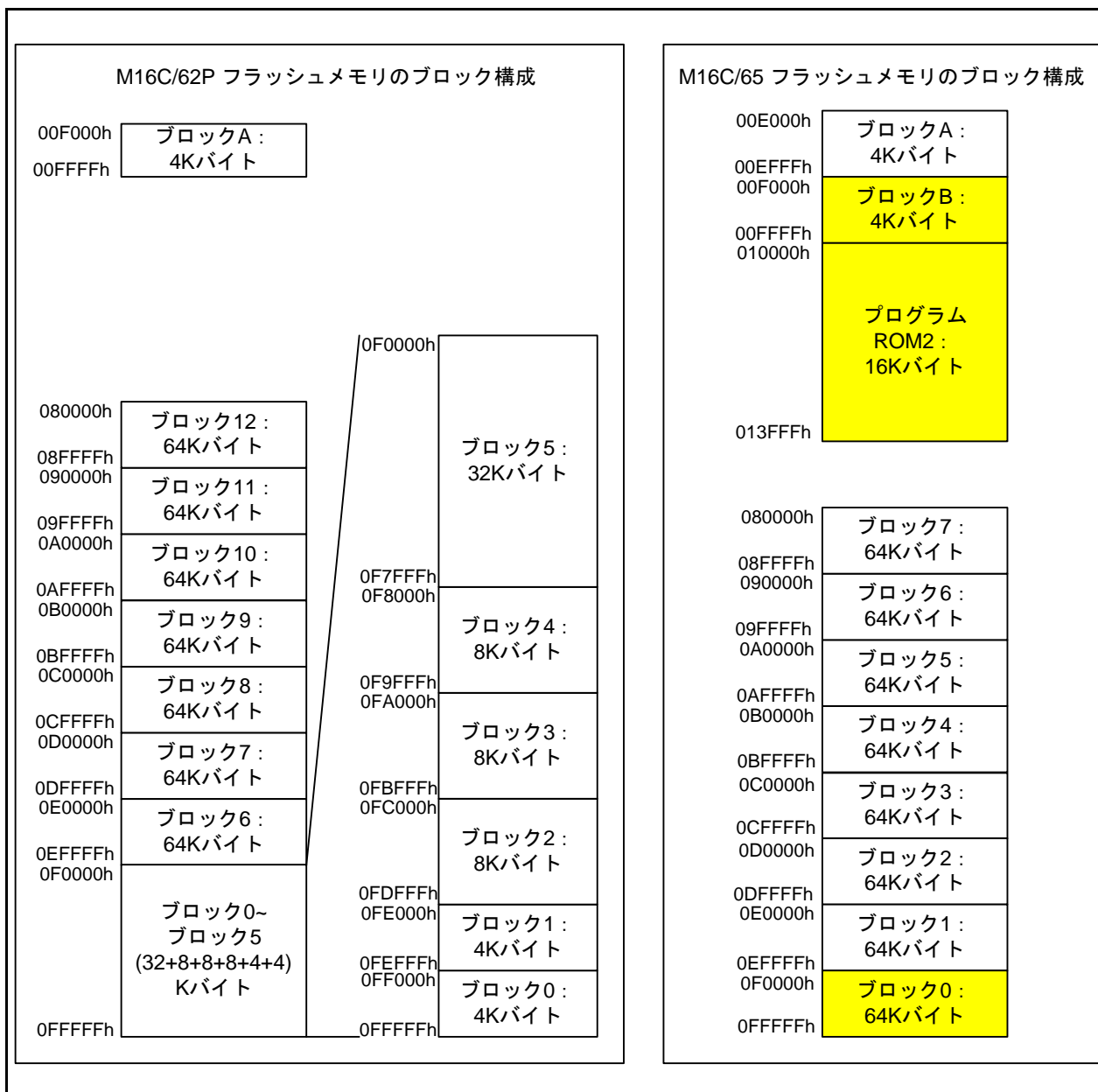
図 2.1 M16C/62P と M16C/65 のフラッシュメモリのブロック構成の相違点
