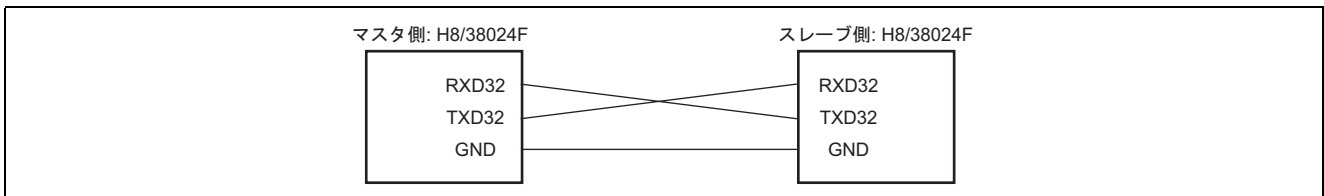
図3 マスタ-スレーブ間の接続図
