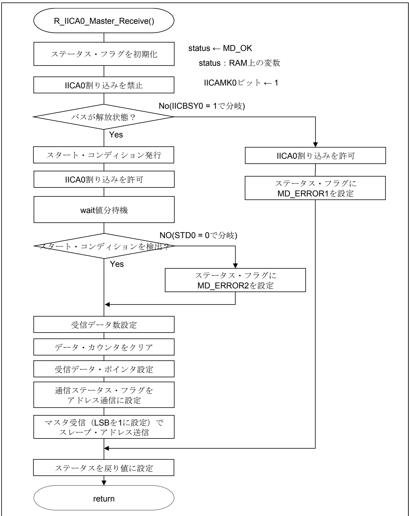
図 5.15 マスタ受信開始要求処理
