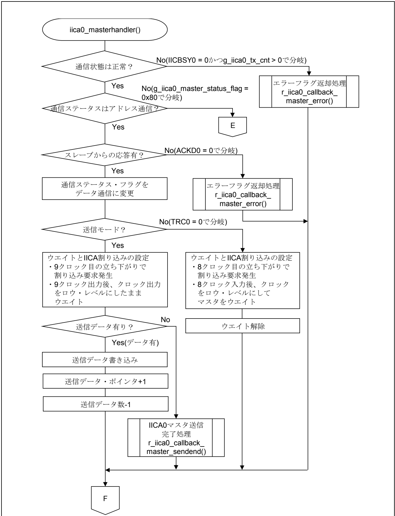
図 5.17 IICA0 マスタ通信処理 (1/2)
