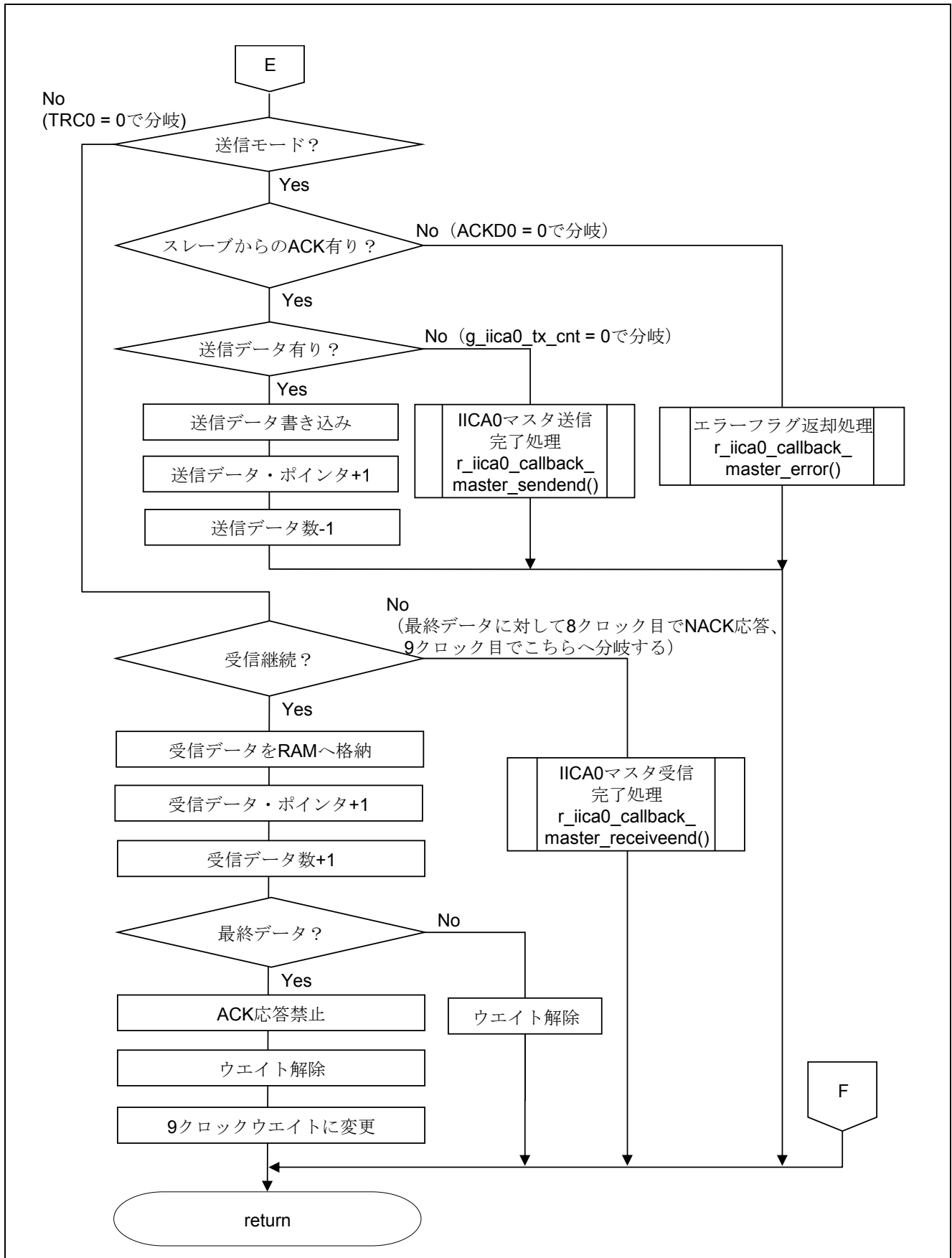
図 5.18 IICA0 マスタ通信処理 (2/2)
