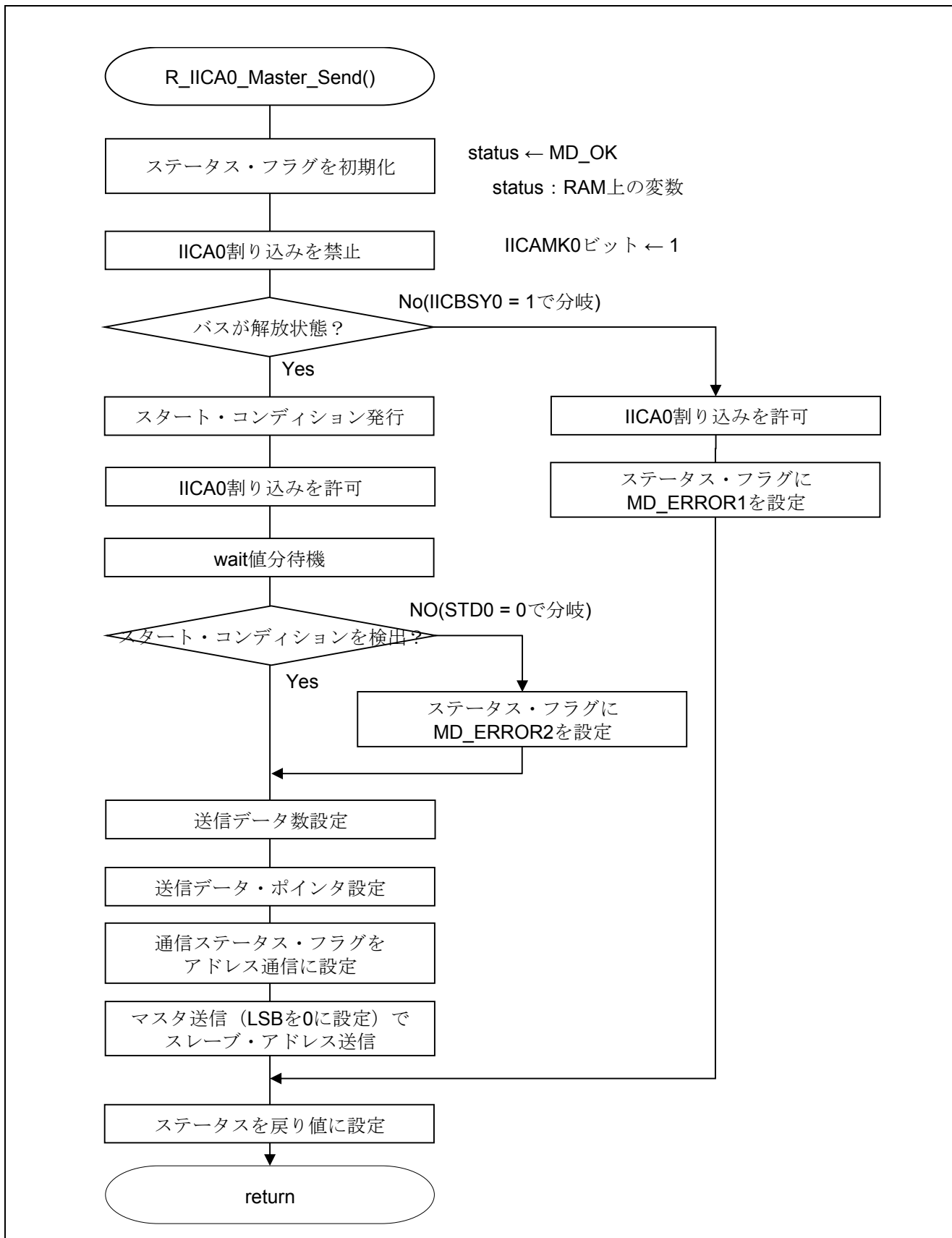
図 5.14 マスタ送信開始要求処理
