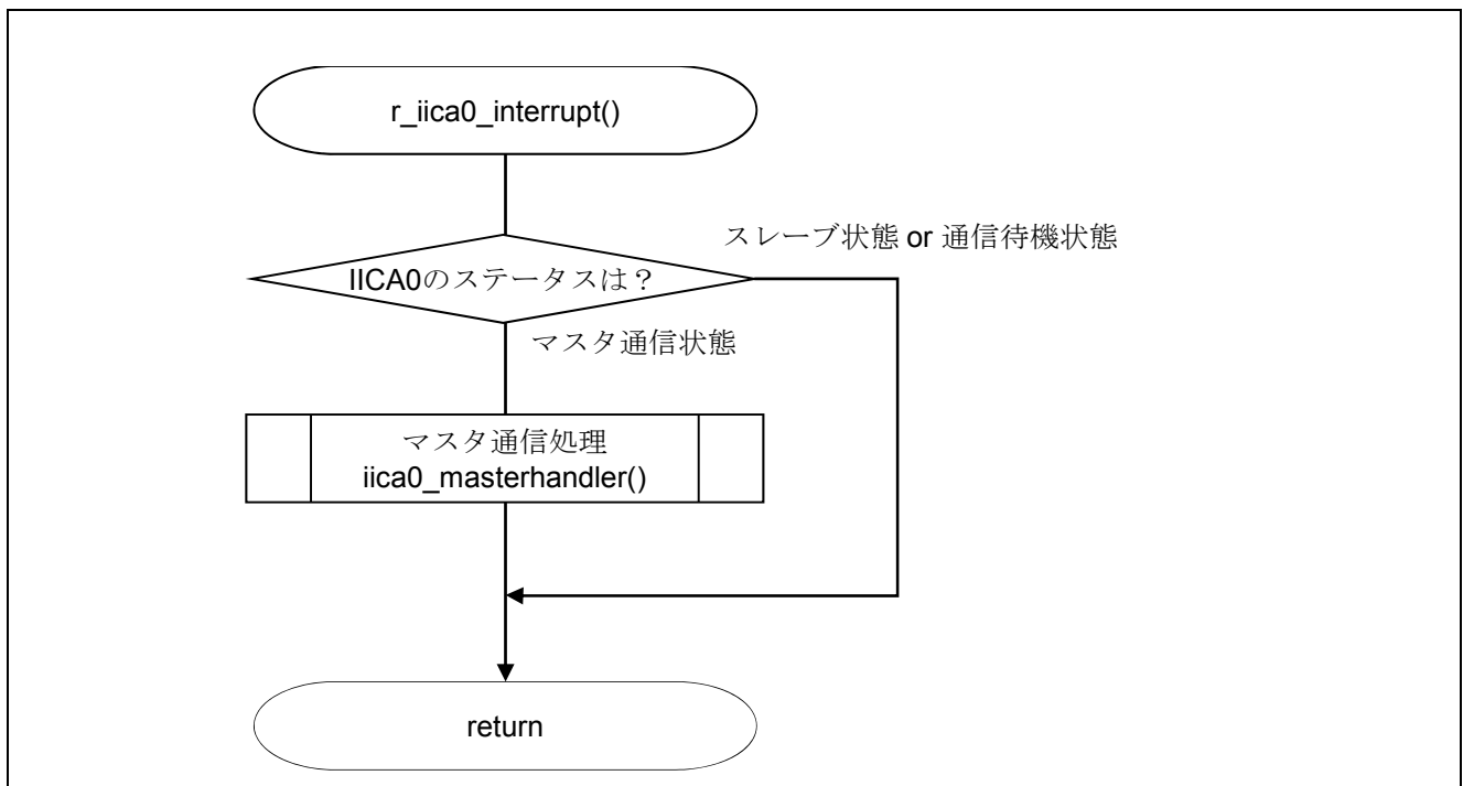
図 5.16 IICA0 割り込み処理
