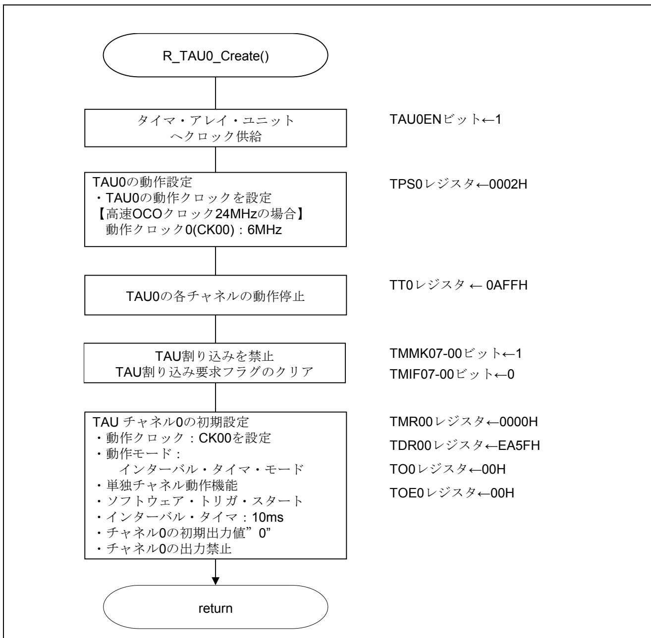
図 5.7 タイマ・アレイ・ユニットの設定
