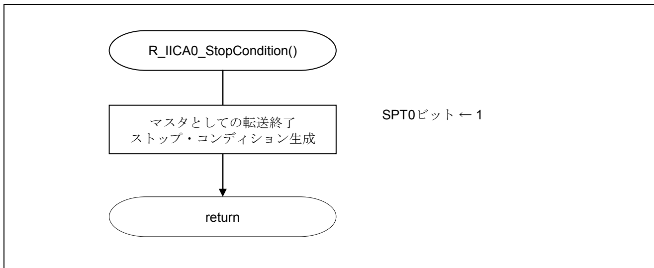
図 5.13 ストップ・コンディション発行処理
