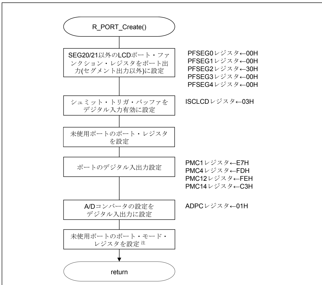
図 5.4 入出力ポートの設定
