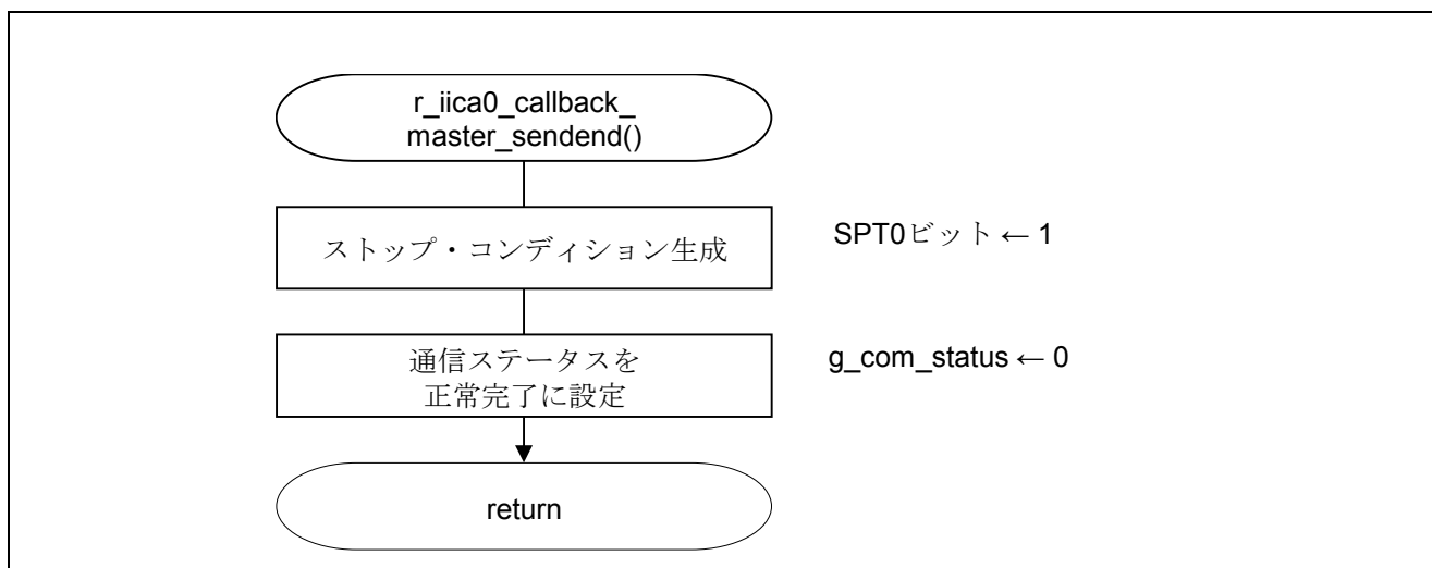
図 5.20 IICA0 マスタ送信完了処理
