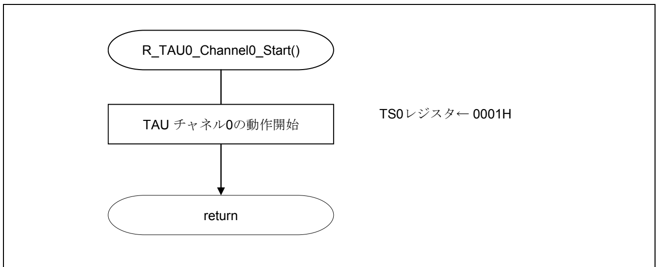
図 5.12 タイマ・アレイ・ユニット動作開始
