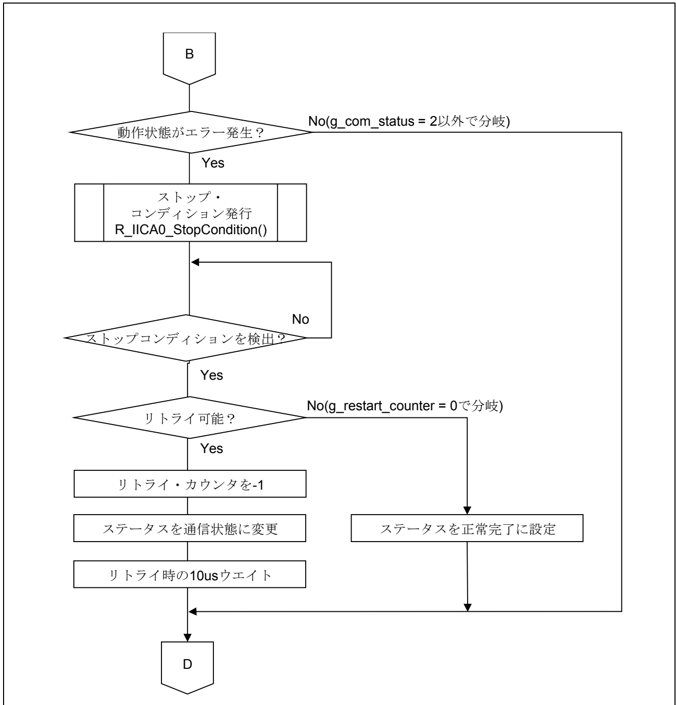
図 5.10 メイン関数 (3/3)
