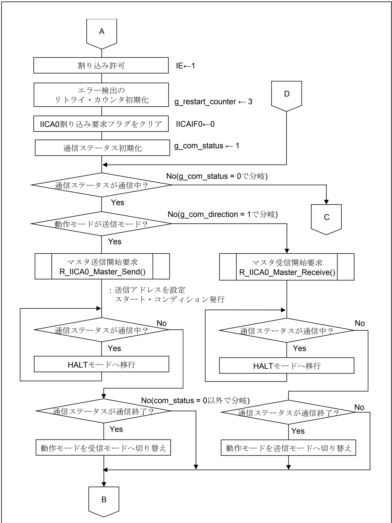
図 5.9 メイン関数 (2/3)
