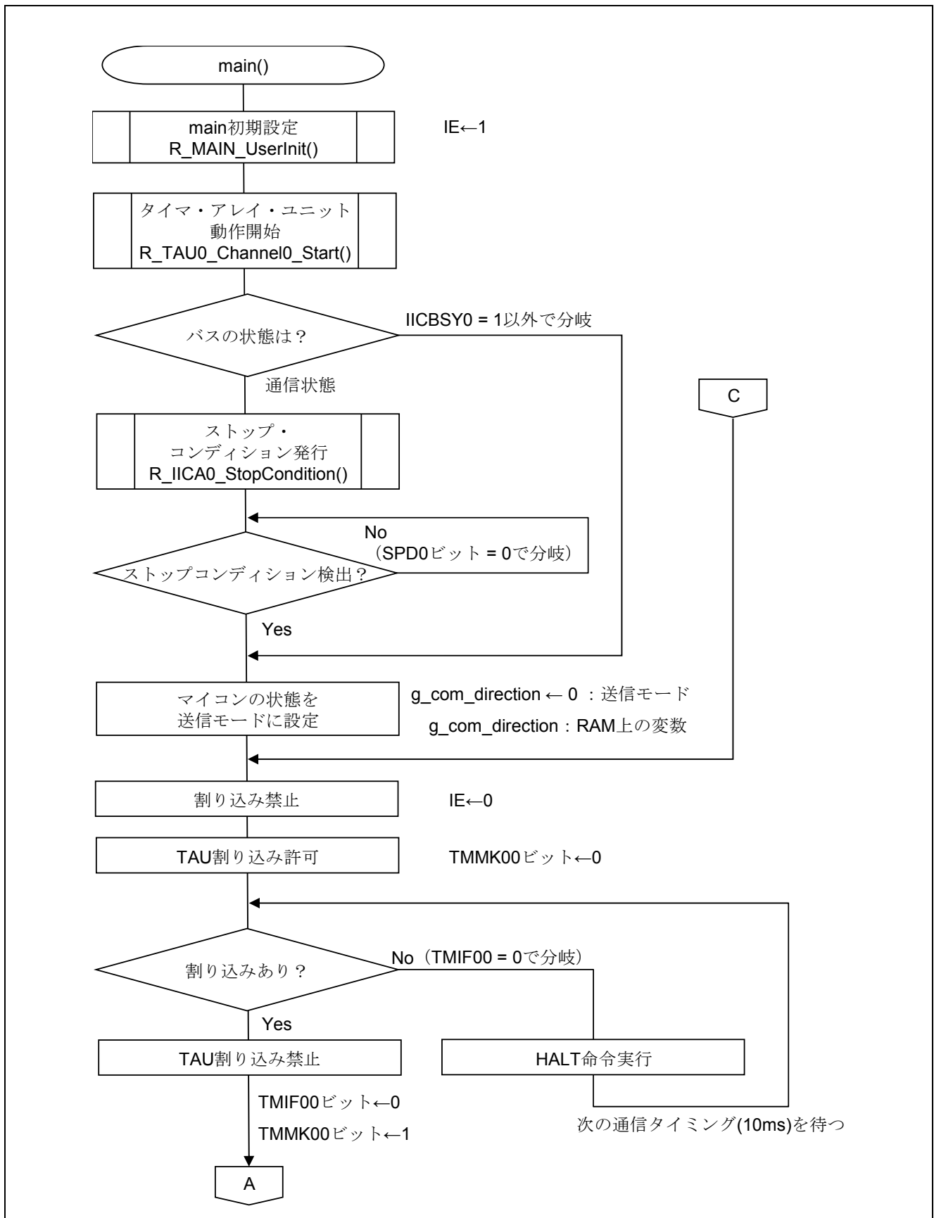
図 5.8 メイン関数 (1/3)
