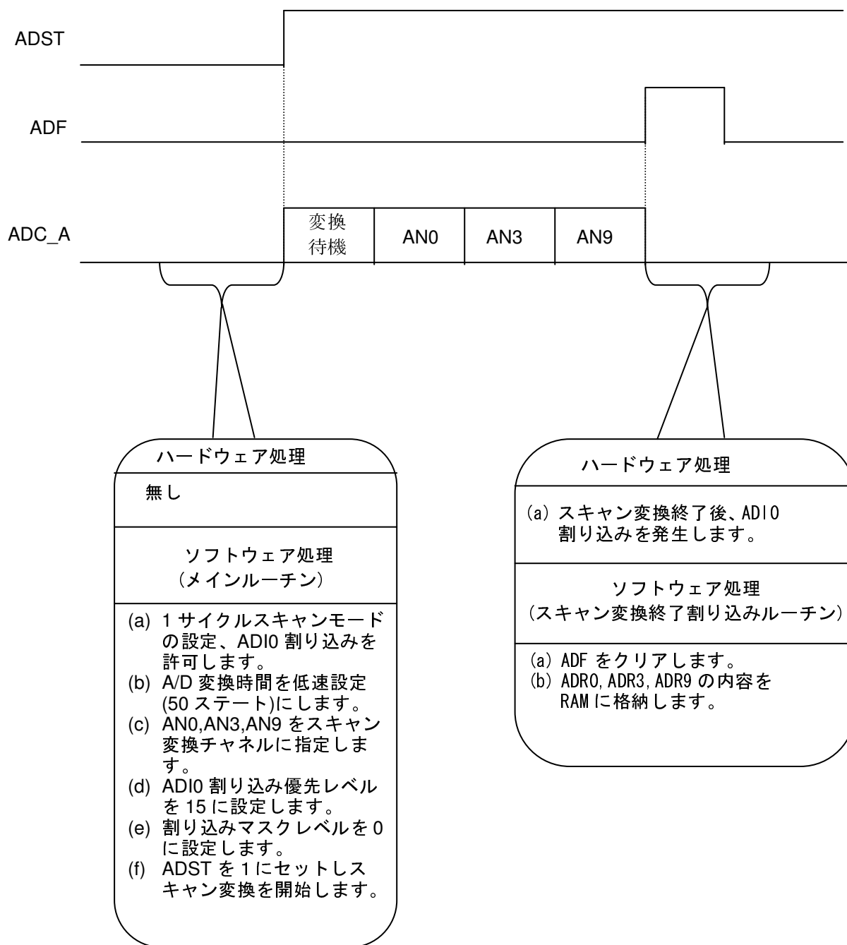
図 2 A/D 変換動作説明
