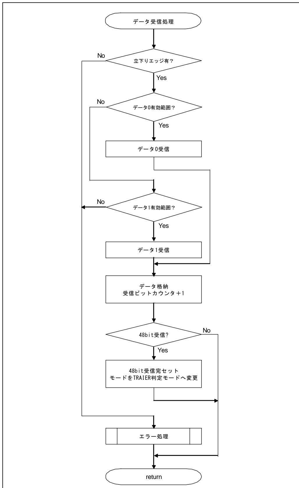
図 5.20 データ受信処理
