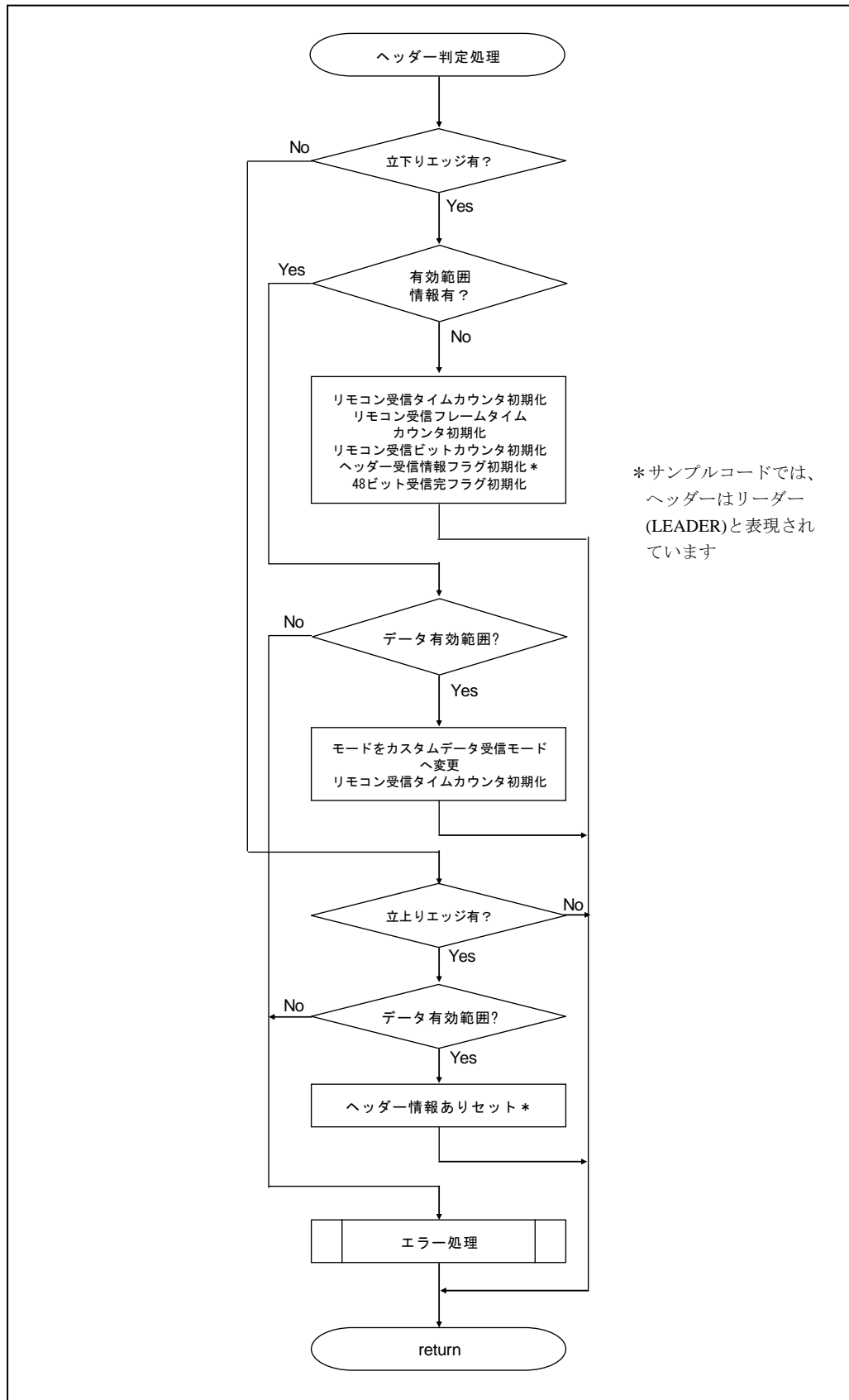
図 5.19 ヘッダー判定処理
