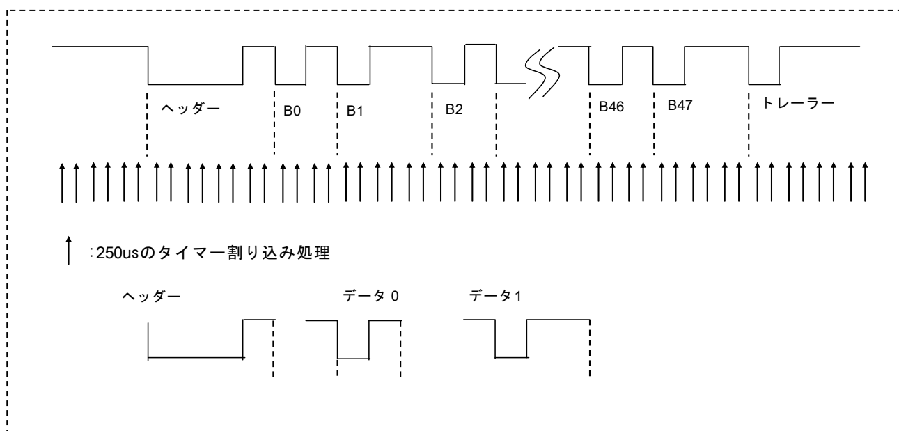
図 5.1 ヘッダーあり 48 ビットリモコンフォーマット受信タイミング
