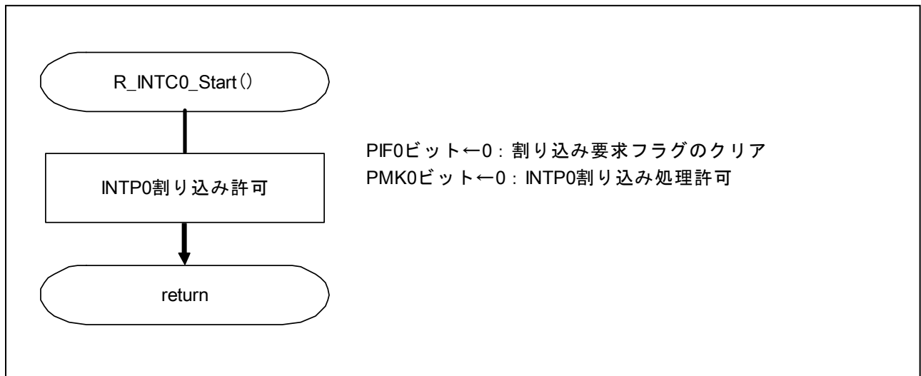
図 5.15 INTP0 割り込み許可
