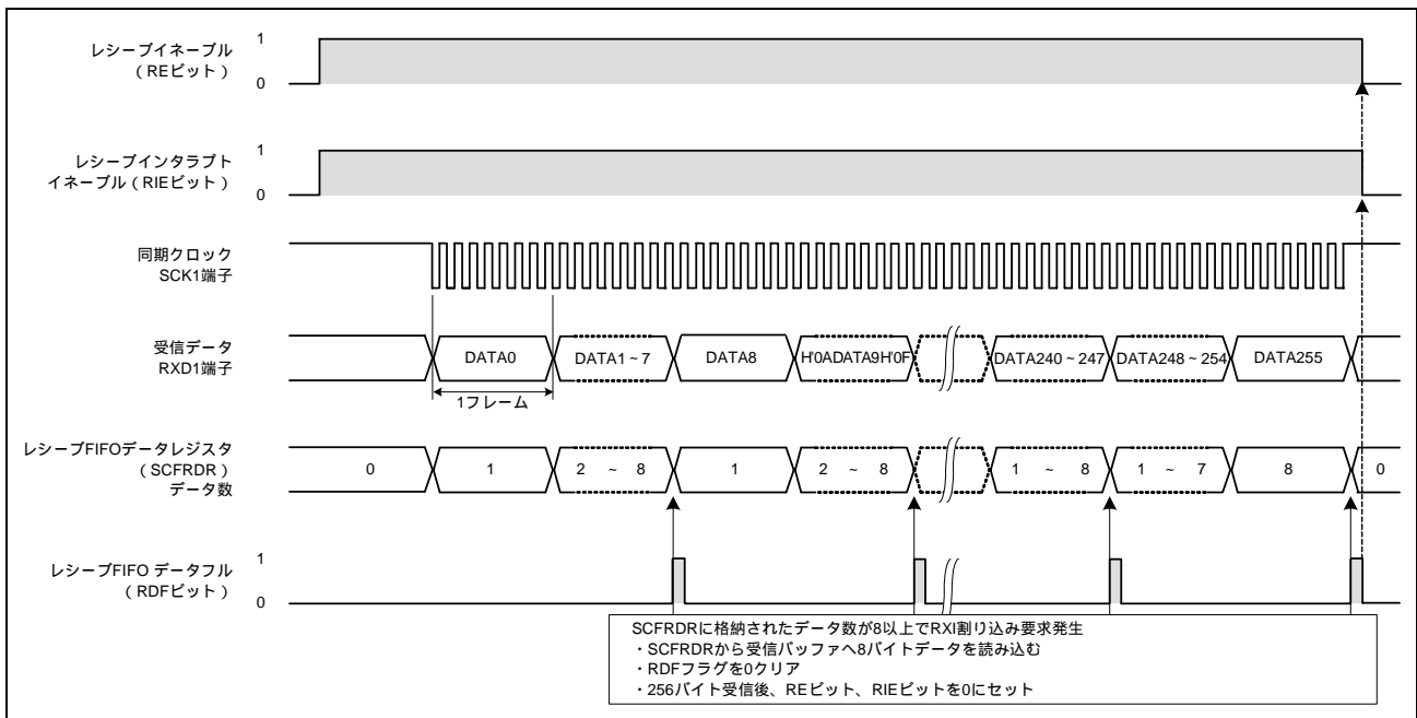
図3 受信動作
