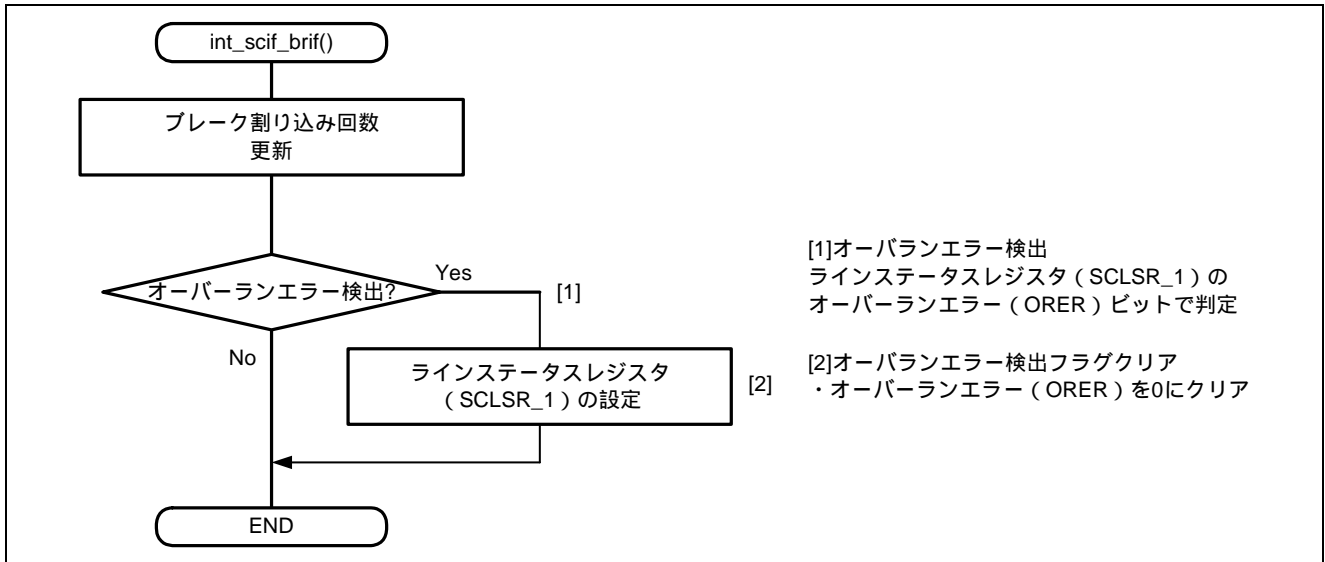
図9 SCIF ブレーク割り込み関数（オーバーランエラー処理）の処理フロー
