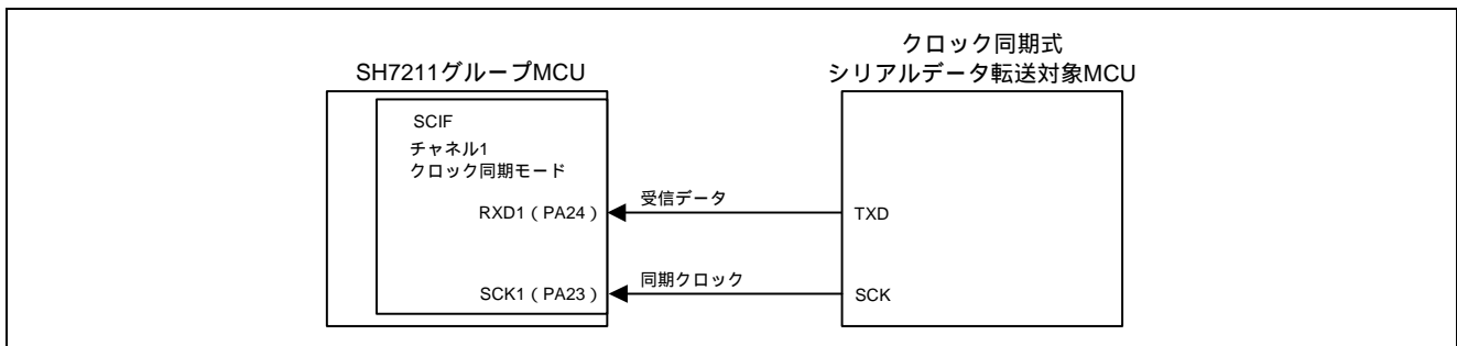
図 1 FIFO 付きクロック同期式シリアルデータ受信動作
