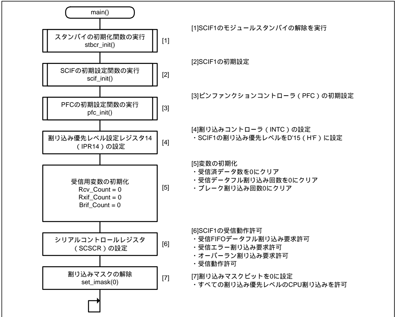
図 4 メイン関数の処理フロー
