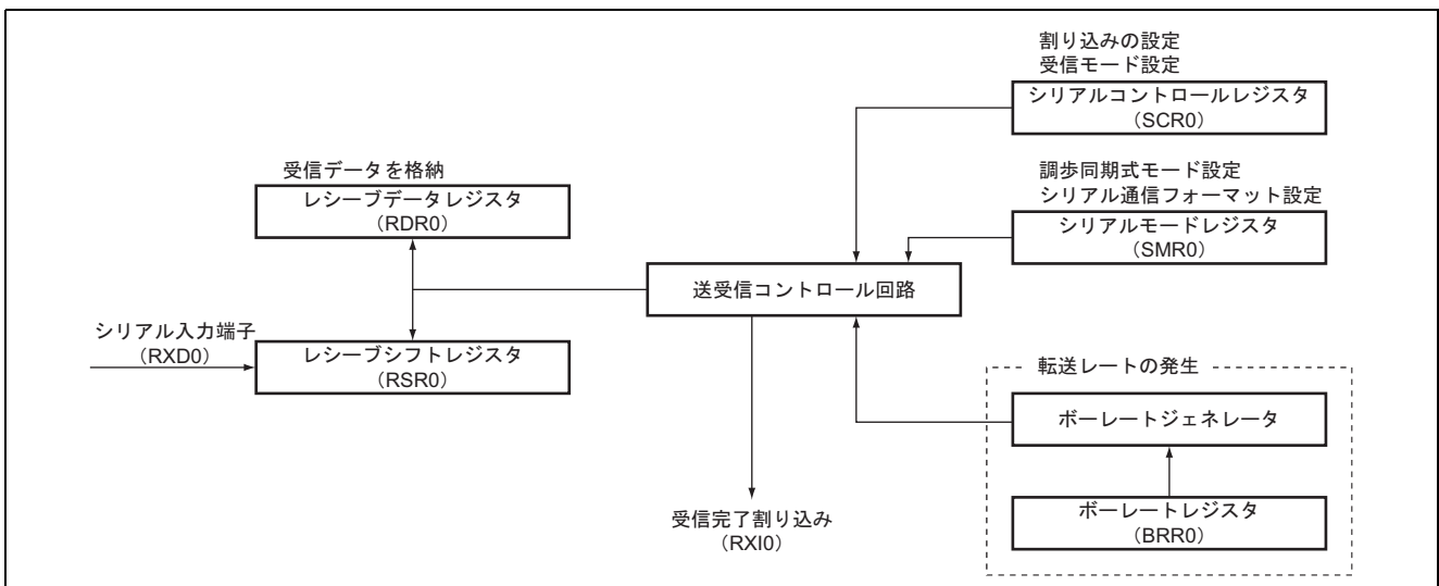
図 3 SCI 受信ブロック図
