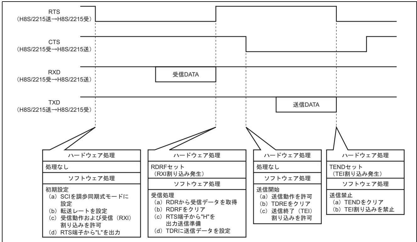
図 4 調歩同期式 SCI 動作原理
