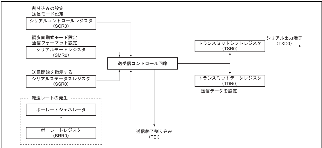
図 2 SCI 送信ブロック図
