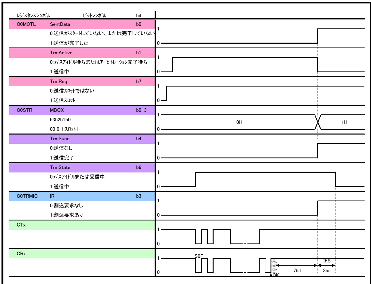
図1 CAN 送信時の各フラグの動作タイミング
