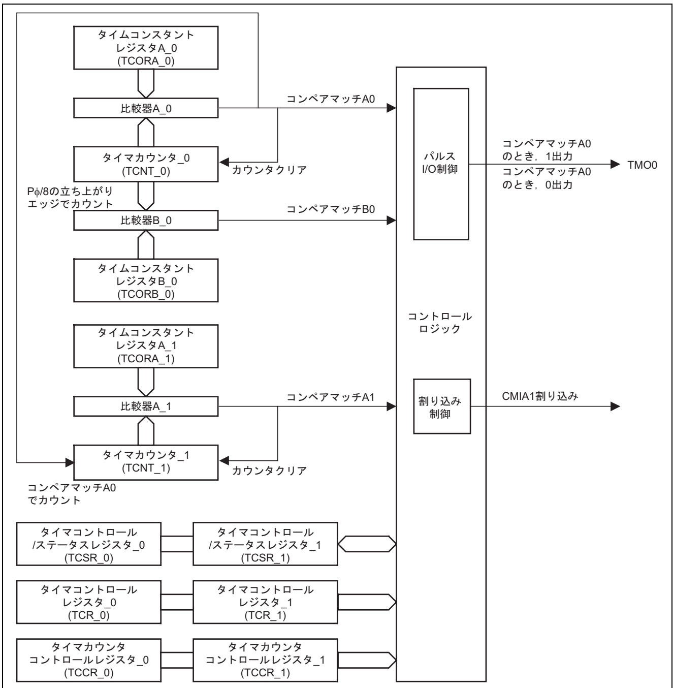
図2 8ビットタイマのブロック図
