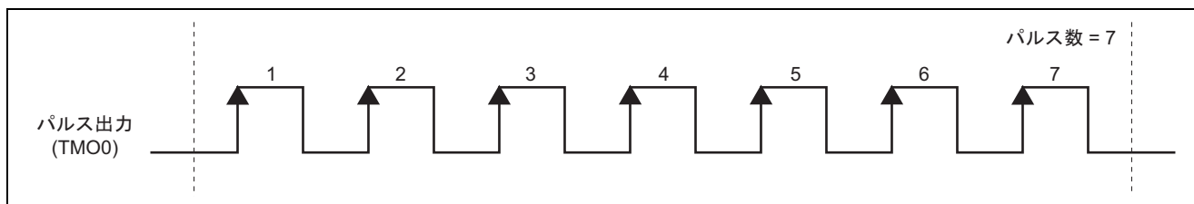
図 1 パルス出力タイミング例
