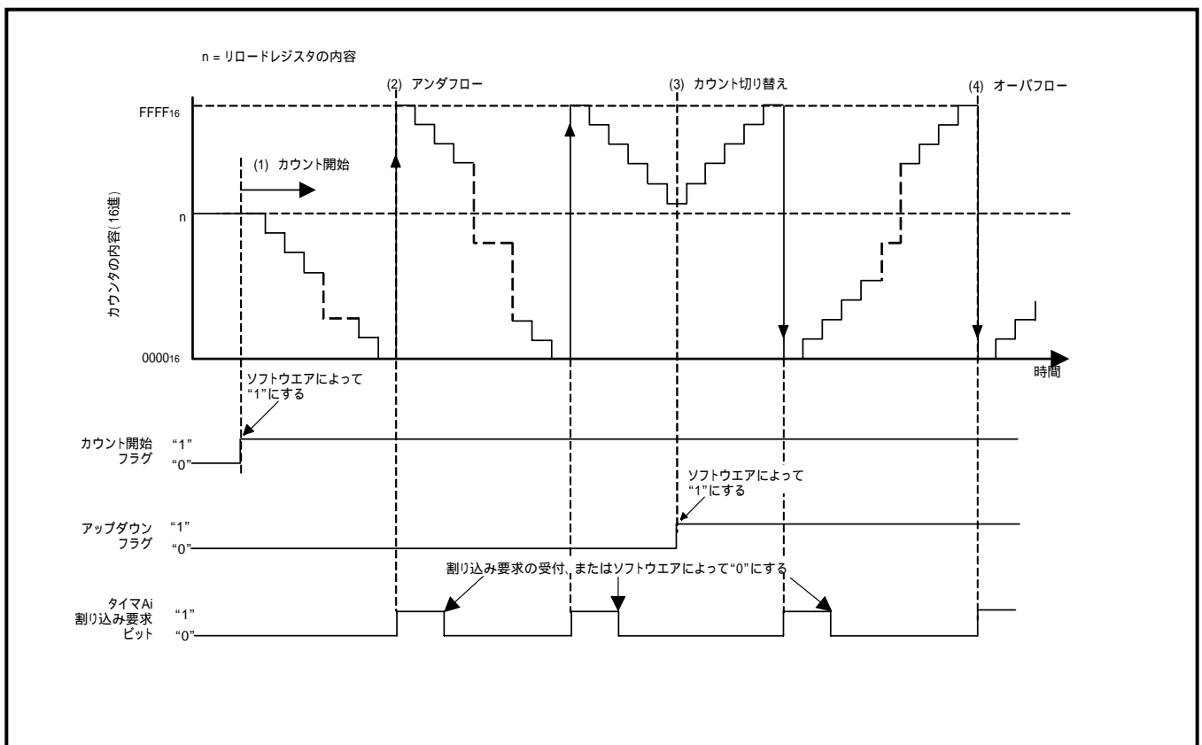
図 1. イベントカウンタモード、フリーランタイプ選択時の動作タイミング図
