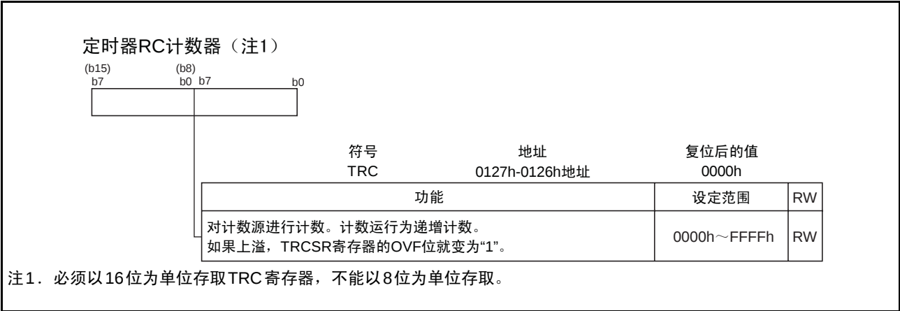
图6 TRC寄存器
