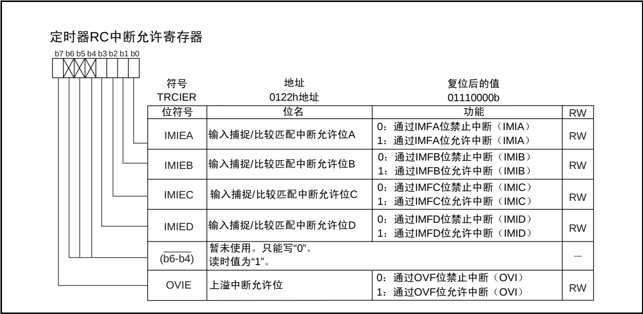
图4 TRCIER 寄存器
