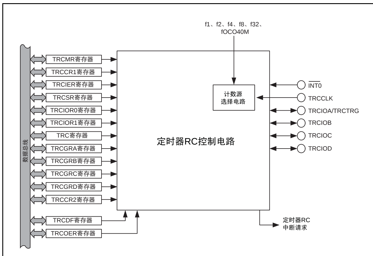
图1 定时器 RC 的框图
