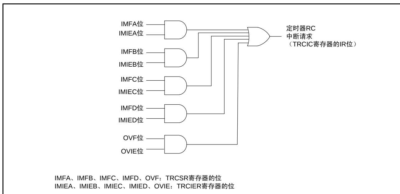
图 19 定时器 RC 中断的框图
