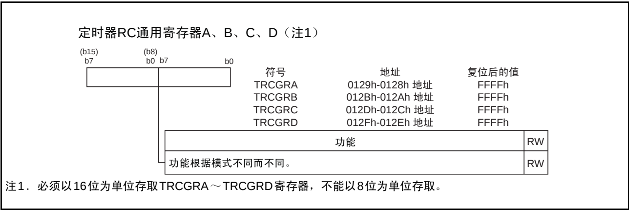
图7 TRCGRA、TRCGRB、TRCGRC、TRCGRD寄存器
