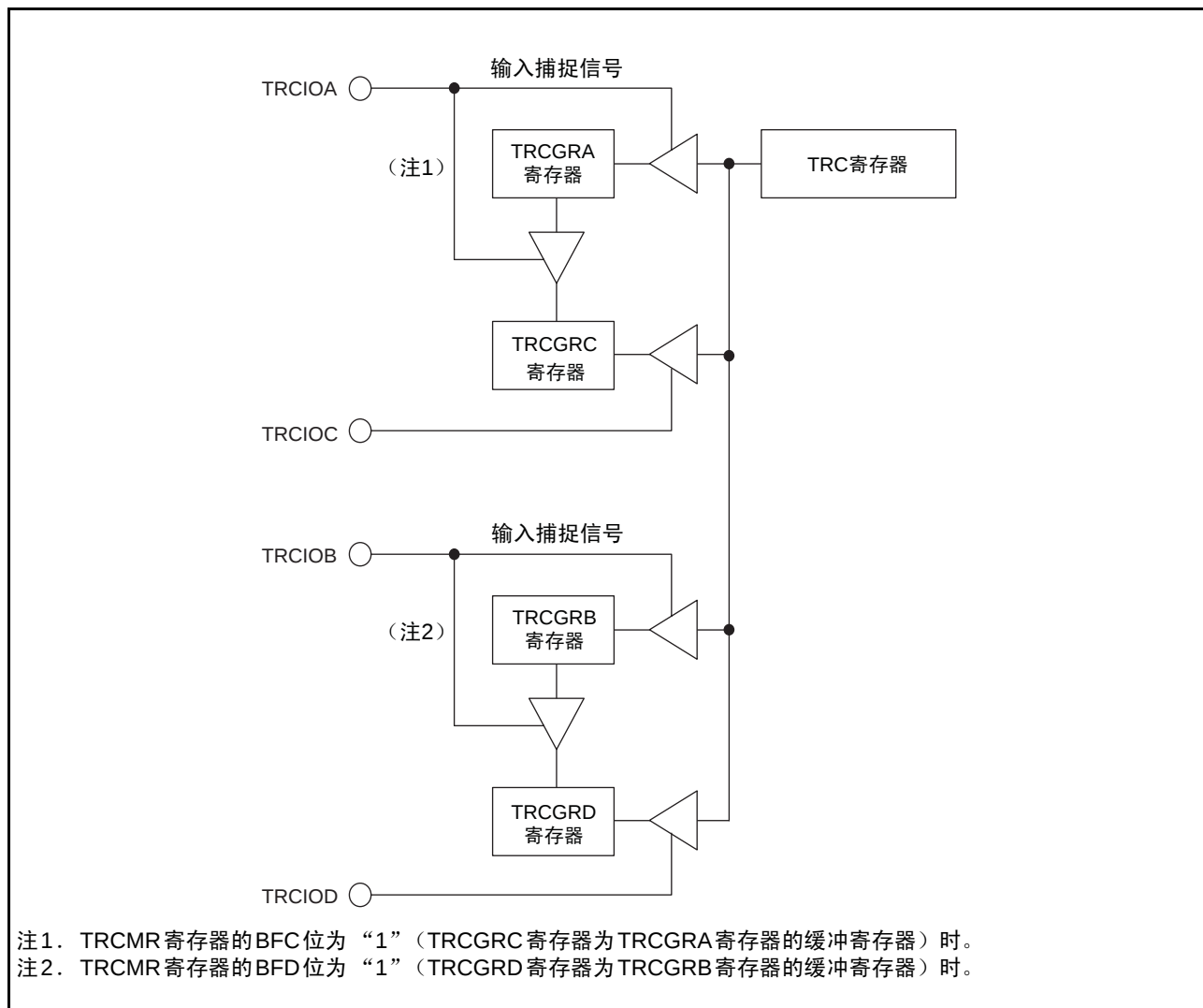
图15 输入捕捉功能的框图
