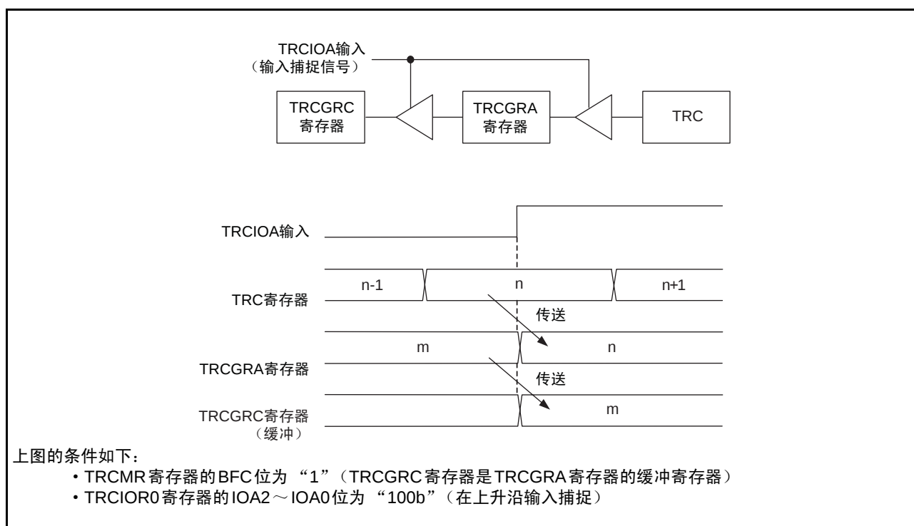
图13 输入捕捉功能的缓冲器运行
