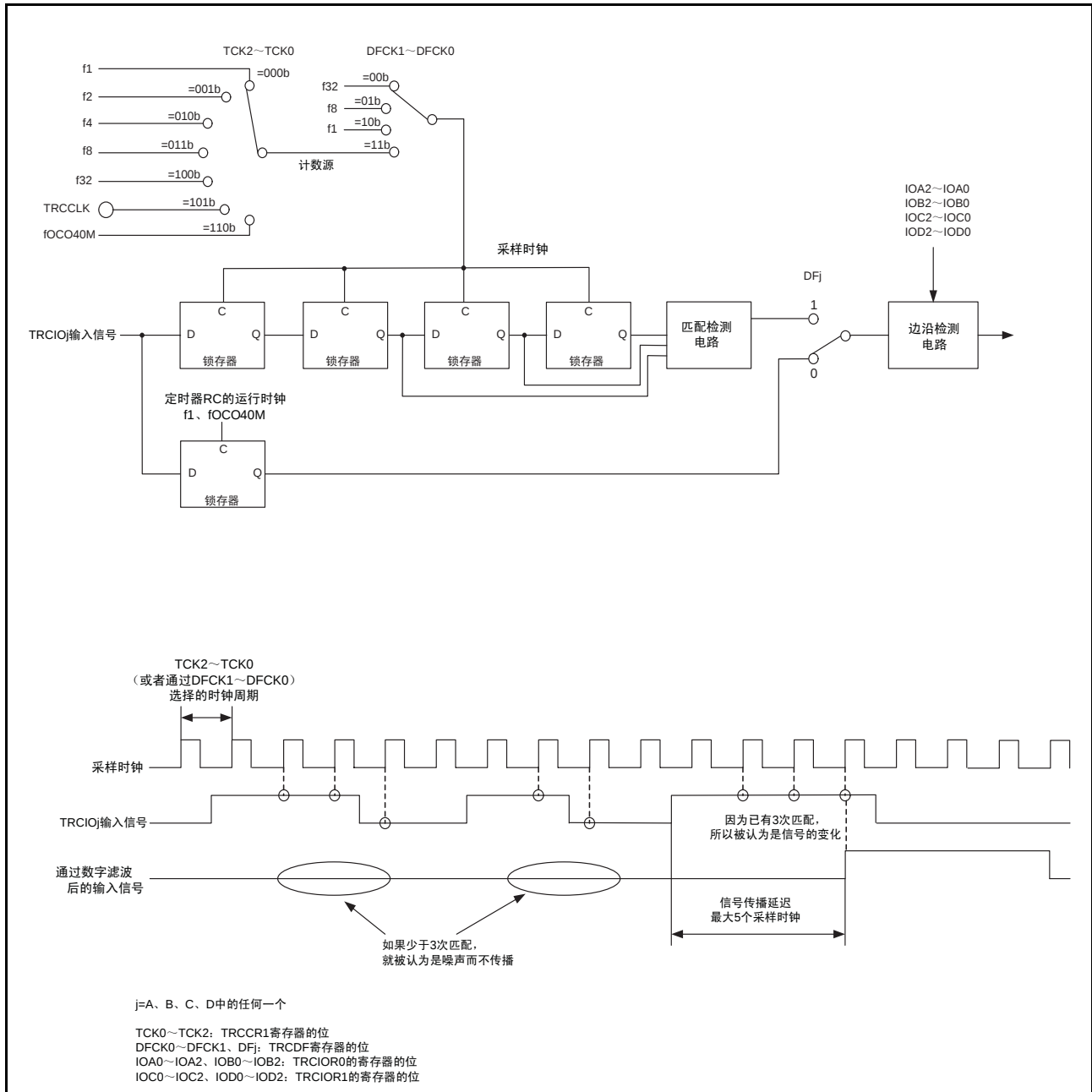
图14 数字滤波器的框图
