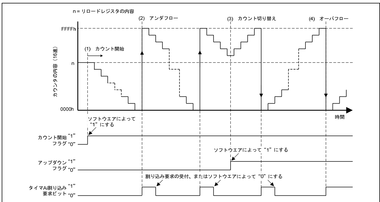
図 1. イベントカウンタモード、フリーランタイプ選択時の動作タイミング
