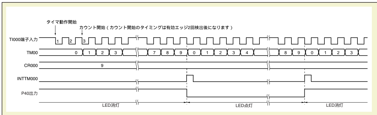
図4 - 5 外部イベント・カウンタ動作のタイミング・チャート例 (本サンプル・プログラム・ソースの場合)
