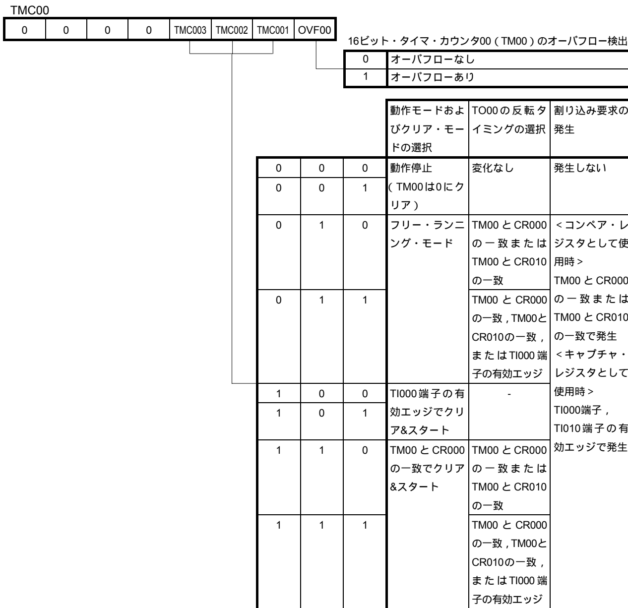
図4 - 4 16ビット・タイマ・モード・コントロール・レジスタ00 (TMC00) のフォーマット
