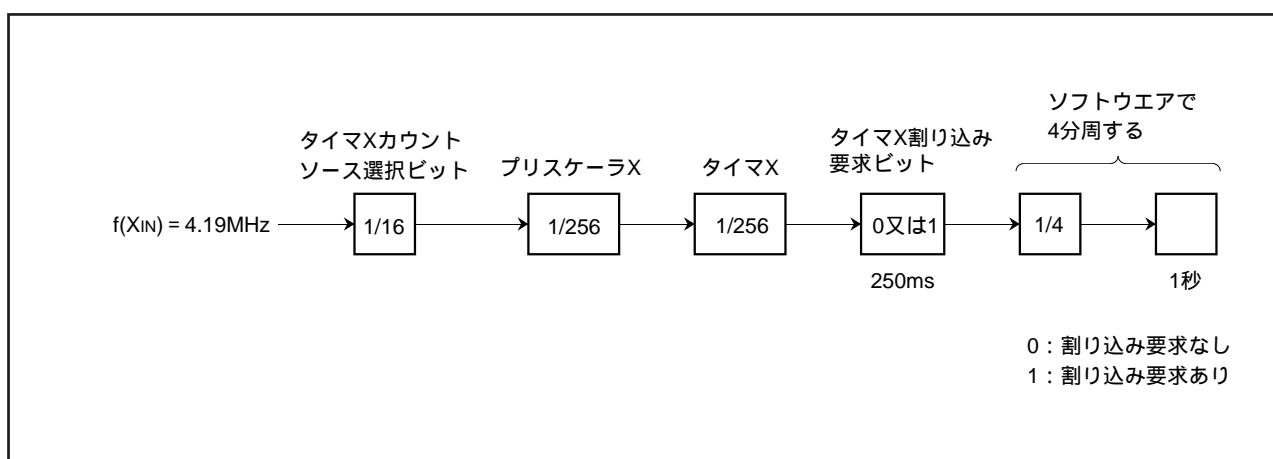
図1. タイマの接続と分周比の設定
