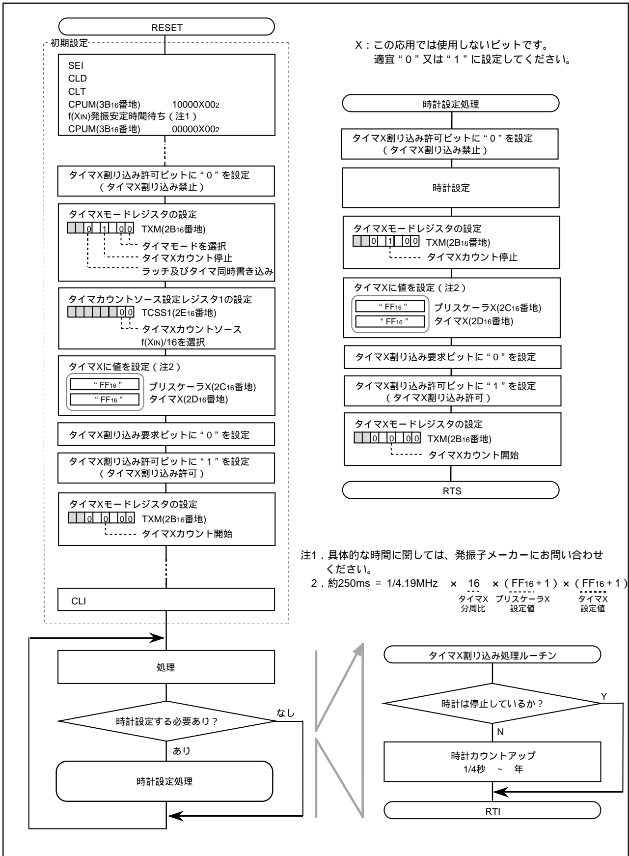
図2. 制御手順例
