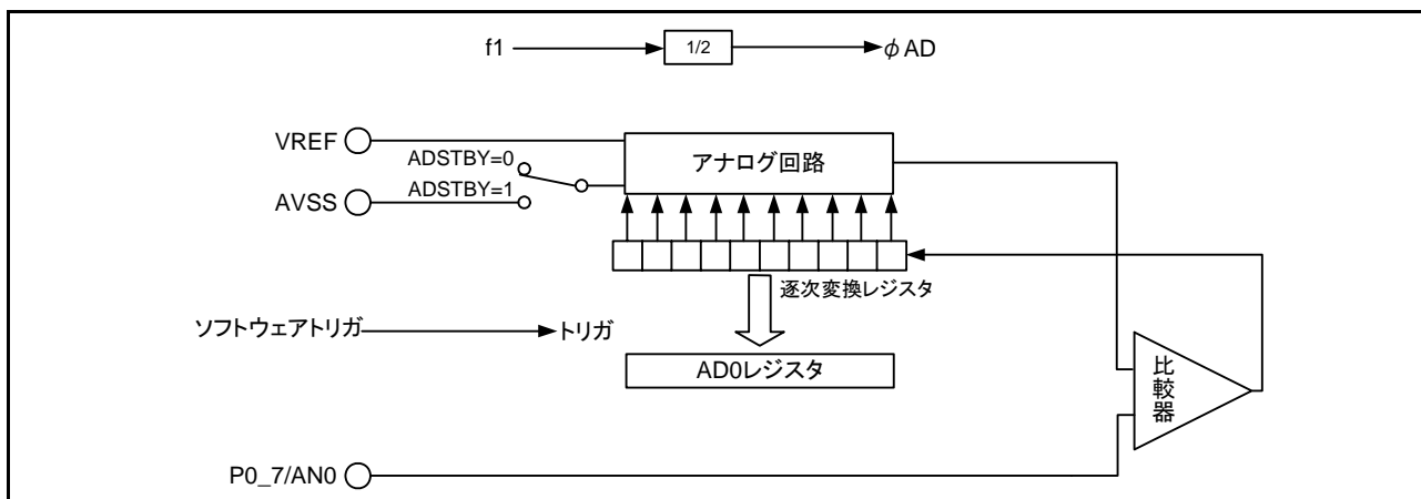
図 3.1 ブロック図
