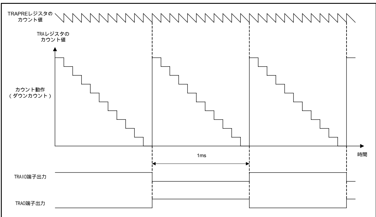
図 3.2 タイミング図
