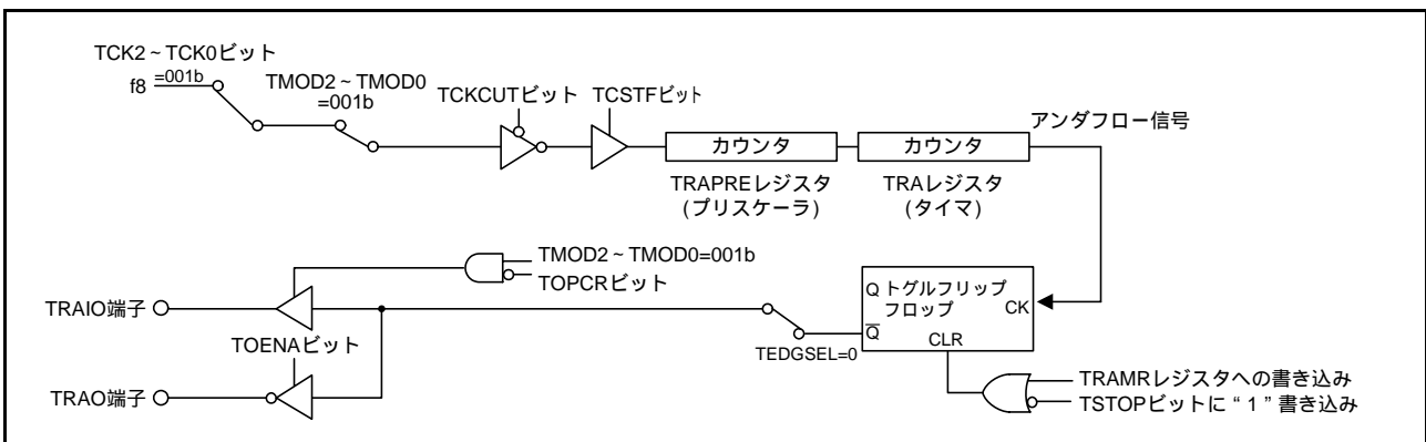
図 3.1 ブロック図
