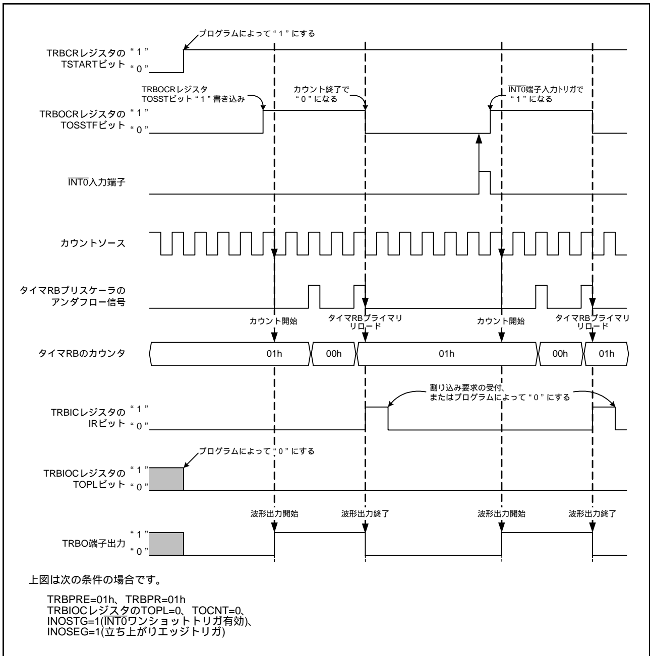
図 3.5 プログラマブルワンショット発生モード時の動作例
