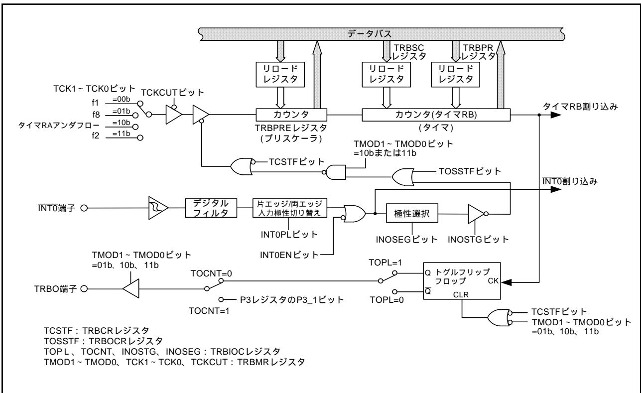
図 3.1 タイマRBのブロック図
