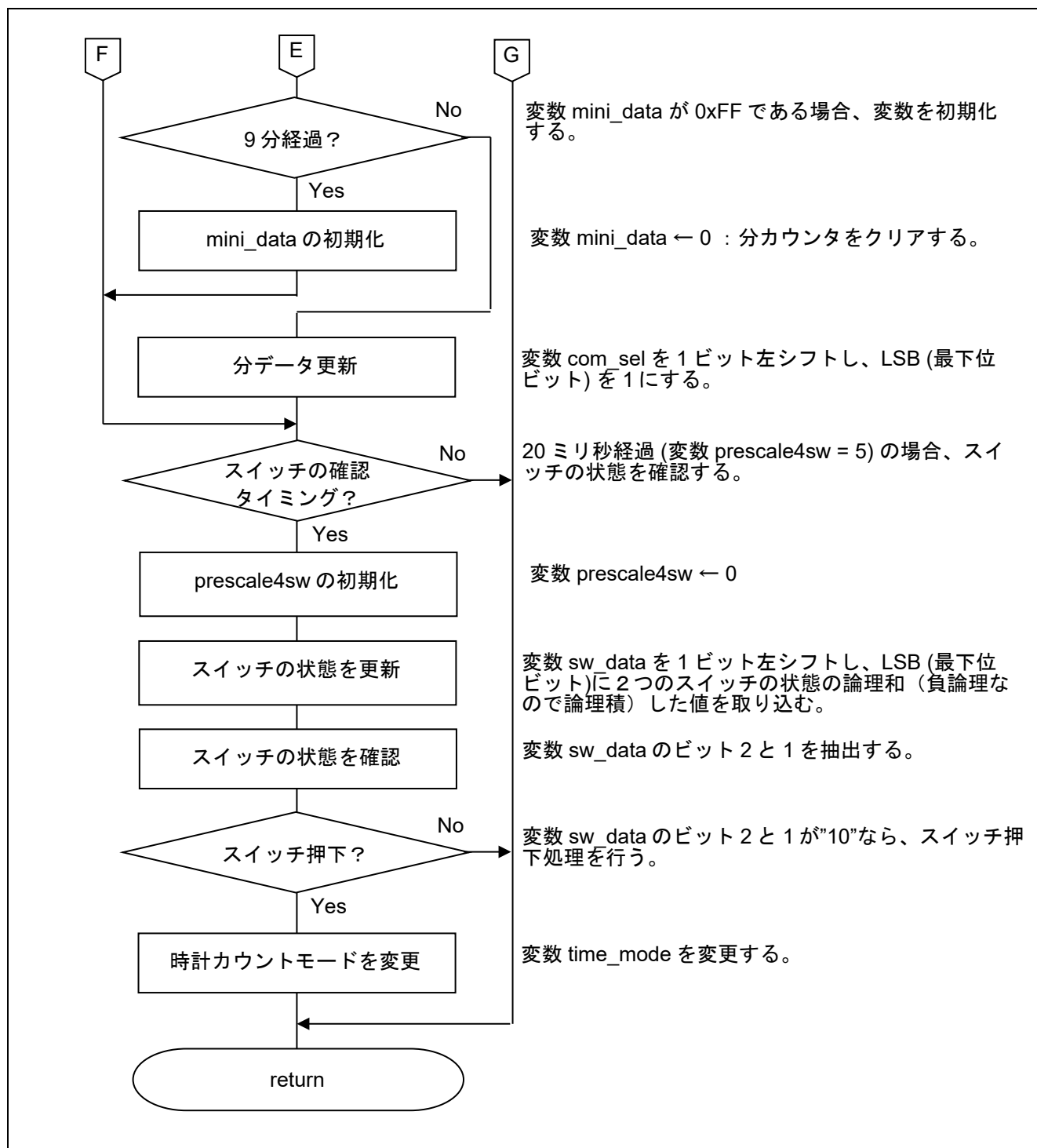
図 5.6 メイン関数 (4/4)
