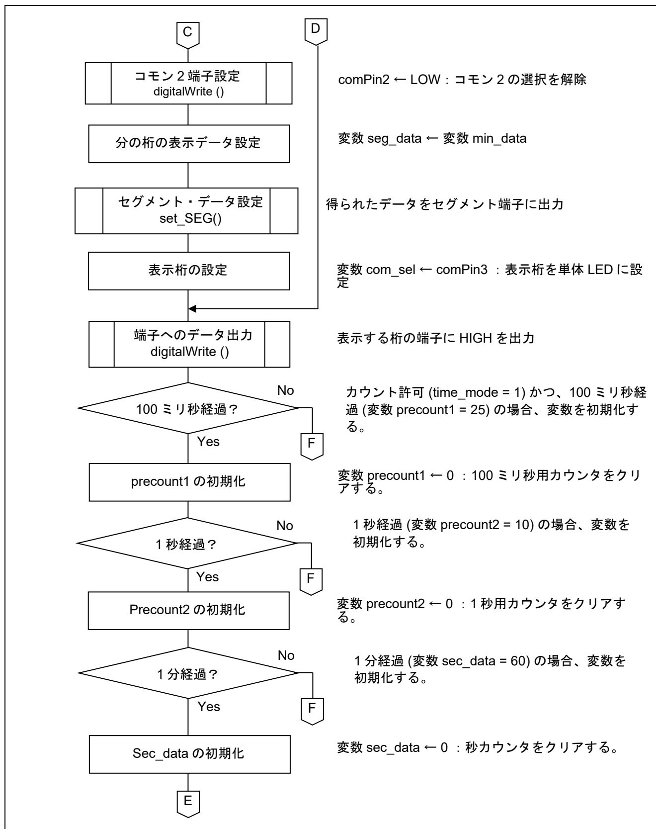
図 5.5 メイン関数 (3/4)
