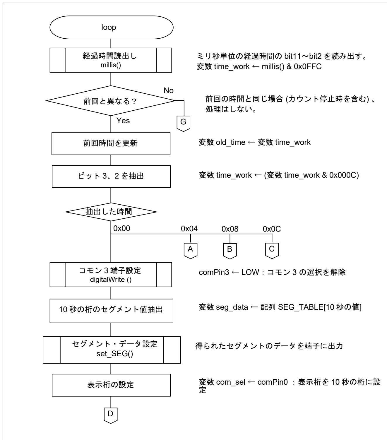
図 5.3 メイン関数 (1/4)
