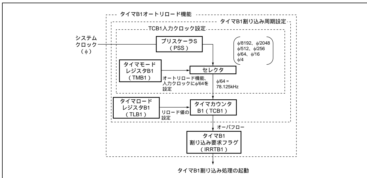
図 2.1 タイマ B1 オートリロード機能ブロック図
