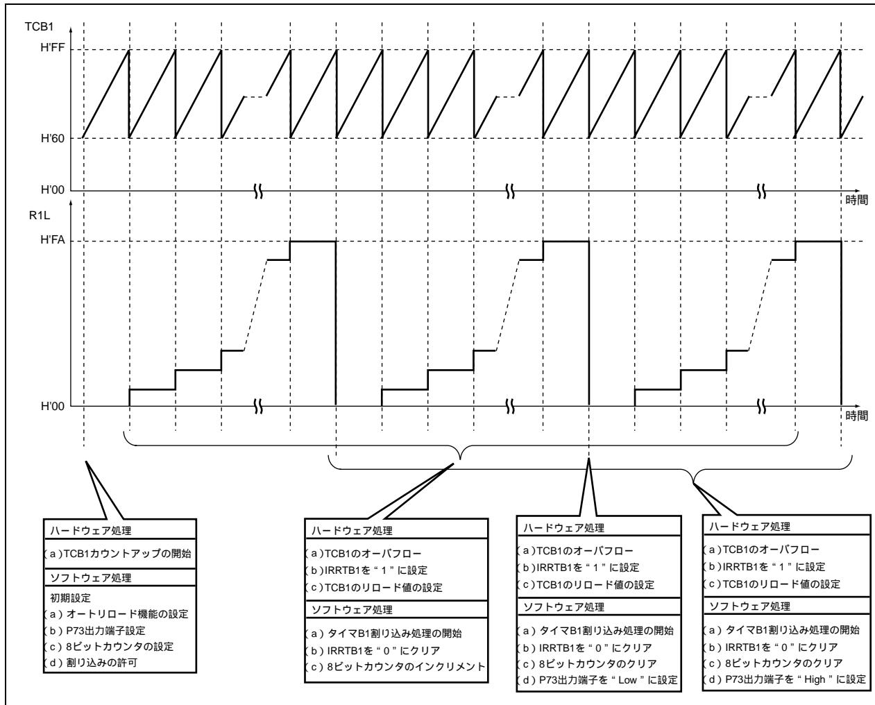
図 3.1 タイマ B1 オートリロード機能による割り込み周期設定の動作原理
