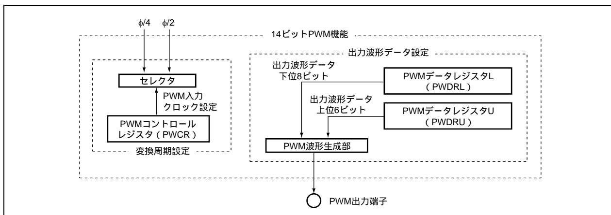
図 2.1 14ビットPWM機能ブロック図
