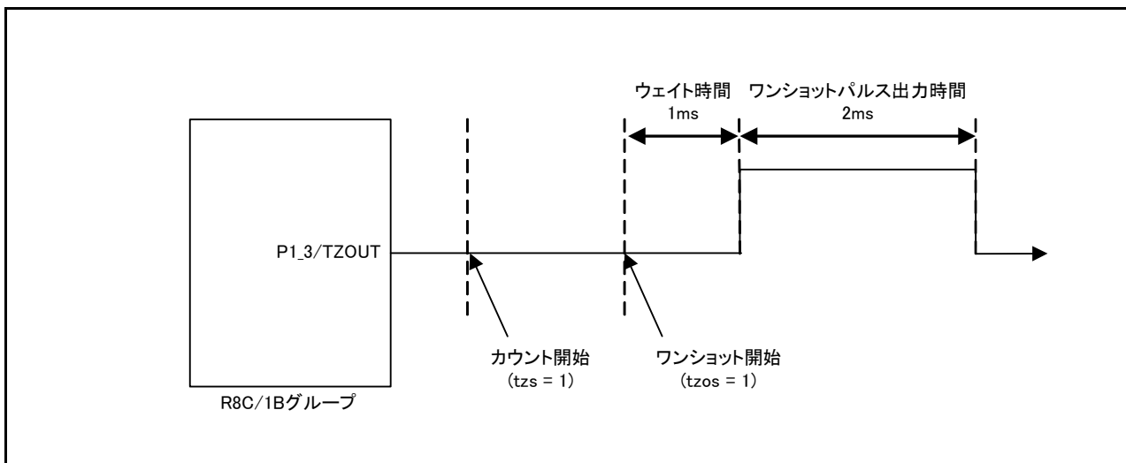
図 5.1 使用端子
