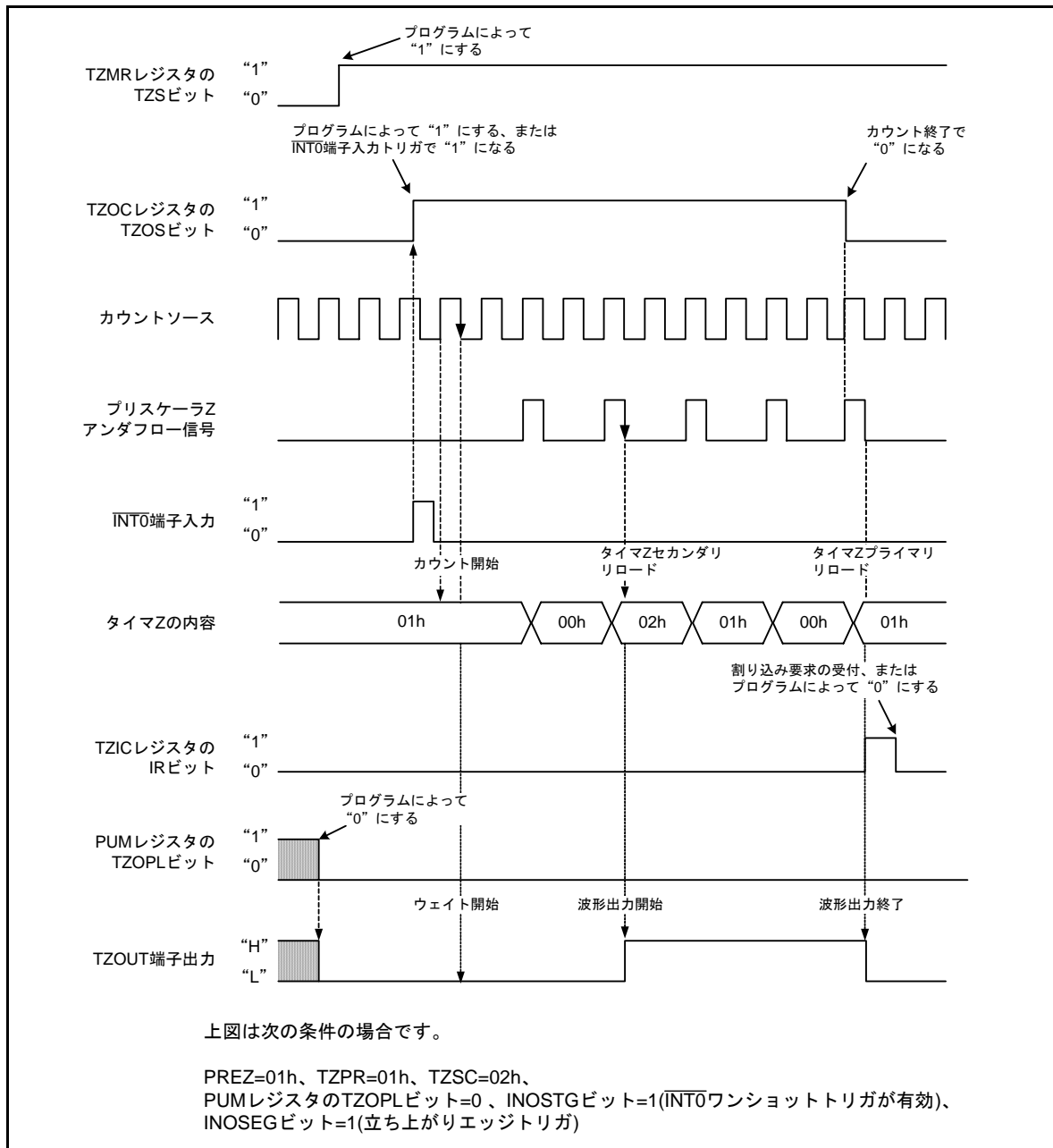
図 3.2 プログラマブルワンショット発生モードの動作例
