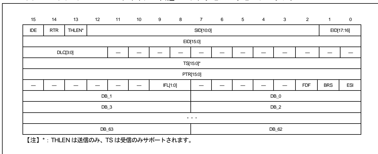
図 3-7 RA6M5 グループのメッセージバッファ構成
